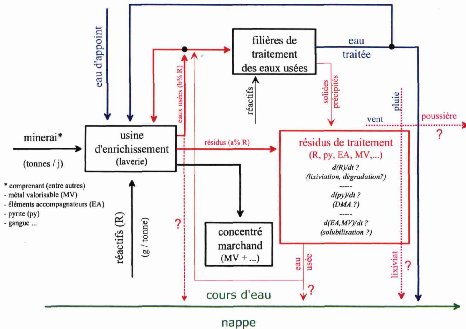
Fig. 13 - Schéma global des processus éventuellement déterminant le flux de réactifs de traitement (et d'autres contaminants originaires du minerai) vers l'environnement.
