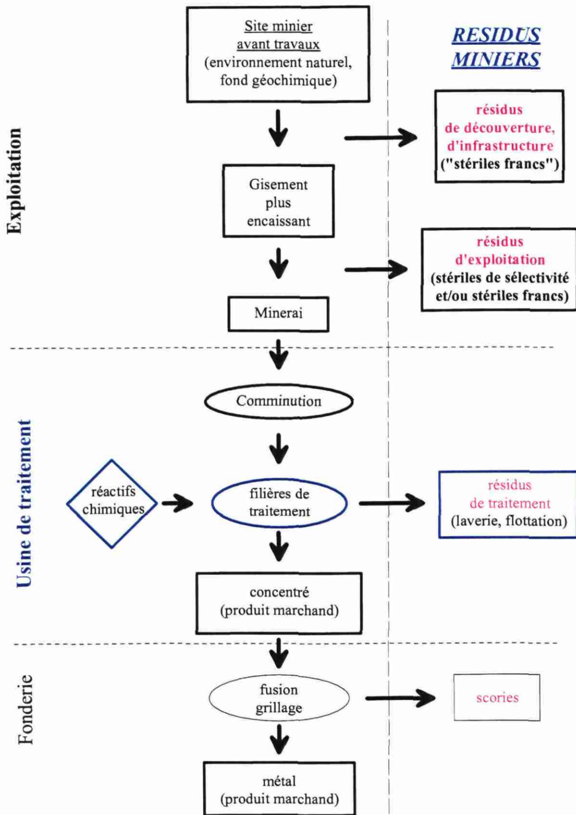
Fig. 2 - Etapes d'exploitation d'un gisement métallique et les résidus miniers correspondants.
