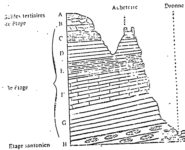
Coupe d'Aubeterre d'après H. COQUAULT (1958)
