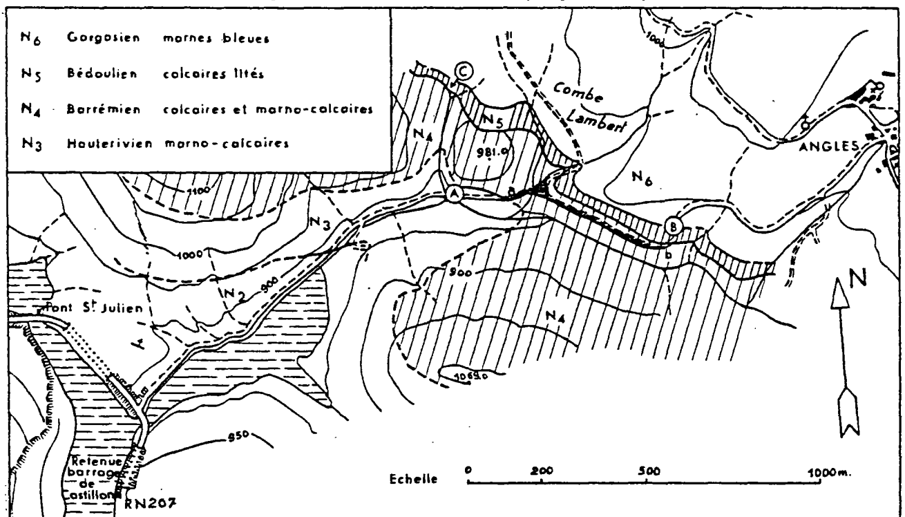
Carte géologique des environs d'Angles.
