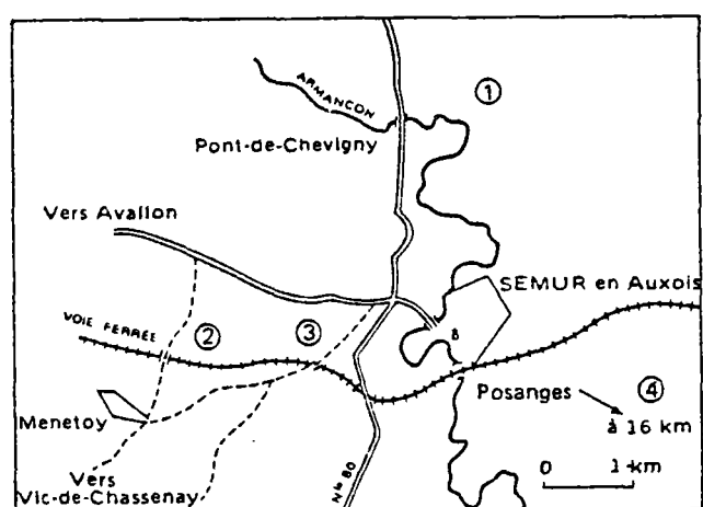
Plan de situation des principaux affleurements du Sinémurien de Semur.
