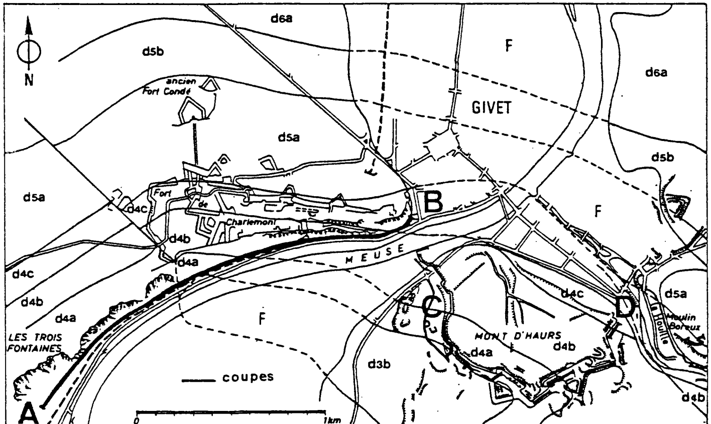
Fig. 3 Carte indiquant les affleurements du Givétien dans la région type, d'après la carte géologique de France à 1/50 000 (feuille de Givet)
