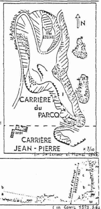
Profil dans la partie méridionale de la Carrière du Parc à Etroeuingt.
