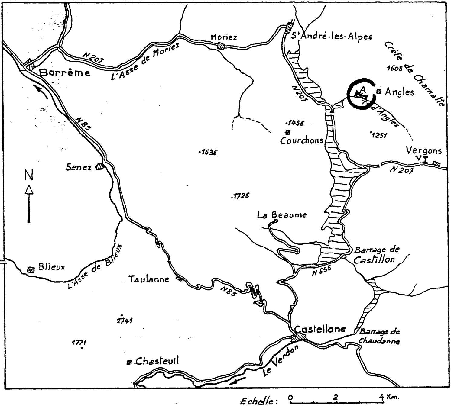
Carte de la région de Barrême , Angles et Castellane (Alpes de Haute Provence). A : situation de la coupe d'Angles, stratotype du Barrémien.
