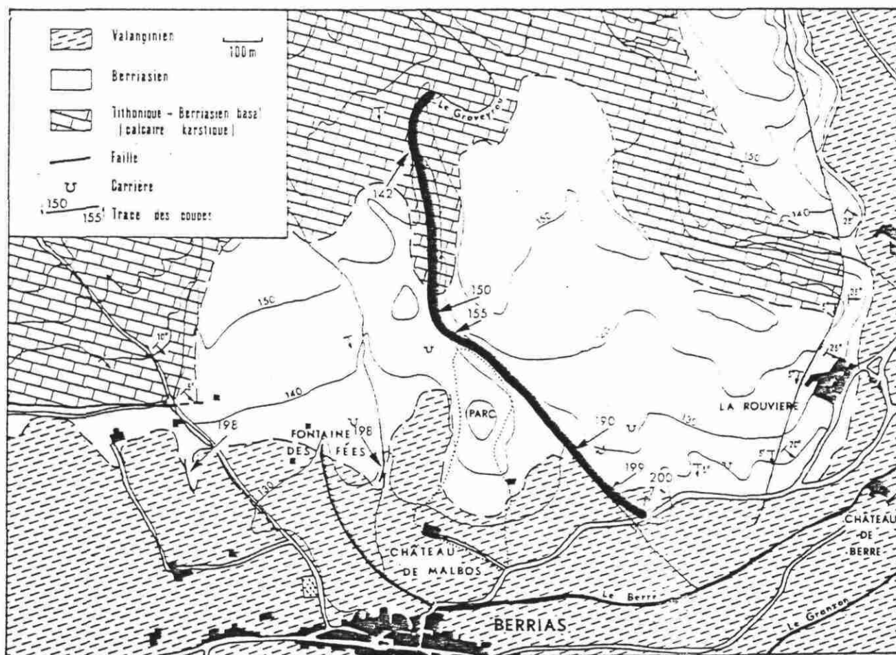
Cheminement de la coupe de Berrias (d'après G. LE HEGARAT, 1965)
