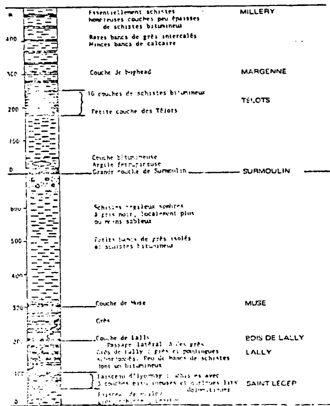
Coupe verticale de l'Autunien.
