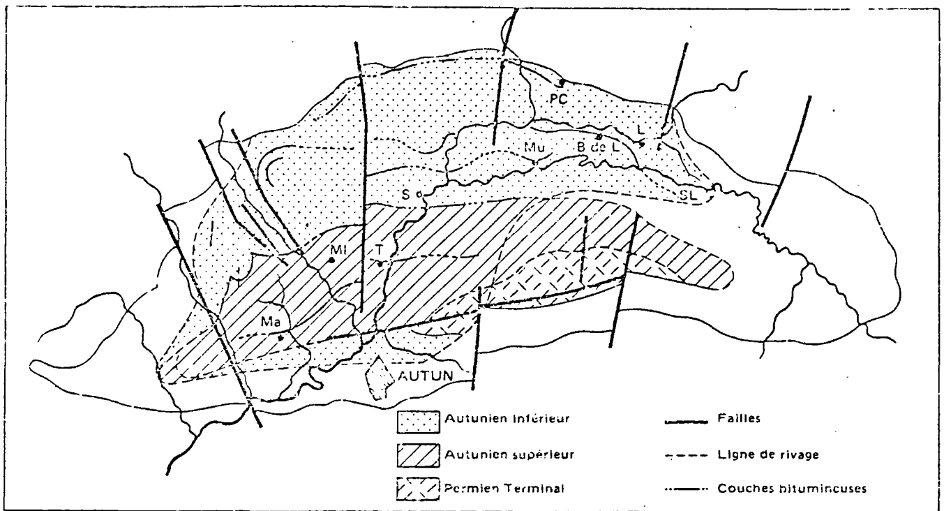
Carte géologique et tectonique du bassin d'Autun. Mi = Miliery, Ma = Margenne, T = Telots, S = Surmoulin, Mu = Muse, L = Lally, B de L = Bois de Lally, SL = St Leger du Bois, PC = Petit Chaume.
