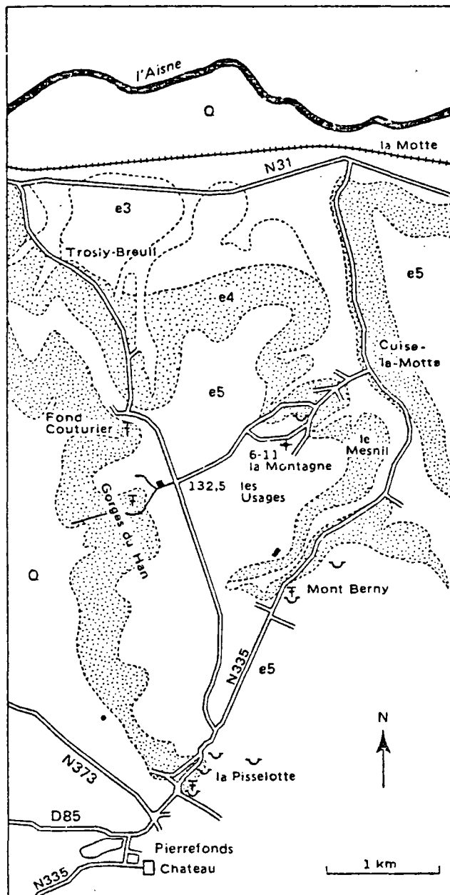
CUISIEN - STRATOTYPE
