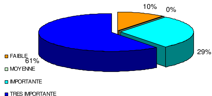
Illustration 25 – Tableaux et graphique de répartition des notes de potentialités des nappes alluviales du Gers
