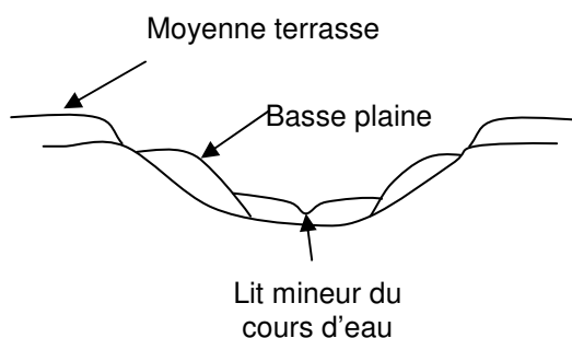
Illustration 17 – Schéma de principe de géométrie des terrasses alluviales
