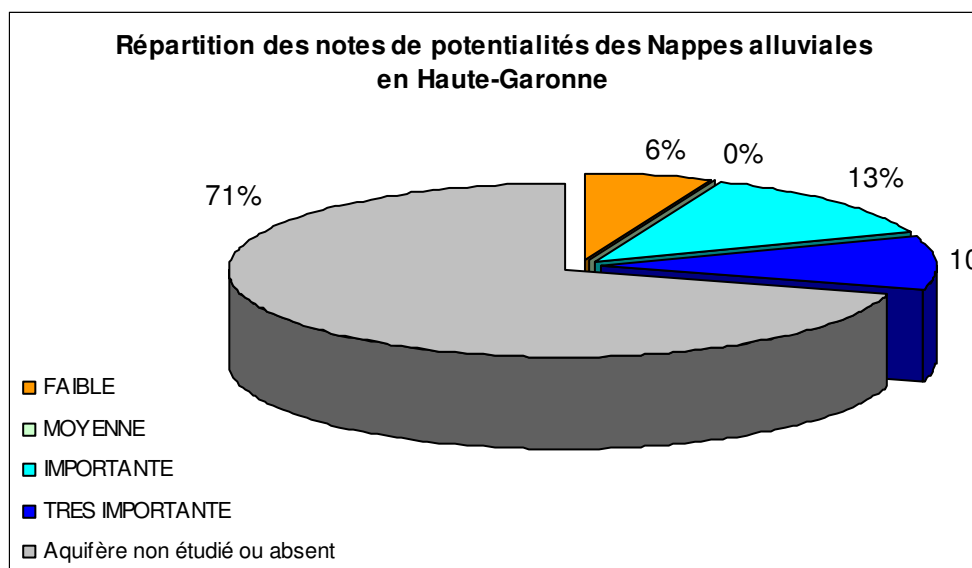
Illustration 29 – Tableaux et graphique de répartition des notes de potentialités des nappes alluviales de la Haute-Garonne
