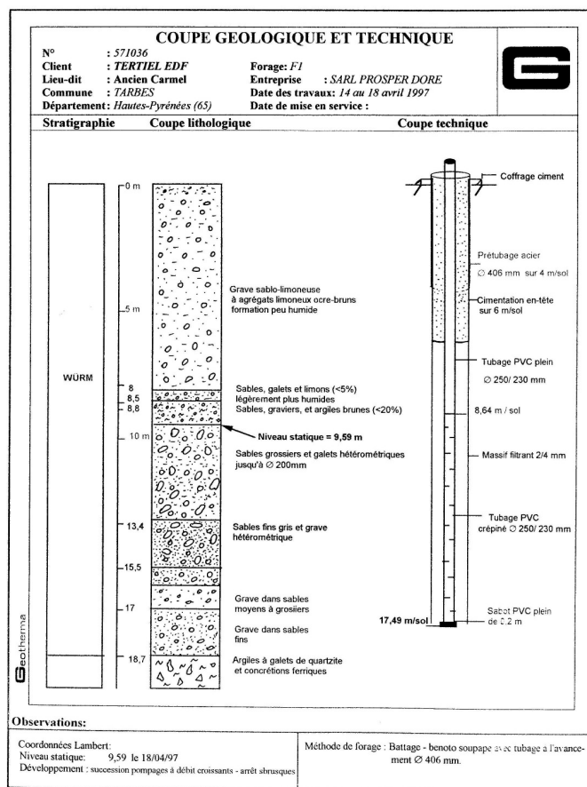
Figure 3 : Coupe lithologique et technique du forage F1.
