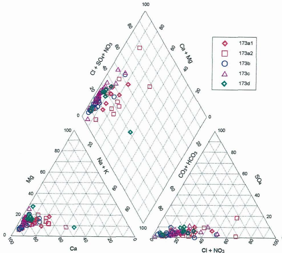
Figure 5 : Diagramme de Piper des eaux des Cailloutis du Sundgau (173a1 : Belfortain alpin ; 173a2 : Belfortain vosgien ; 173b : Est Largue ; 173c : Thalbach ; 173d : Largue/Doller)
