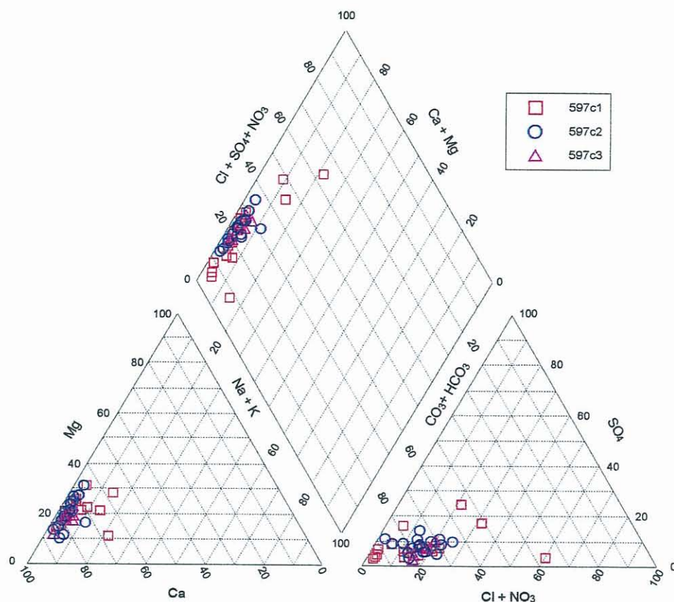
Figure 4 : Diagramme de Piper des eaux de l'Oligocène du Sundgau
