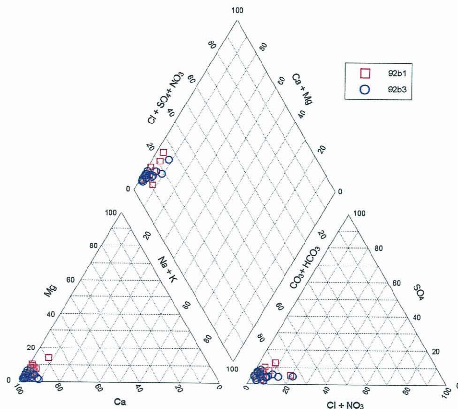
Figure 3 : Diagramme de Piper des eaux du Jura alsacien (92b1 : Grande oolithe, 92b3 : Jurassique supérieur)
