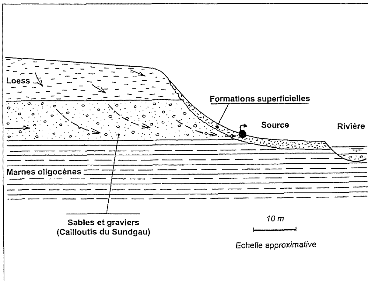
Figure 2 : Schéma de fonctionnement des circulations d'eau dans les Cailloutis du Sundgau
