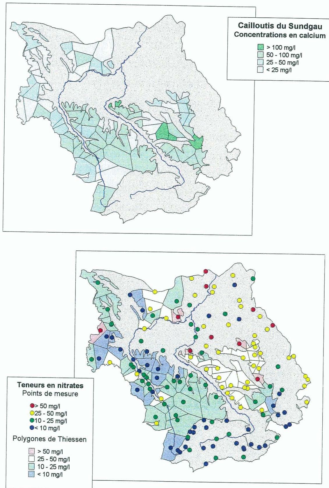
Figure 6 : Représentations par polygones de Thiessen des teneurs en calcium et en nitrates des Cailloutis du Sundgau
