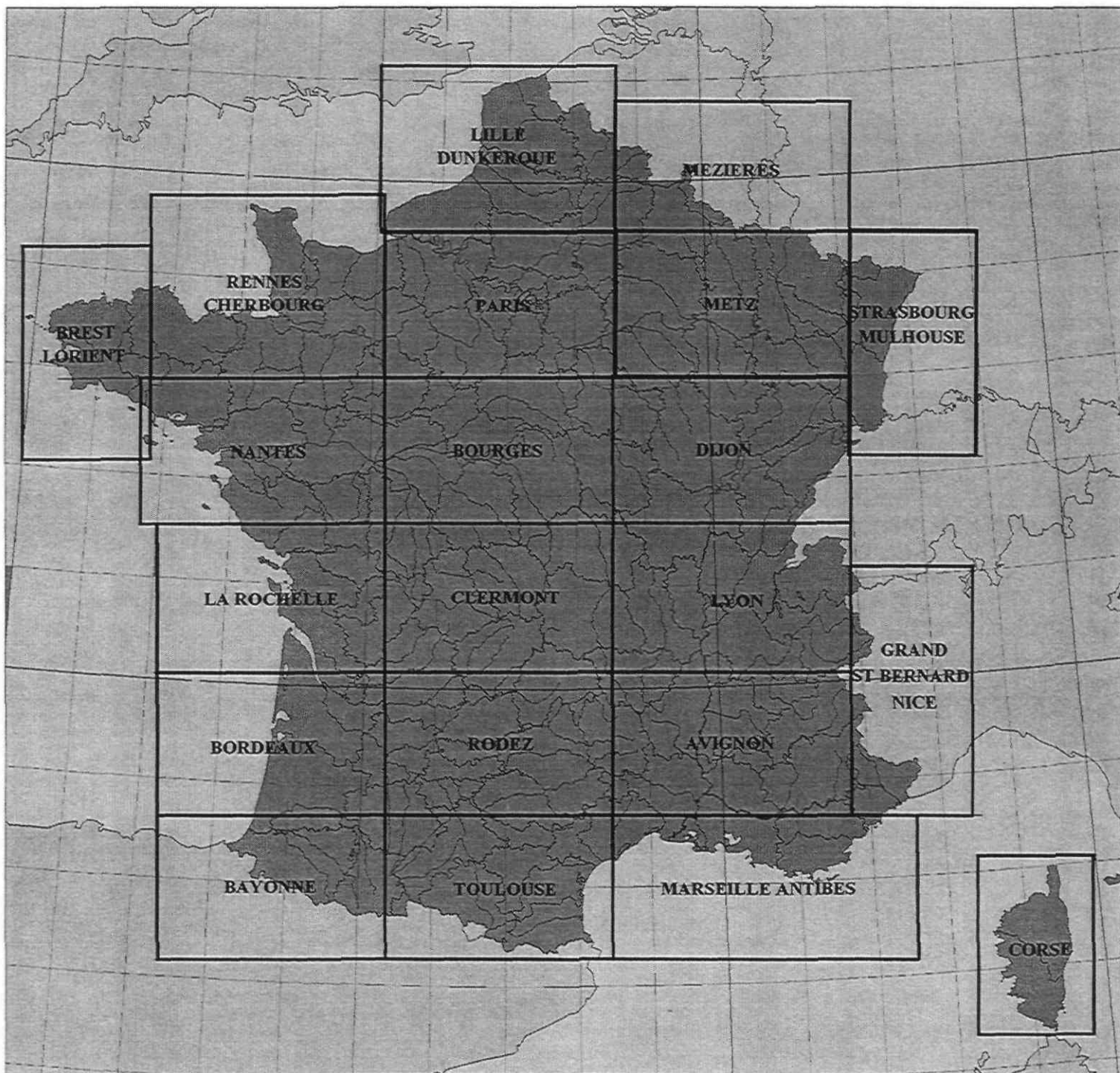
CARTE GEOLOGIQUE DE LA FRANCE A 1/320.000
