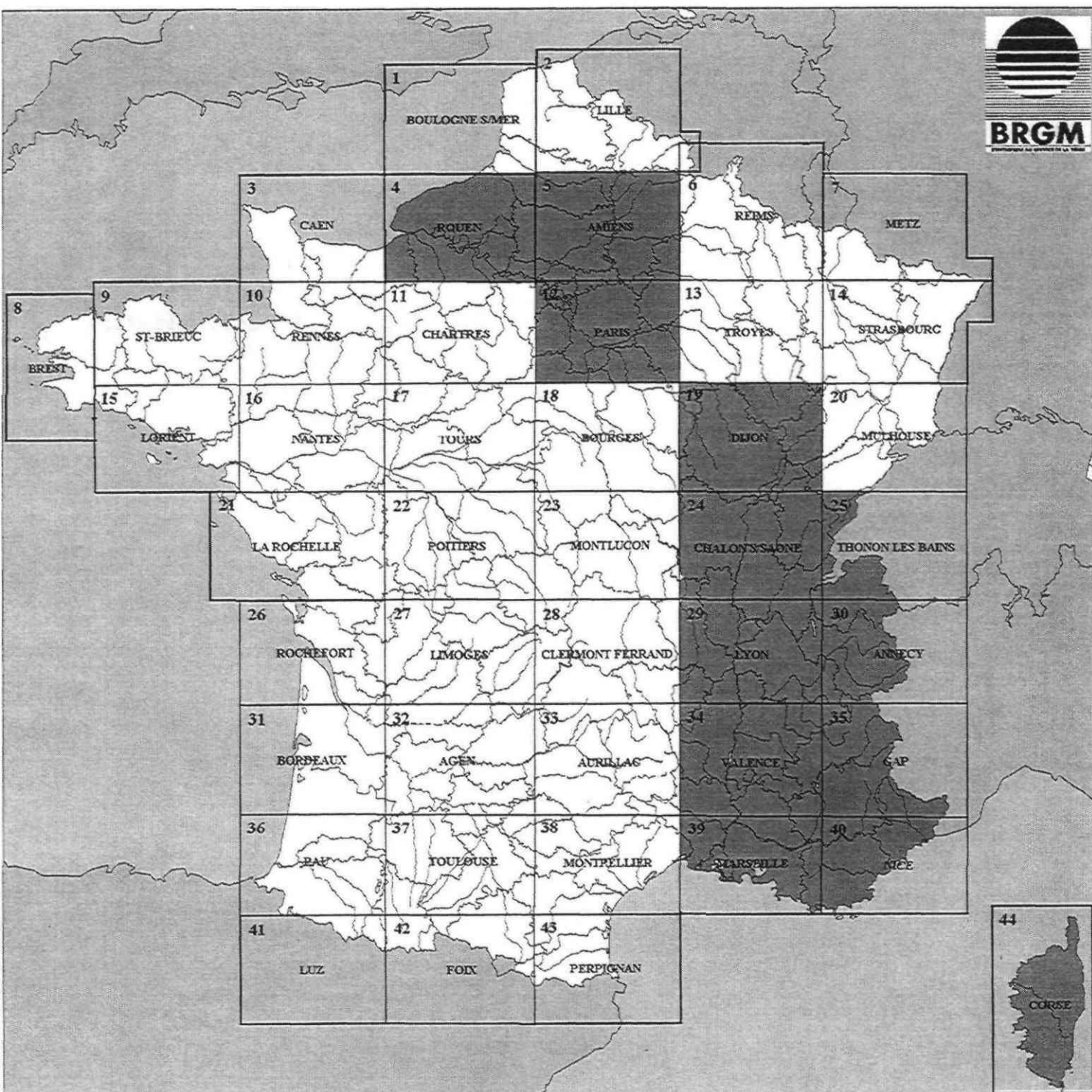
CARTE GEOLOGIQUE DE LA FRANCE A 1/250.000
