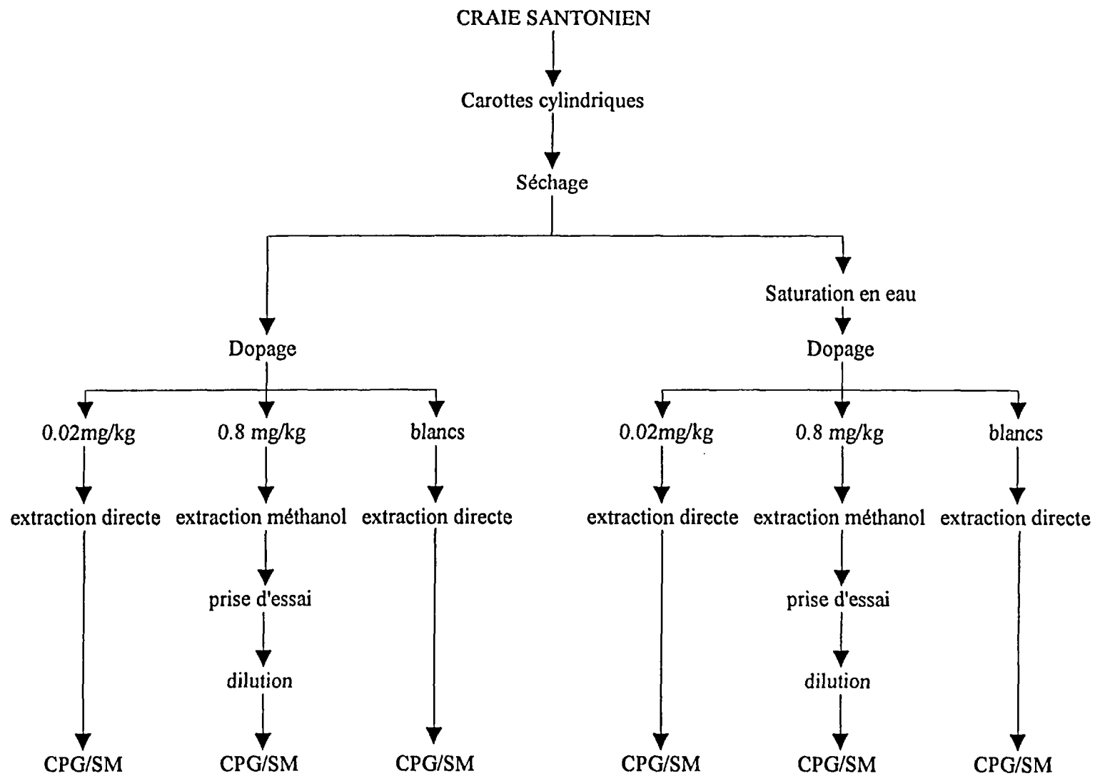
Fig. 1 - Méthodologie d'extraction de composés organohalogénés utilisée lors des tests sur échantillons de craie du Santonien.
