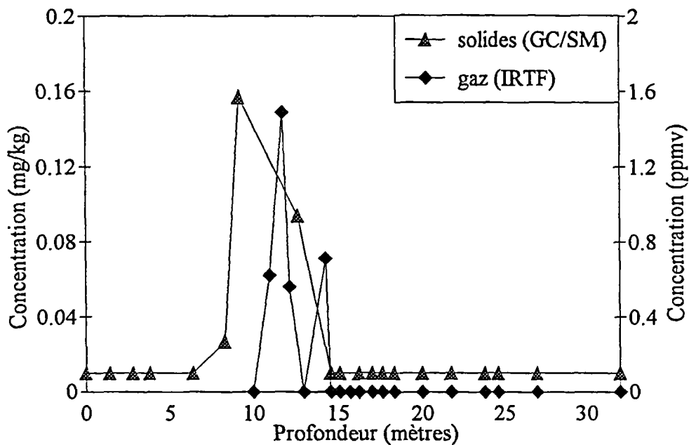
Fig. 7 - Comparaison des teneurs en 1, 1, 1 TCA obtenues par extraction sur les solides et par mesure IRTF des gaz des fluides de forage.
