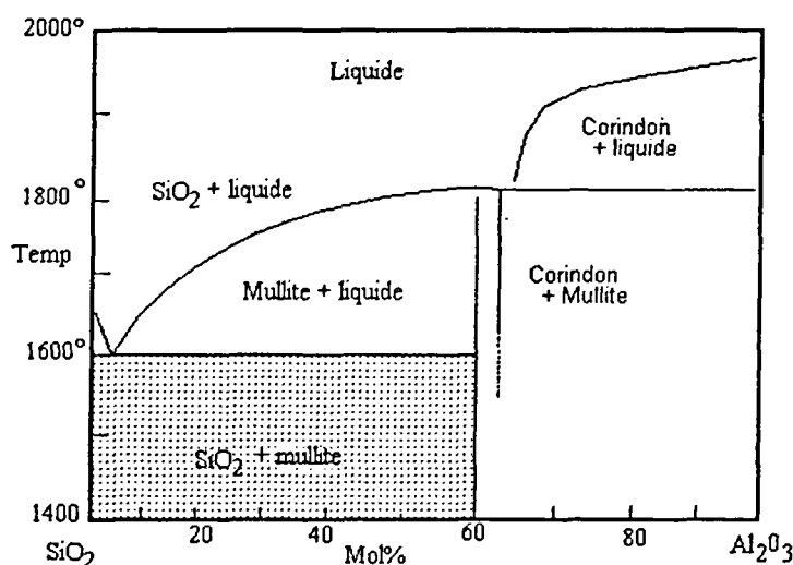
Fig. 14 - Diagramme des phases du système \text{SiO}_2\text{-Al}_2\text{O}_3
