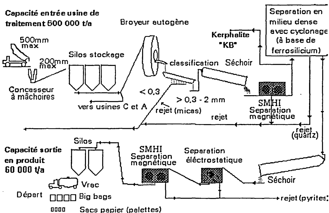
Fig. 4 - Schéma de traitement simplifié de l'usine d'andalousite, Glomel (22).
