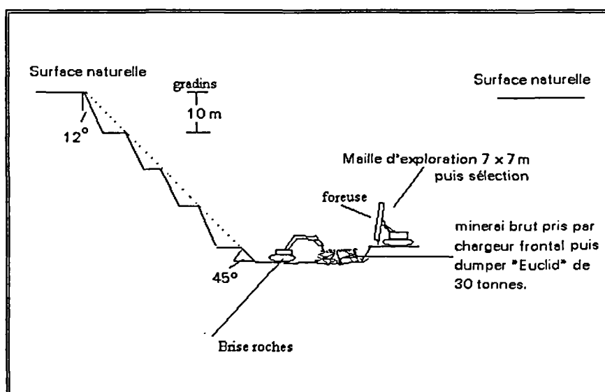
Fig. 2 - Présentation schématique de la carrière d'andalousite de Glomel (22).
