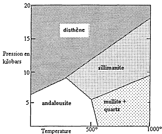
Fig. 5 - Diagramme de phase du système \text{Al}_2\text{SiO}_5 .
