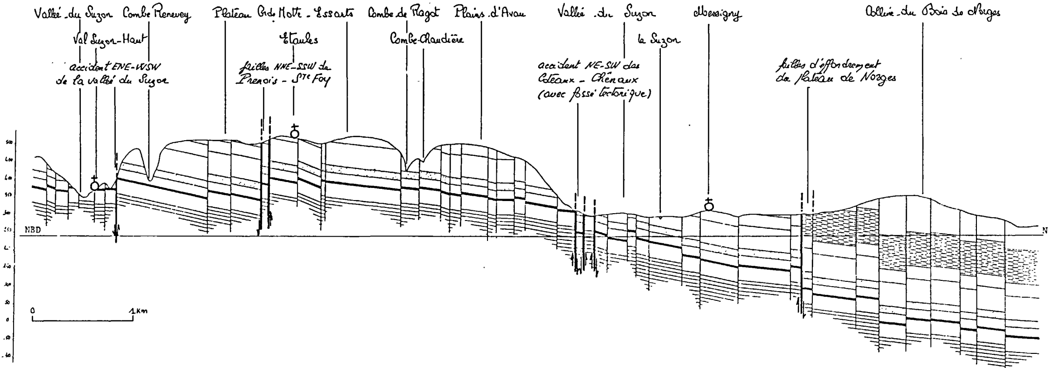
Coupe de Val Suzon à Mbessigny et Morges
