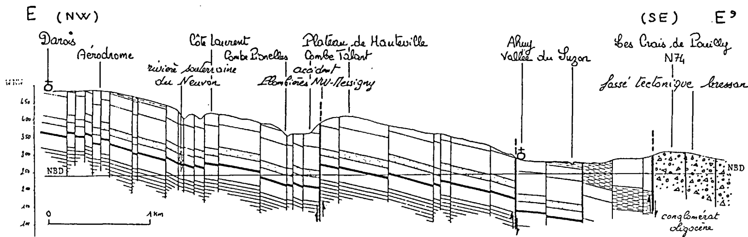
Coupe de Darois a Ahuy et Pouilly
