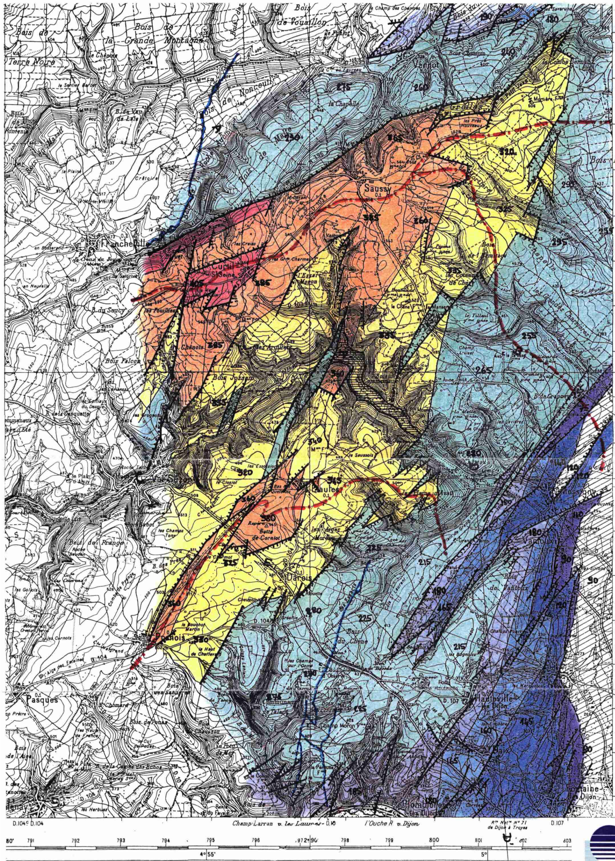
Planche 1.2 - Carte structurale du bassin oriental du Suzon
