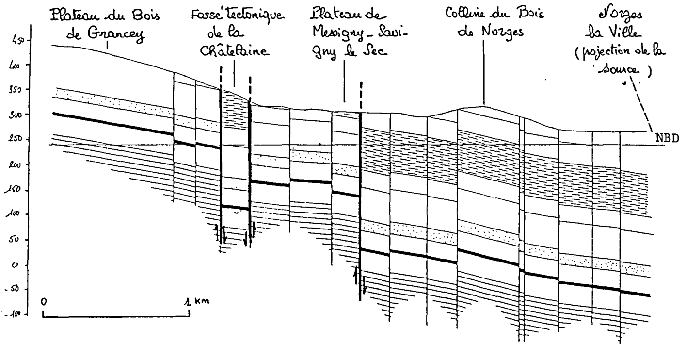
Coupe du plateau nord de Messigny à Norges la Ville
