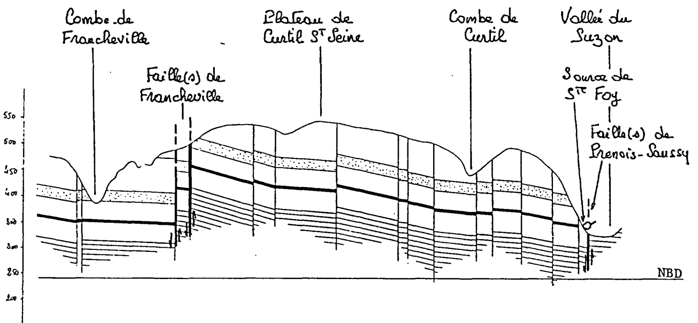
Coupe des plateaux de Francheville au Suzon
