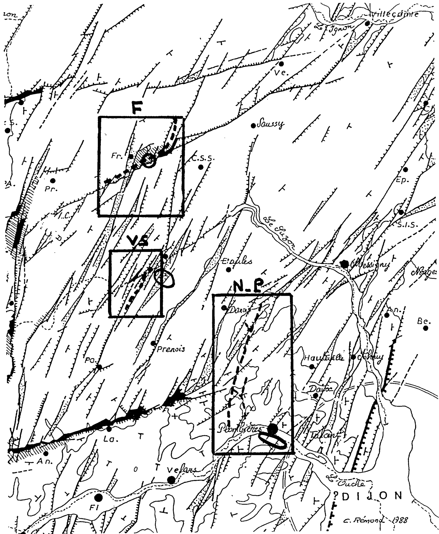
Planche 1.4 c - Fracturation du bassin Sazon-Ouche
