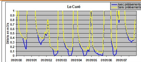
❷ Chroniques de débits simulées « calage » (avec prélèvements) et scénario sans prélèvement
