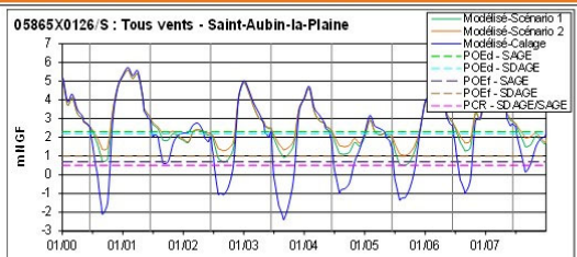
❶ Chroniques piézométriques simulées pour différents scénarios sur les prélèvements
