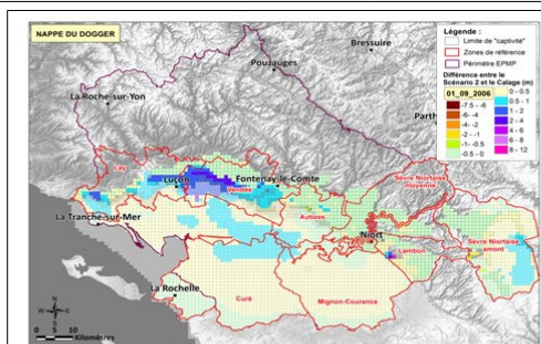
❸ Carte de différence piézométrique : entre 1 scénario de prélèvements et « calage »
