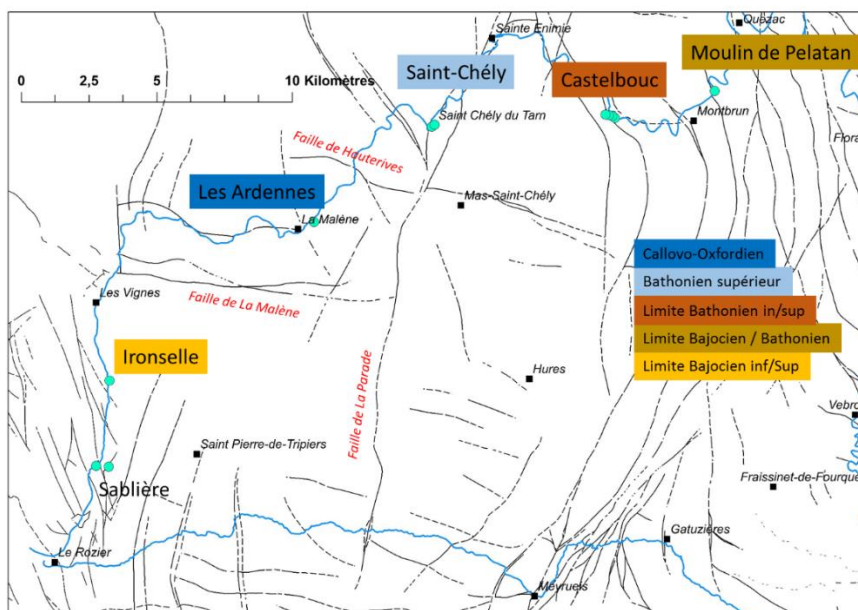
Figure 4 : Localisation des sources (cercles verts) ayant fait l'objet d'une reconnaissance de terrain. La position de l'exsurgence dans le log stratigraphique, pour chaque source, est indiquée par une couleur différente marquant l'âge des terrains.
