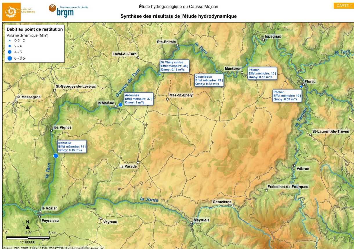
Figure 16 : Carte de synthèse des résultats de l'étude hydrodynamique.
