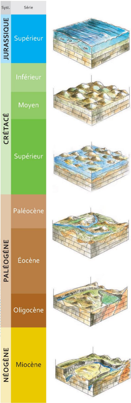
Figure 12 : Évolution géodynamique et karstique du Causse Méjean (extrait du bulletin n°6).
