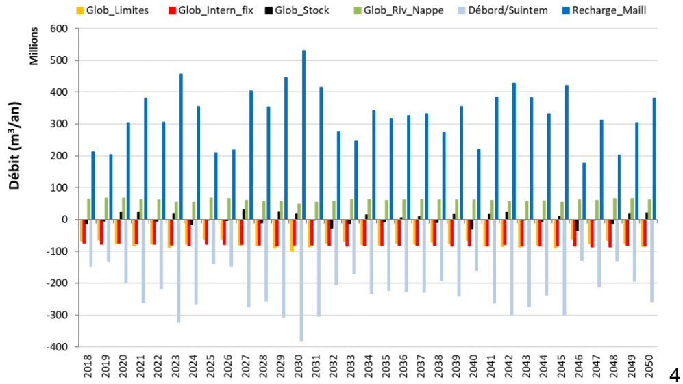
Evolution du bilan hydrique du scénario 4 (valeurs négatives indiquent une sortie d'eau de l'hydrosystème et valeurs positives indiquent une entrée d'eau dans l'hydrosystème)
