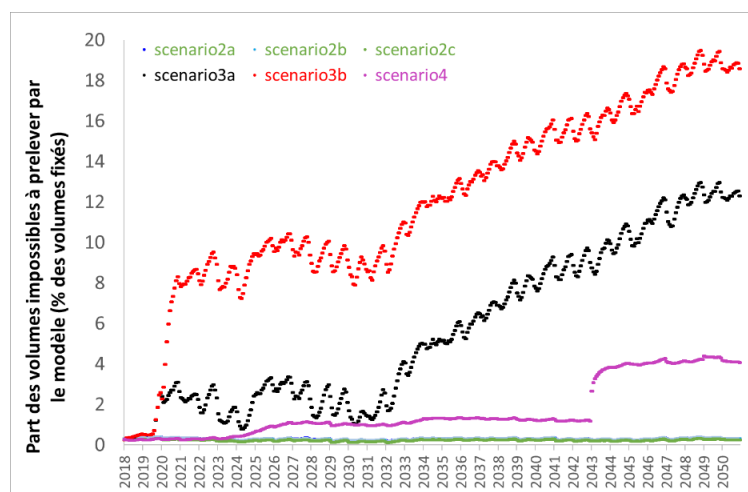
Figure 14. Proportion des volumes impossibles à prélever par le modèle dans la couche 4 aquifère carbonifère pour chaque scénario et variantes associées (scénario 2a.b.c : volumes prélevés moyens)
