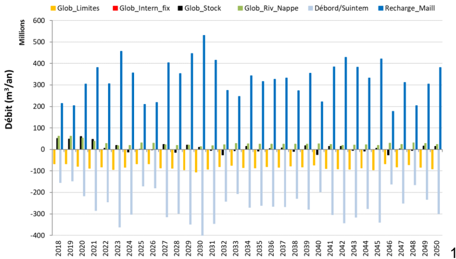
Figure 15 : Evolution des termes du bilan hydrique calculé de 2018 à 2050 à l'échelle de l'hydrosystème pour le scénario 1 avec arrêt des prélèvements (Les valeurs positives indiquent une entrée d'eau et les valeurs négatives une sortie d'eau dans l'hydrosystème).
