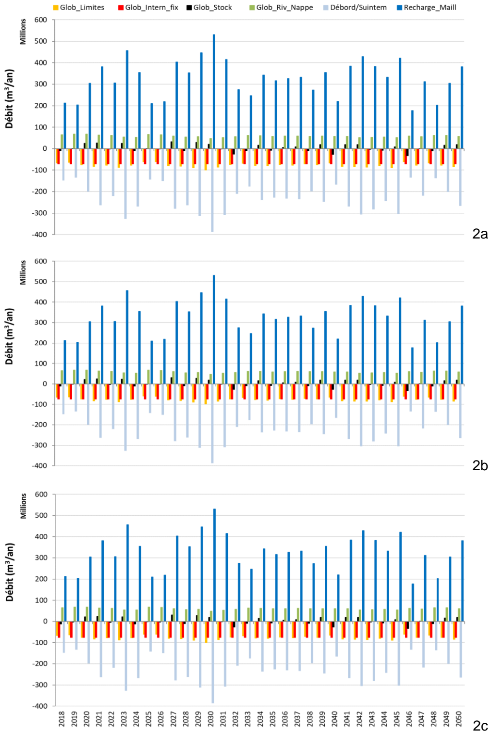
Evolution du bilan hydrique du scénario 2 et de ses variantes (valeurs négatives indiquent une sortie d'eau de l'hydrosystème et valeurs positives indiquent une entrée d'eau dans l'hydrosystème)
