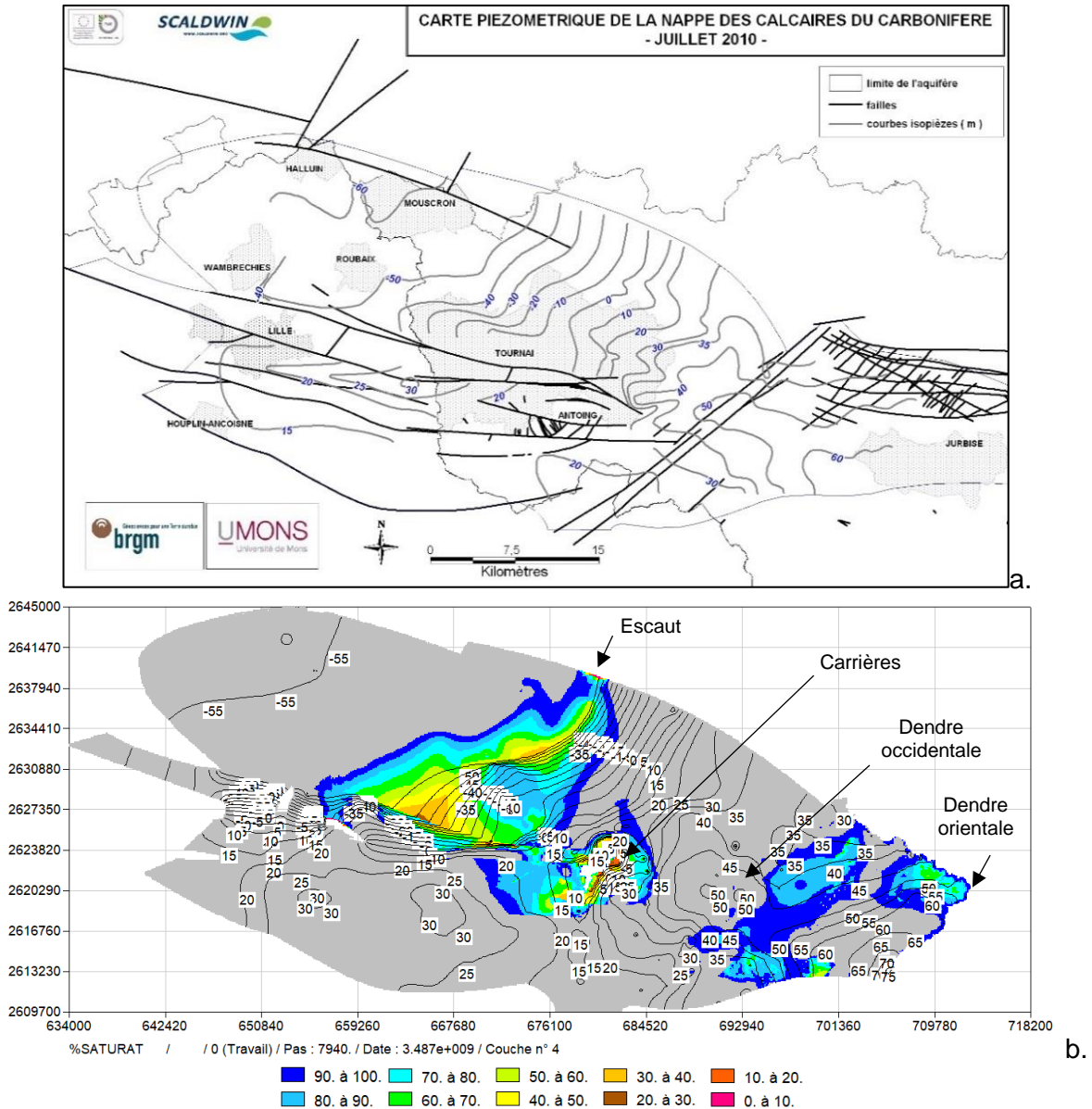
Figure 12. Cartes piézométriques 2010 des calcaires carbonifères (a) et simulée en 2010 (b) (isopiètes en mNGF, coordonnées x et y en mL2E), et saturation en eau simulée en 2010 (%) de la couche n°4 représentant l'aquifère des calcaires carbonifères (en gris 100% saturation indique une nappe captive ou semi-captive, les valeurs < 100% indiquent que la nappe est libre).
