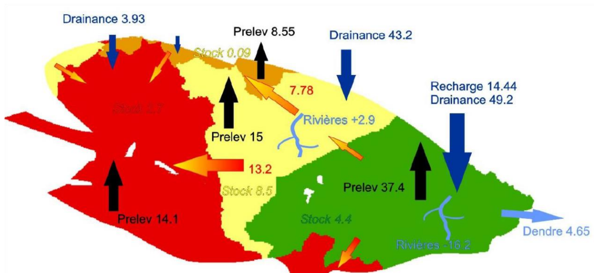
Figure 10 : Représentation des volumes échangés par masses d'eau (Mm 3 par an) au sein des calcaires carbonifères calculés pour l'année 2010 (Rorive et Bastien, 2016). En rouge masse d'eau française 1015, en orange masse d'eau flamande ss_1300, en jaune masse d'eau wallonne RWE060, en vert masse d'eau wallonne RWE013.
