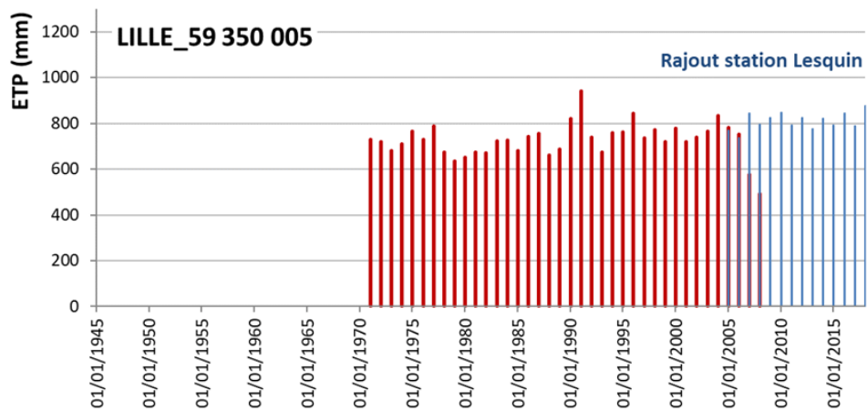
Historiques d'ETP (EvapoTranspiration Potentielle) des stations de suivi météorologique, Lille (en rouge) et Lesquin (en bleu)
