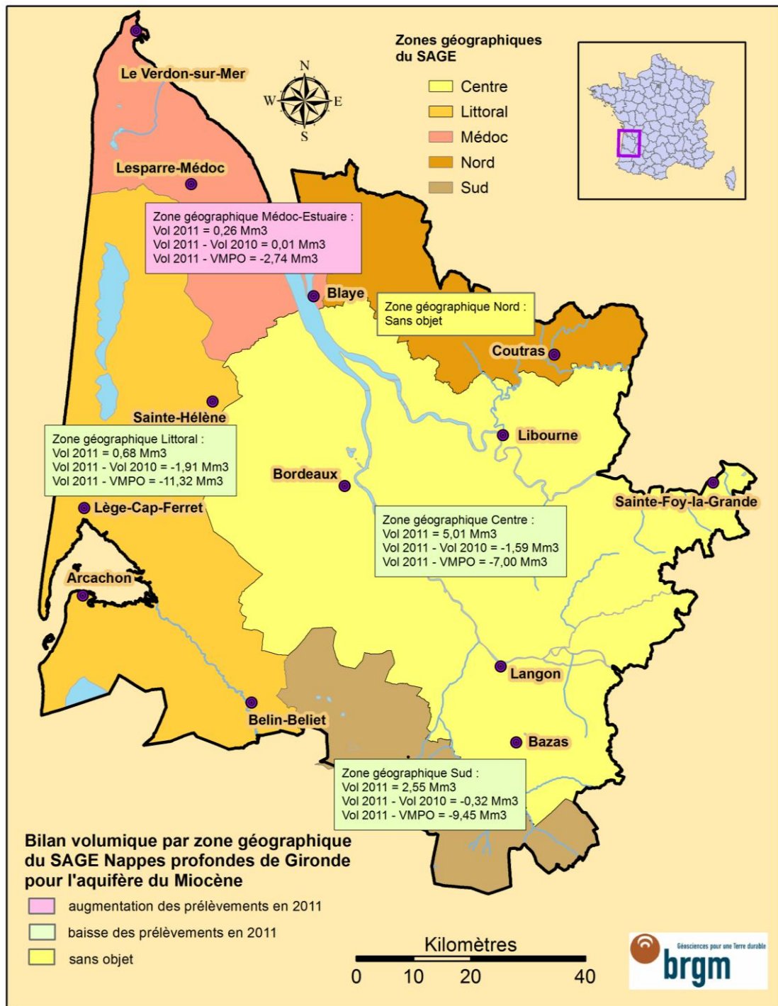
Illustration 42 : Evolution des prélèvements par unité de gestion du SAGE « Nappes profondes » pour les nappes du Miocène
