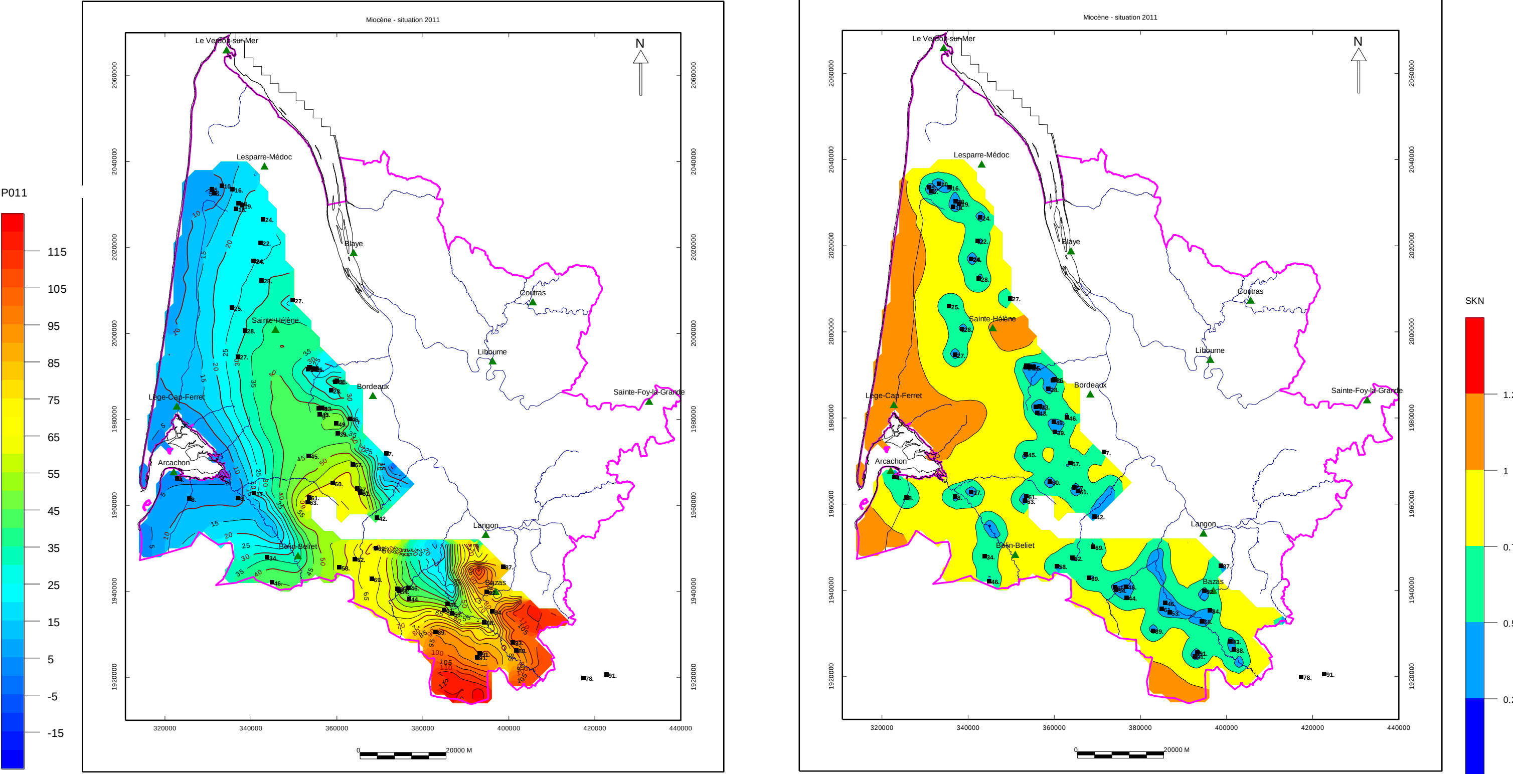
Illustration 44 : Carte piézométrique 2011 du Miocène et carte d'indice de confiance (isopièzes en m NGF et indice de confiance d'autant plus proche de 0 que la fiabilité est bonne)
