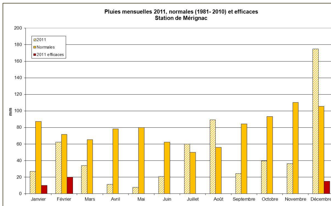
Illustration 2 : Pluies mensuelles 2011, normales et efficaces sur le poste de Mérignac
