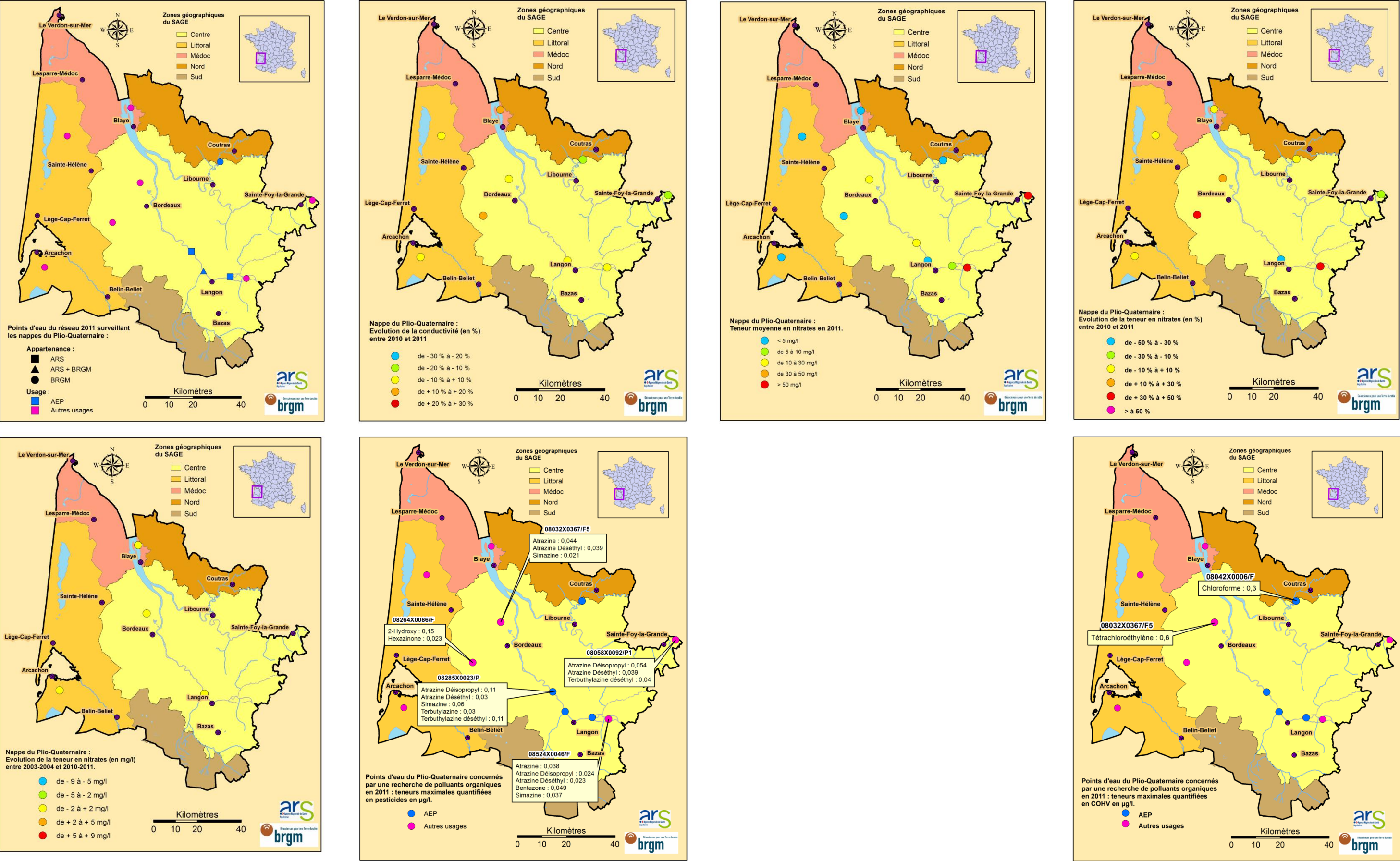
Illustration 56 : Valorisation des données chimiques pour les nappes du Plio-Quaternaire
