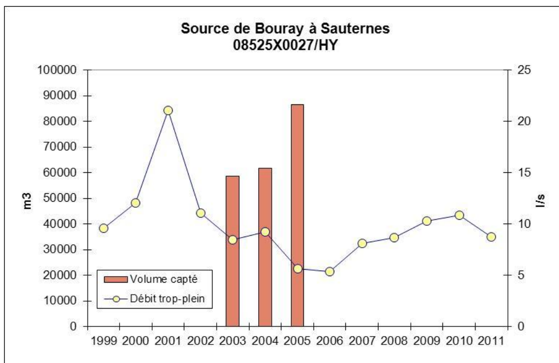
Illustration 46 : Volumes captés et débits moyens du trop-plein de la source du Bouray à Sauternes
