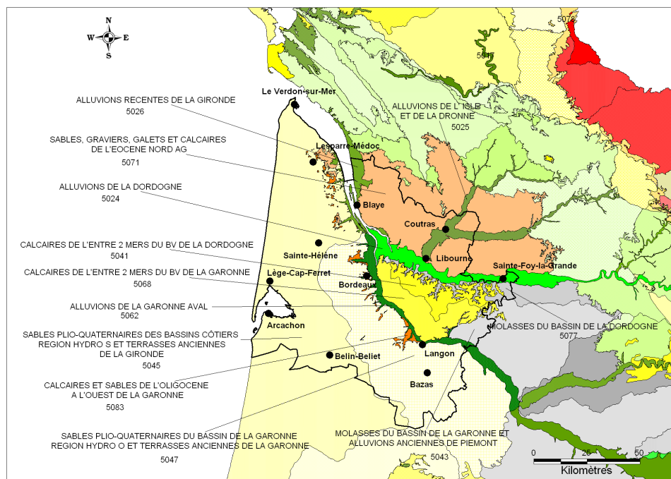
Illustration 50 : Emprises des masses d'eau libres sur le département de la Gironde
