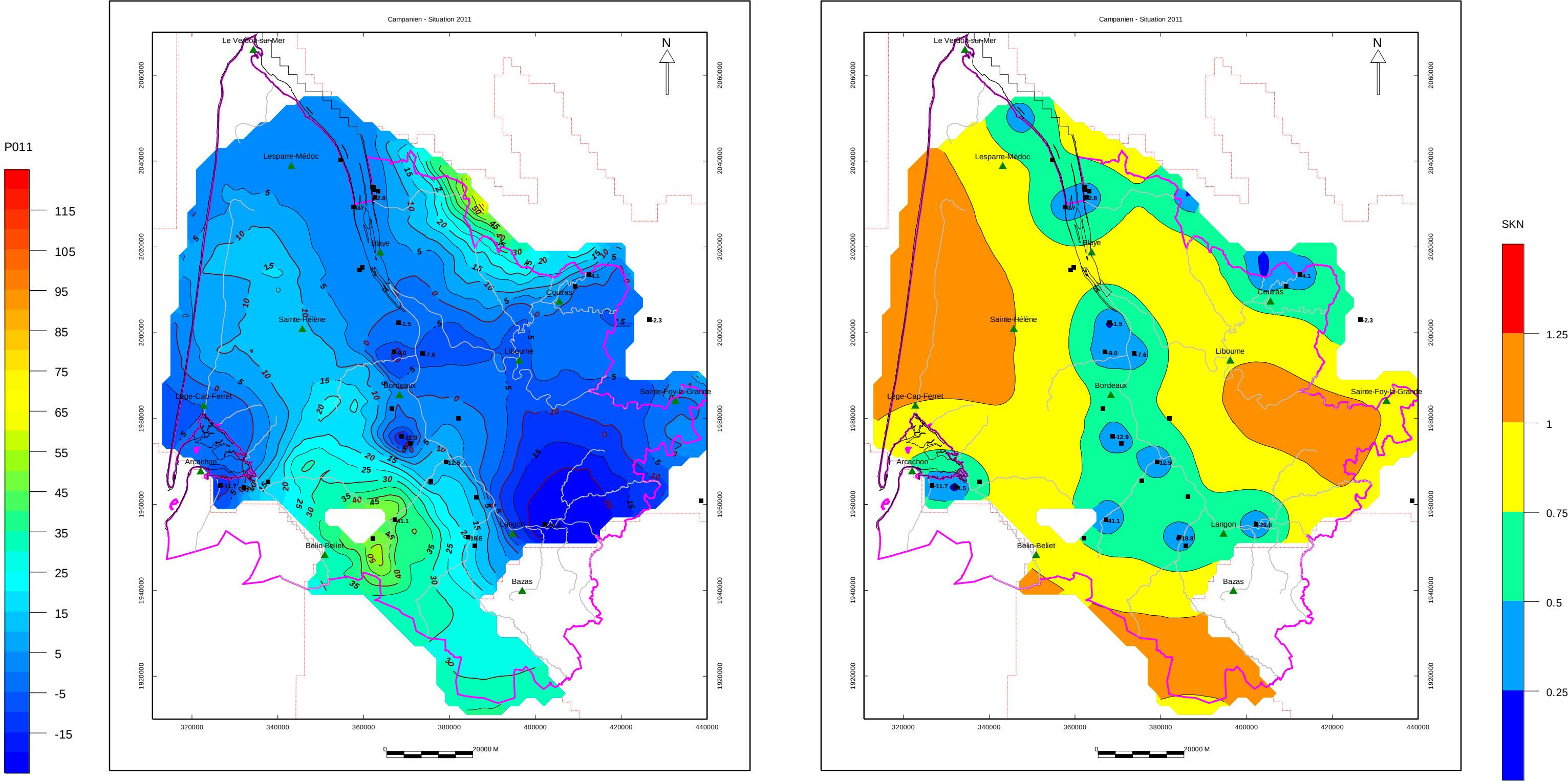
Illustration 14 : Nappe du sommet du Crétacé supérieur : carte piézométrique 2011 et carte d'indice de confiance (isopièzes en m NGF et indice de confiance d'autant plus proche de 0 que la fiabilité est bonne)
