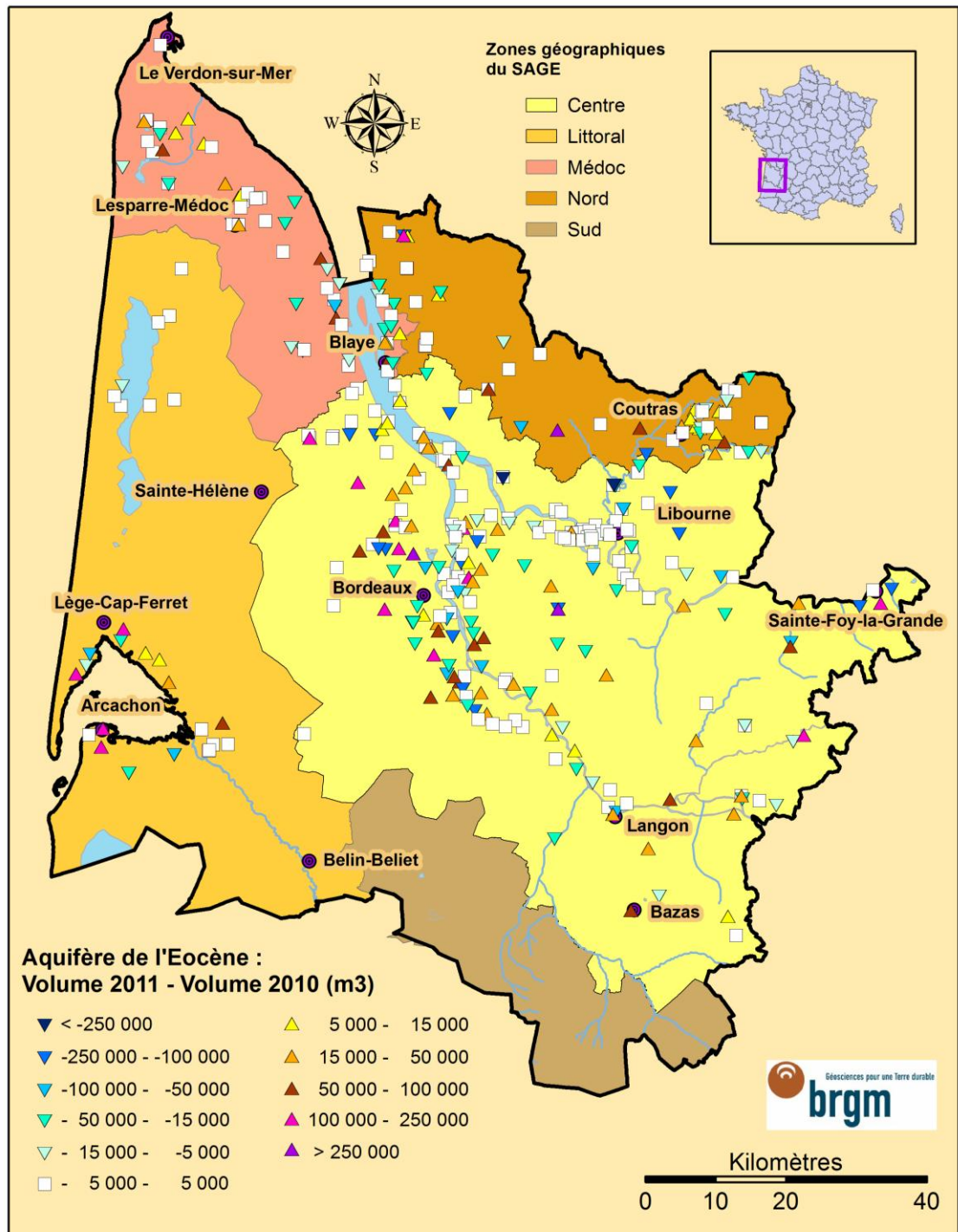
Illustration 20 : Evolution des prélèvements entre 2010 et 2011 pour les nappes de l'Eocène
