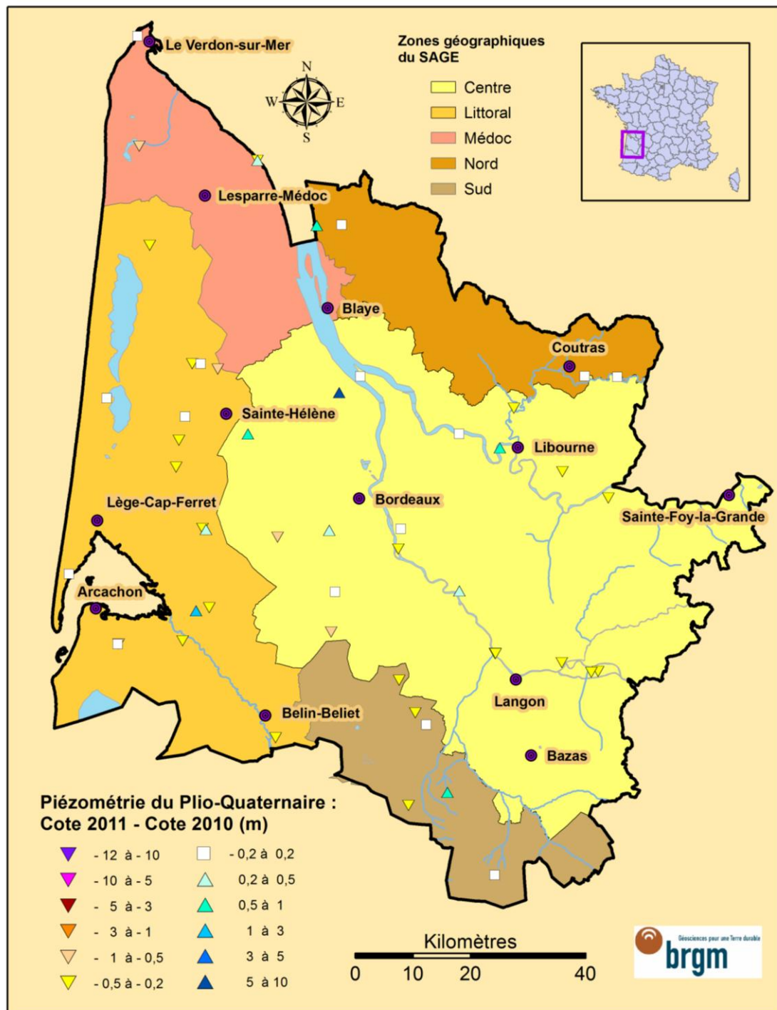
Illustration 53 : Evolution de la piézométrie entre 2010 et 2011 pour les nappes du Plio-Quaternaire
