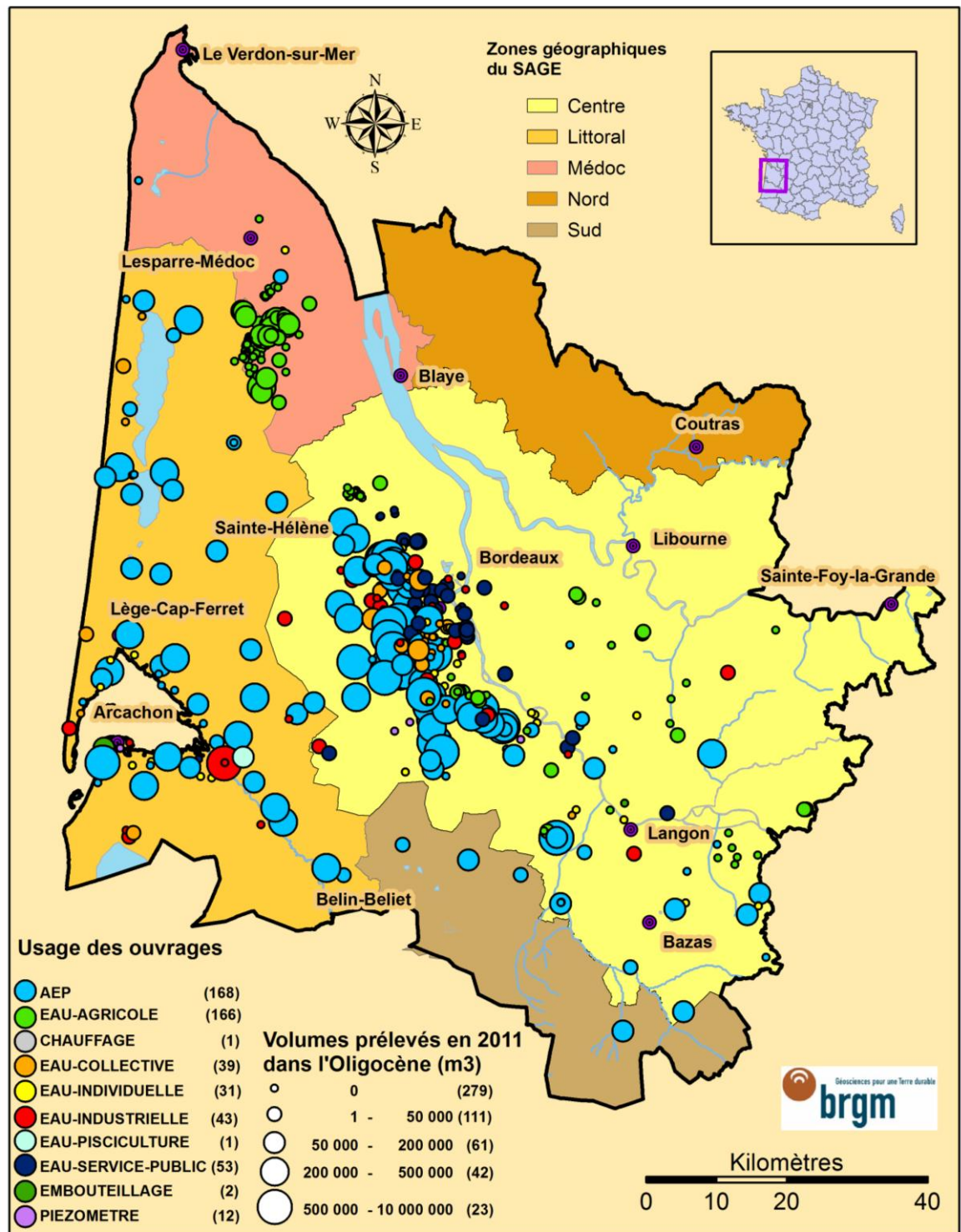
Illustration 28 : Carte de répartition des ouvrages et des prélèvements pour les nappes de l'Oligocène en 2011
