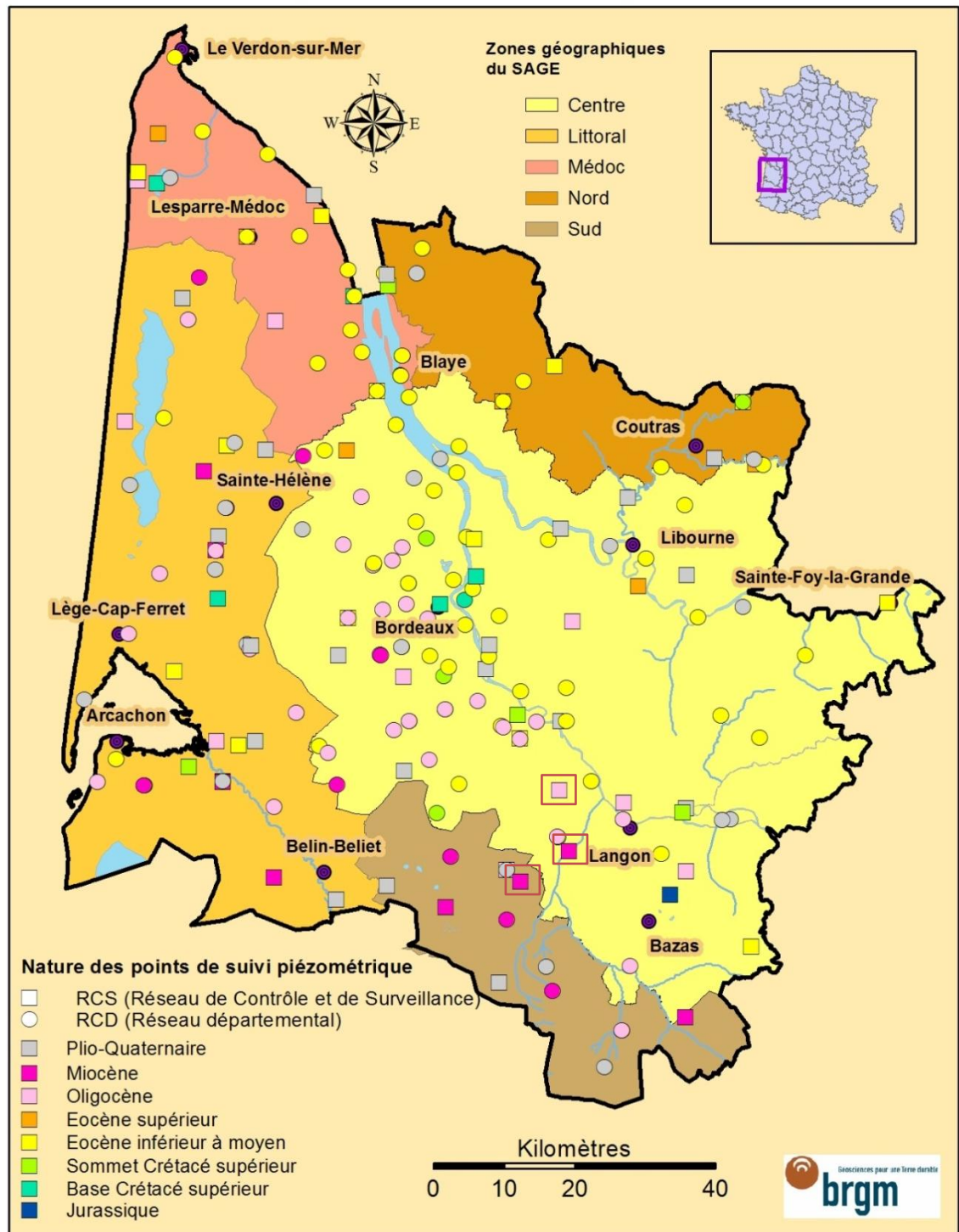
Illustration 4 : Localisation des points de mesures piézométriques en 2011 (sources suivies par jaugeages entourées par des cadres rouges)
