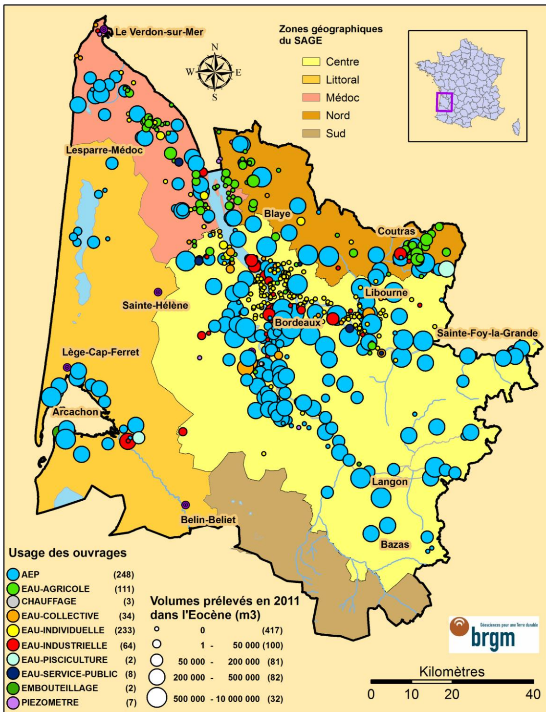
Illustration 19 : Carte de répartition des ouvrages et des prélèvements pour les nappes de l'Eocène en 2011
