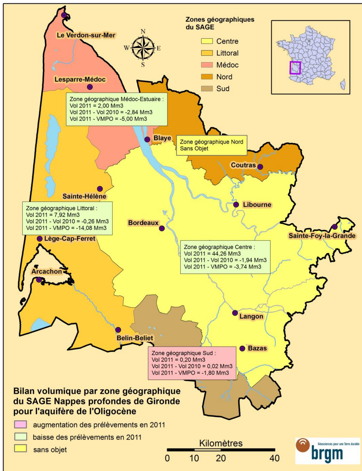
Illustration 32 : Evolution des prélèvements par unité de gestion du SAGE « Nappes profondes » pour les nappes de l'Oligocène
