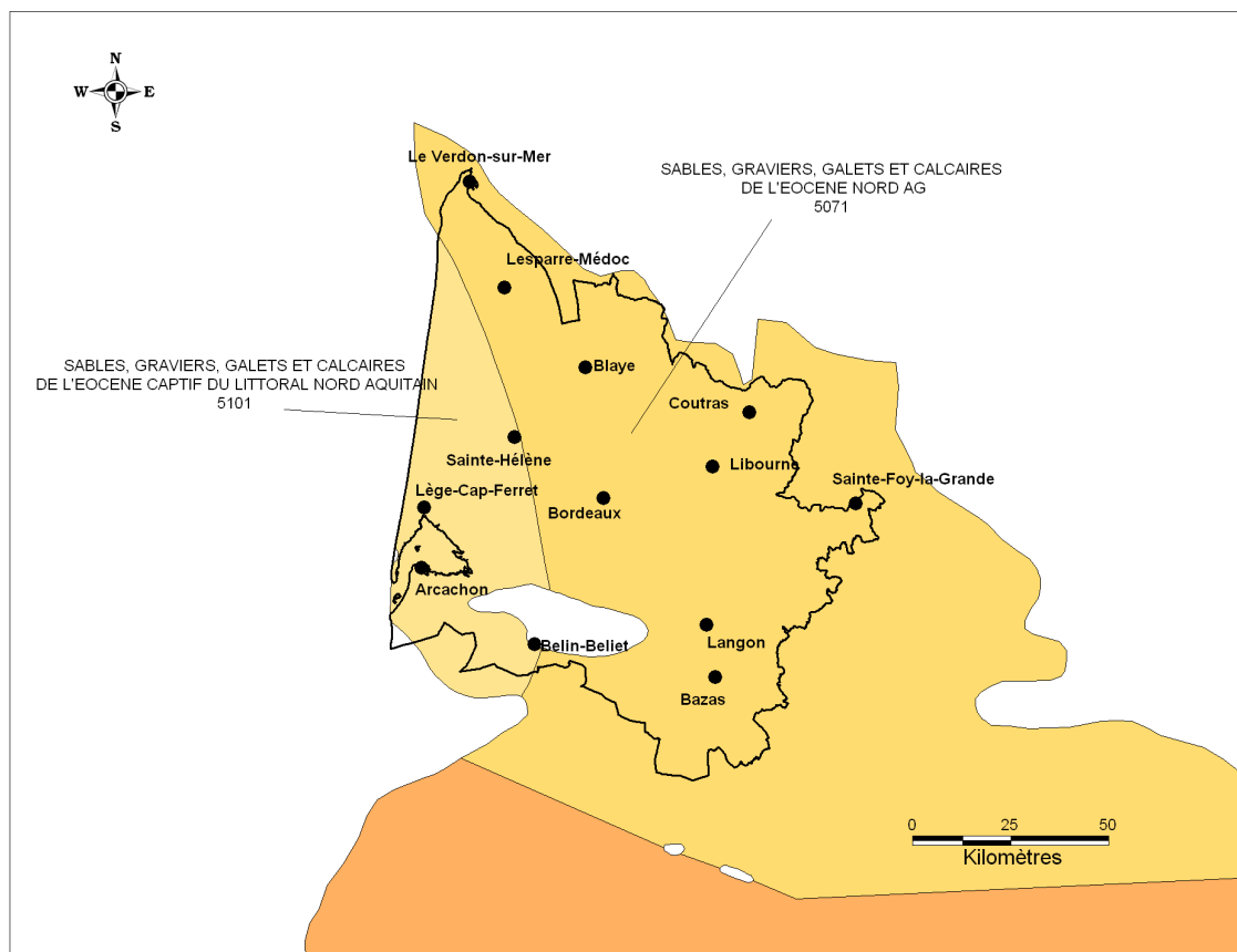
Illustration 18 : Emprises des masses d'eau 5071 ou FG071 et 5101 ou FG101 (Eocène captif)
