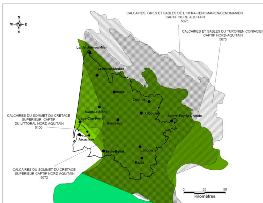
Illustration 8 : Emprises des masses d'eau 5072 ou FG072, 5073 ou FG073, 5075 ou FG075 et 5100 ou FG100 (Crétacé supérieur captif)
