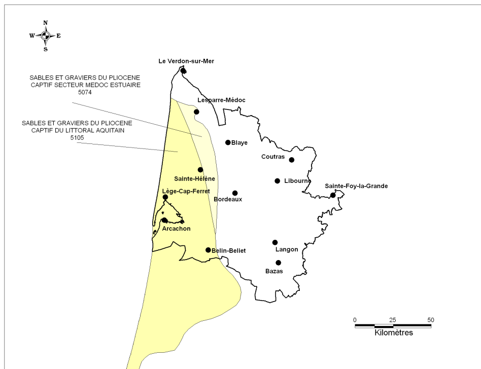
Illustration 49 : Emprises des masses d'eau 5074 ou FG074 et 5105 ou FG105 (Pliocène captif)
