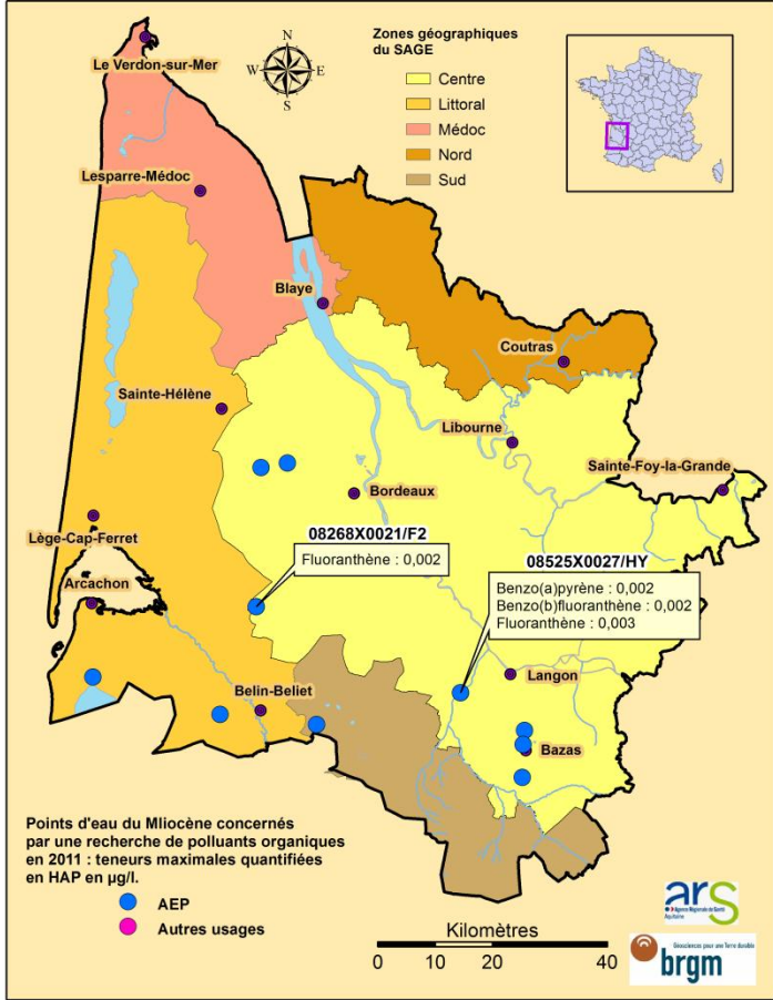
Illustration 48 : Valorisation des données chimiques pour les nappes du Miocène
