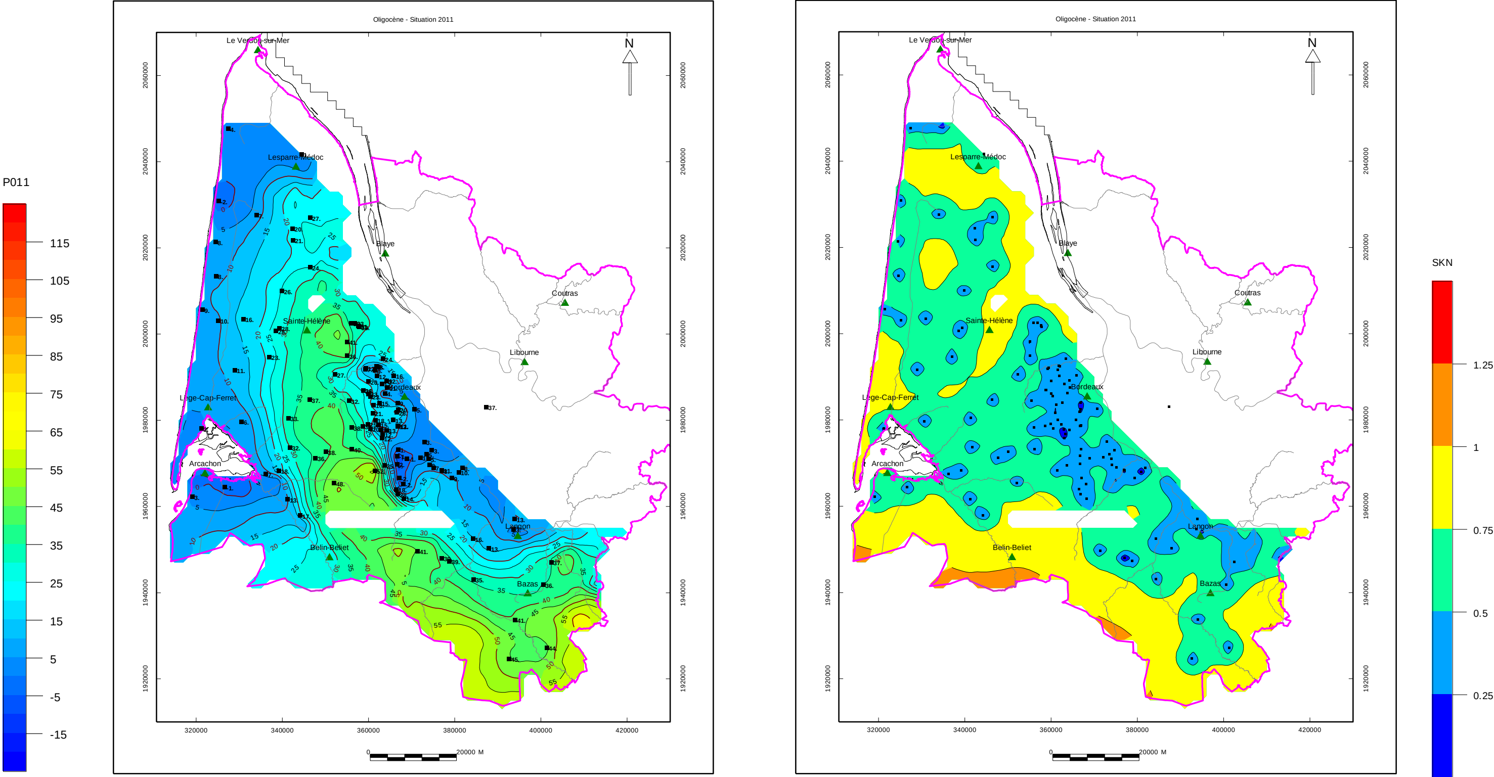
Illustration 34 : Nappe des calcaires de l'Oligocène : carte piézométrique 2011 et carte d'indice de confiance (isopièzes en m NGF et indice de confiance d'autant plus proche de 0 que la fiabilité est bonne)
