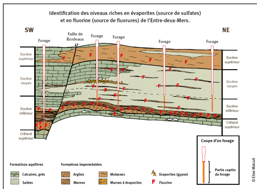
Illustration 26 : Localisation des sources de sulfates et de fluor dans les formations de l'Eocène (d'après Revue de l'Agence de l'Eau Adour-Garonne n°119)
