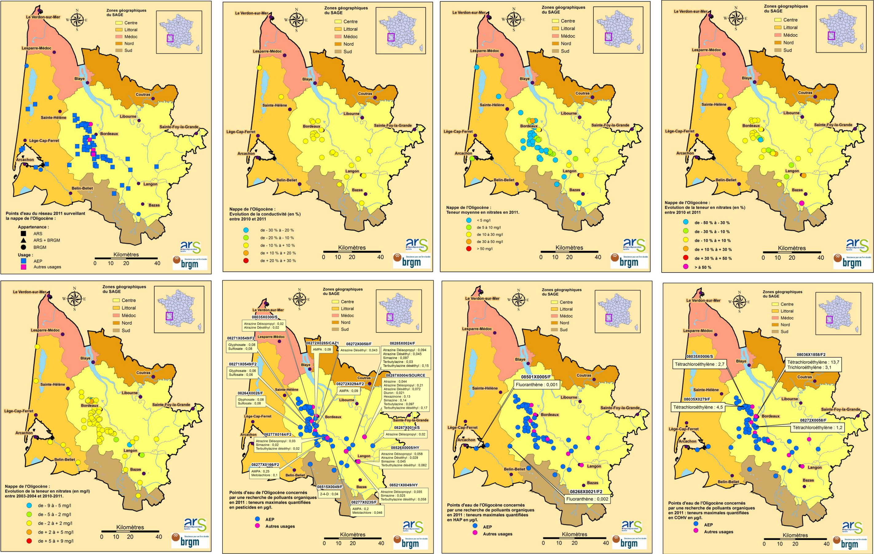
Illustration 38 : Valorisation des données chimiques pour la nappe de l'Oligocène
