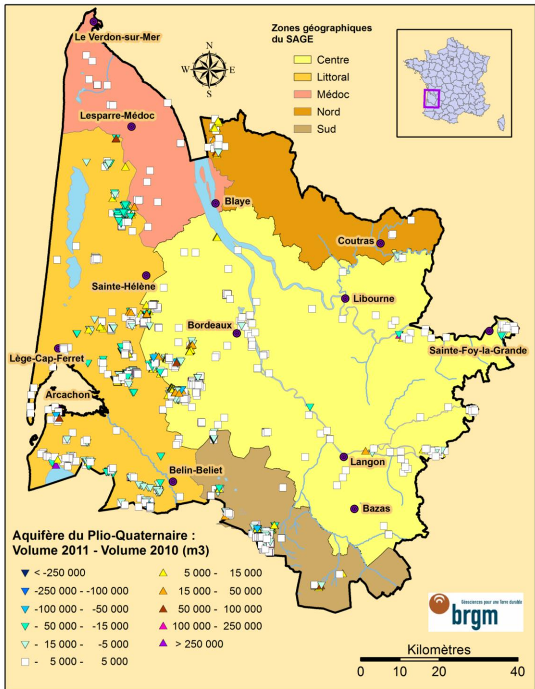
Illustration 52 : Evolution des prélèvements entre 2010 et 2011 pour les nappes du Plio-Quaternaire
