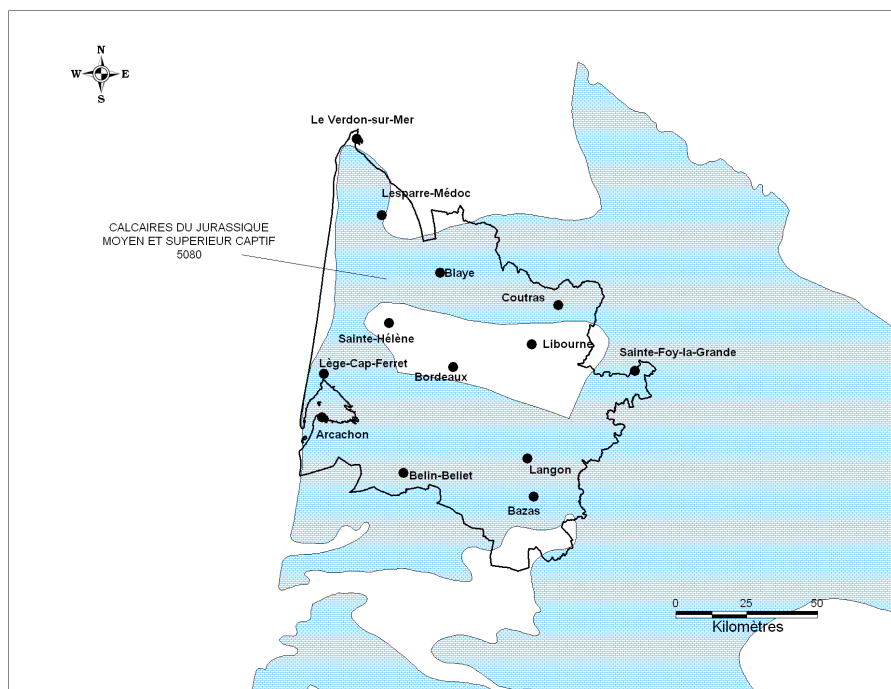
Illustration 7 : Emprise de la masse d'eau 5080 ou FG080 (Jurassique moyen et supérieur captif)
