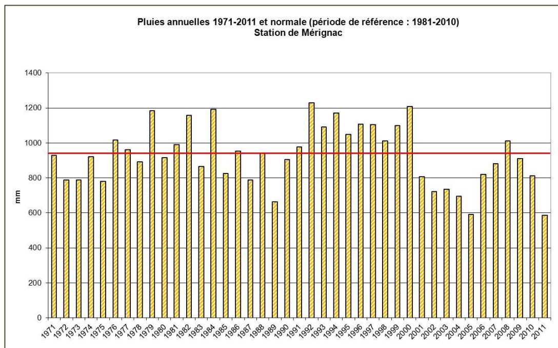
Illustration 1 : Historique des pluies annuelles sur le poste de Mérignac (1971-2011)
