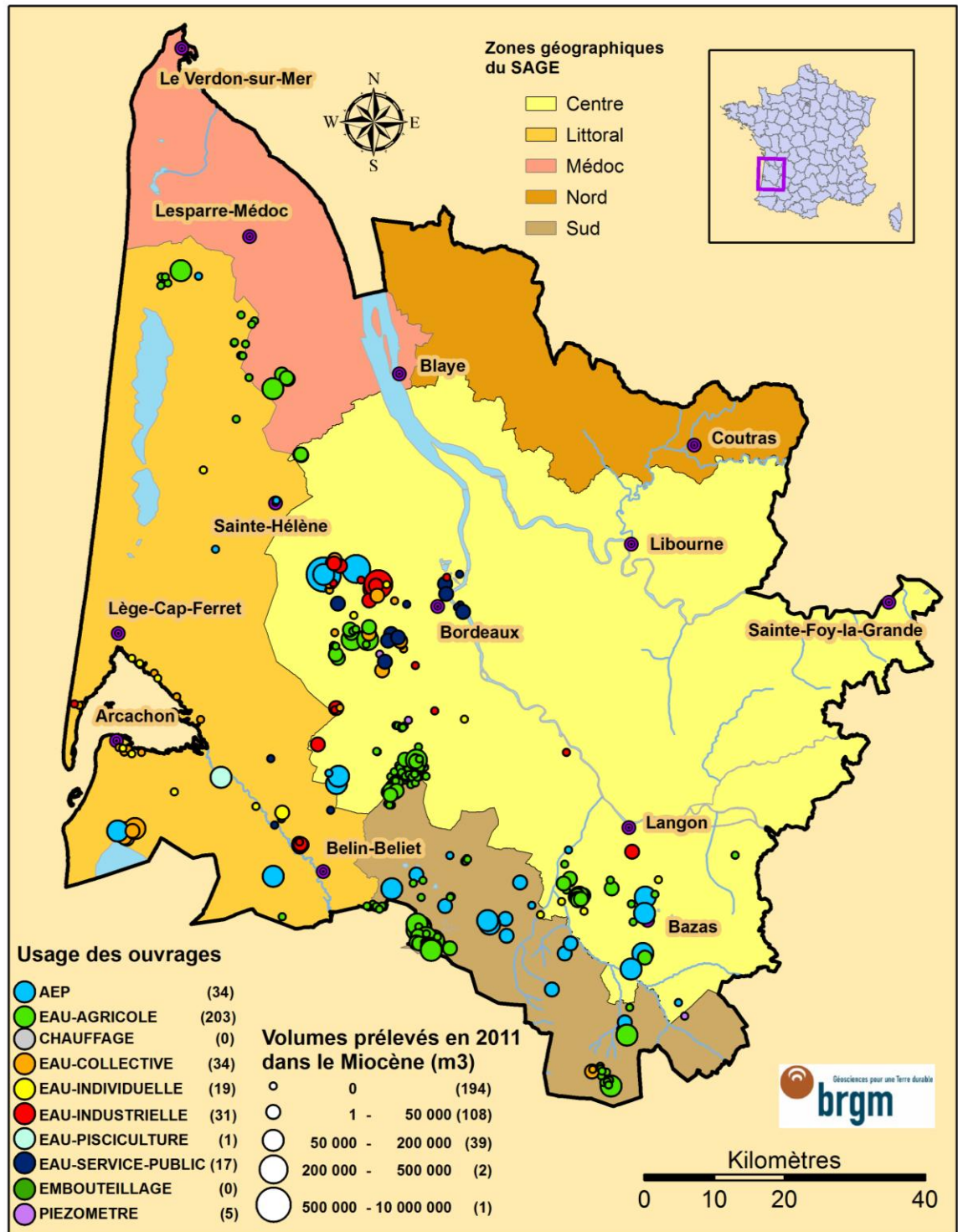
Illustration 40 : Carte de répartition des ouvrages et des prélèvements pour les nappes du Miocène en 2011
