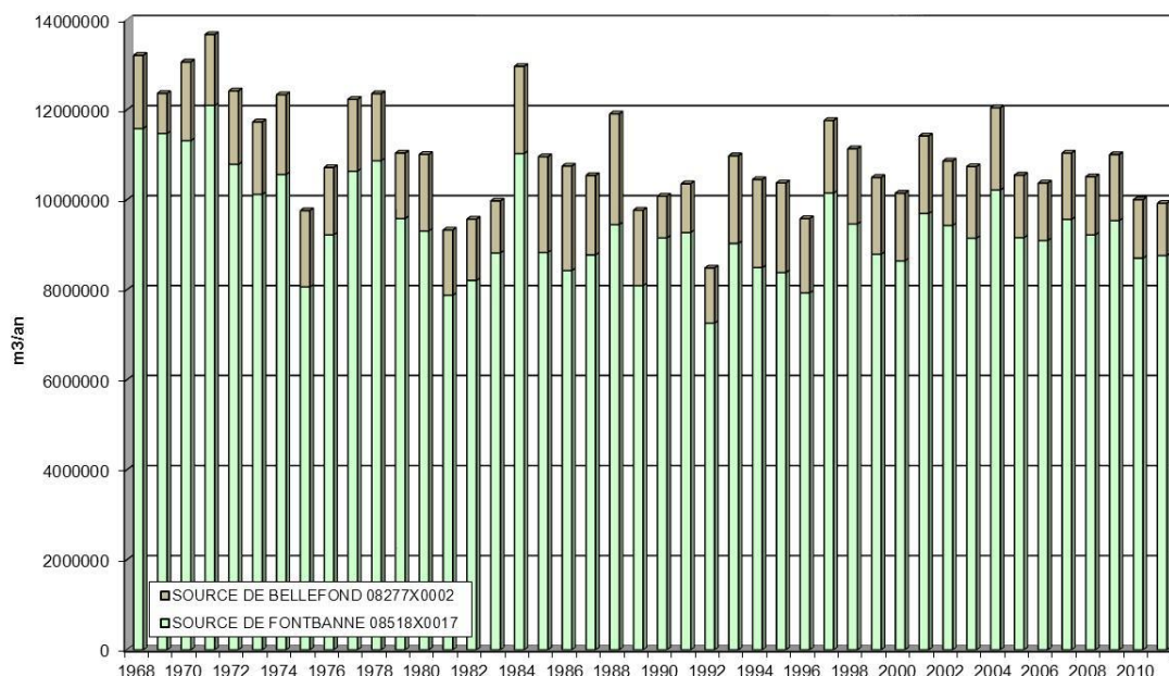
Illustration 31 : Evolution des prélèvements sur les sources situées au sud de Bordeaux (Fontbanne à Budos et Bellefond à Castres-sur-Gironde) de 1968 à 2011
