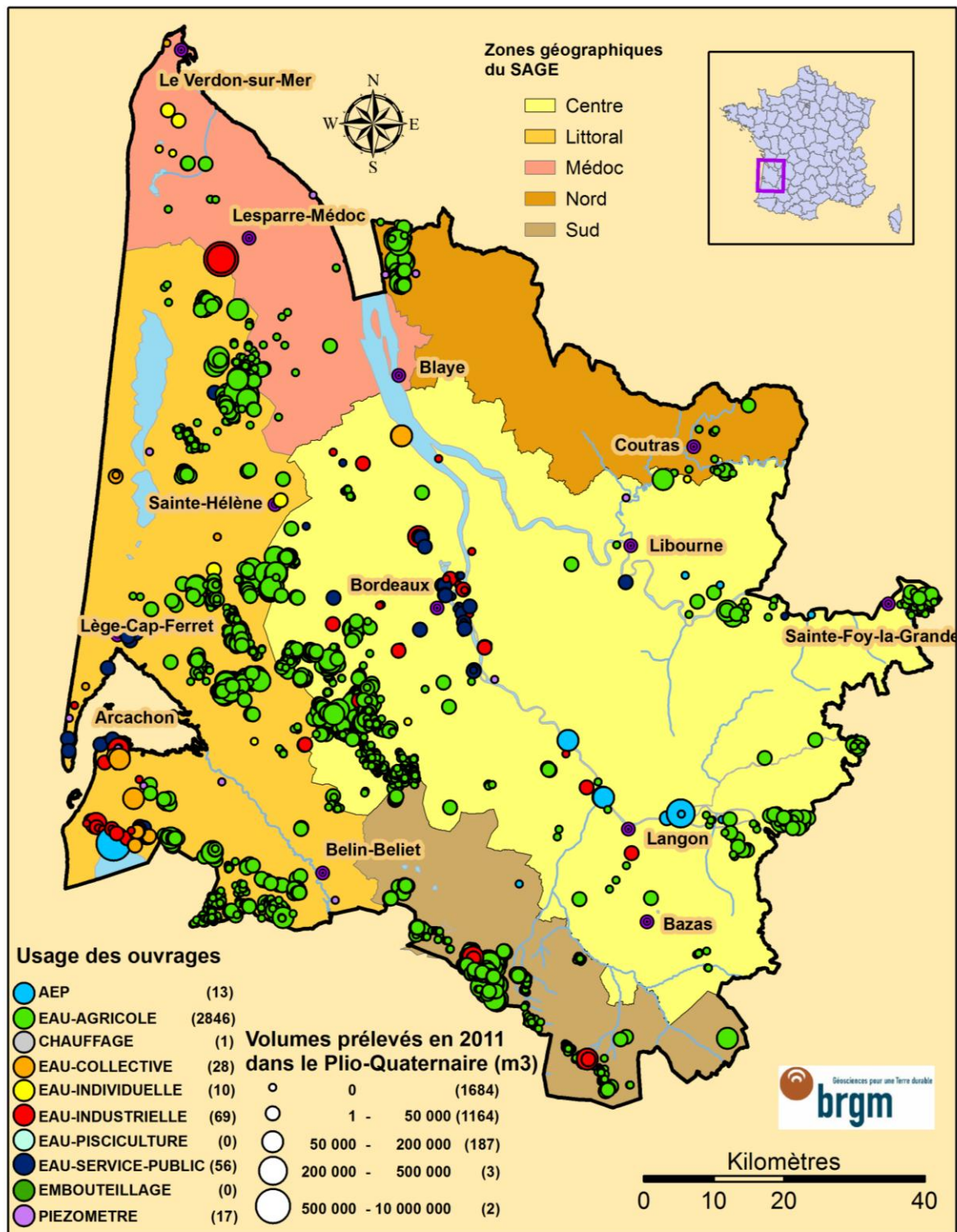
Illustration 51 : Carte de répartition des ouvrages et des prélèvements pour les nappes du Plio-Quaternaire en 2011
