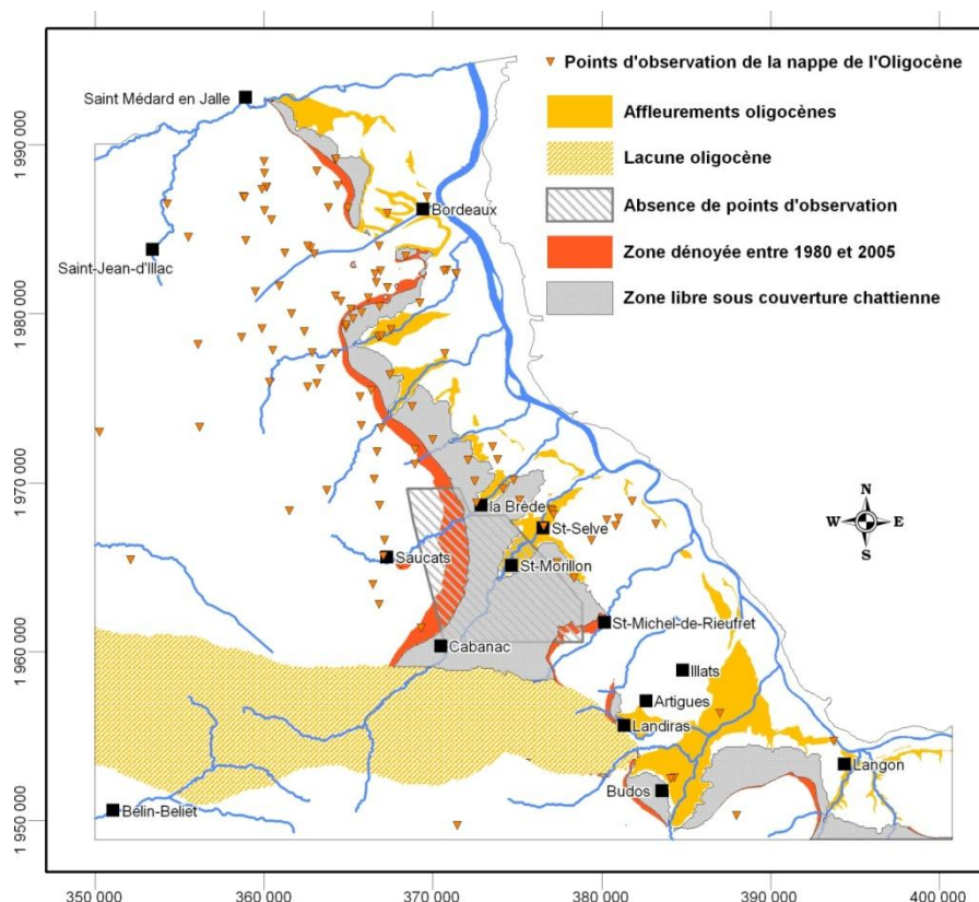
Illustration 37 : Secteur étudié dans le cadre du projet RODEO d'après rapport BRGM/RP-61559-FR
