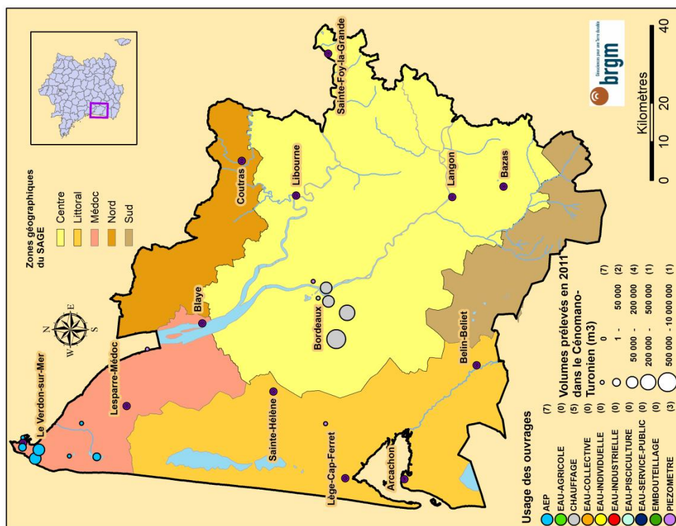
Illustration 9 : Carte de répartition des ouvrages et des prélèvements pour les nappes de la base et du sommet du Crétacé supérieur en 2011
