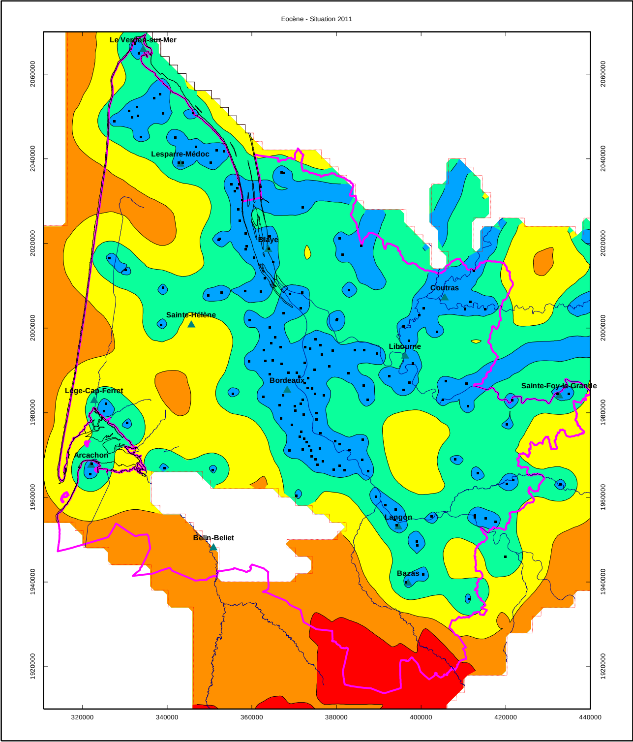
Illustration 23 : Nappe de l'Eocène inférieur à moyen : carte piézométrique 2011 et carte d'indice de confiance (isopièzes en m NGF et indice de confiance d'autant plus proche de 0 que la fiabilité est bonne)
