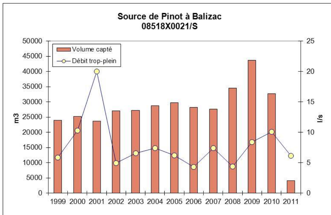
Illustration 45 : Volumes captés et débits moyens du trop-plein de la source de Pinot à Balizac
