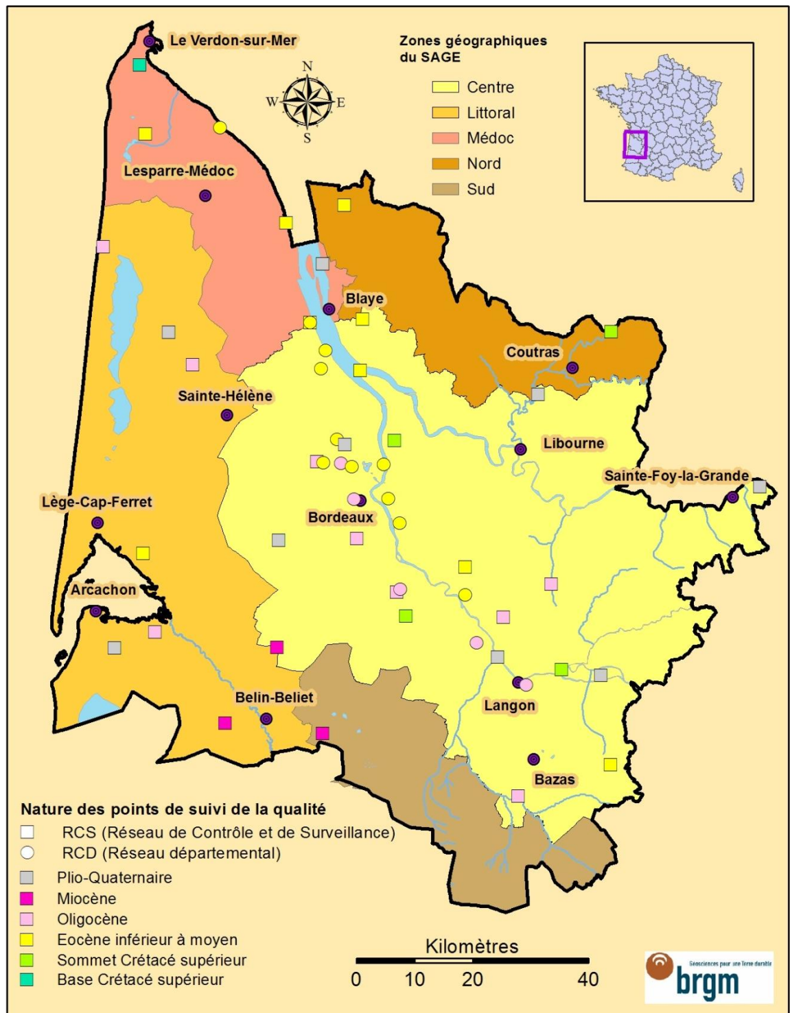
Illustration 5 : Localisation des points de mesures de la qualité en 2011
