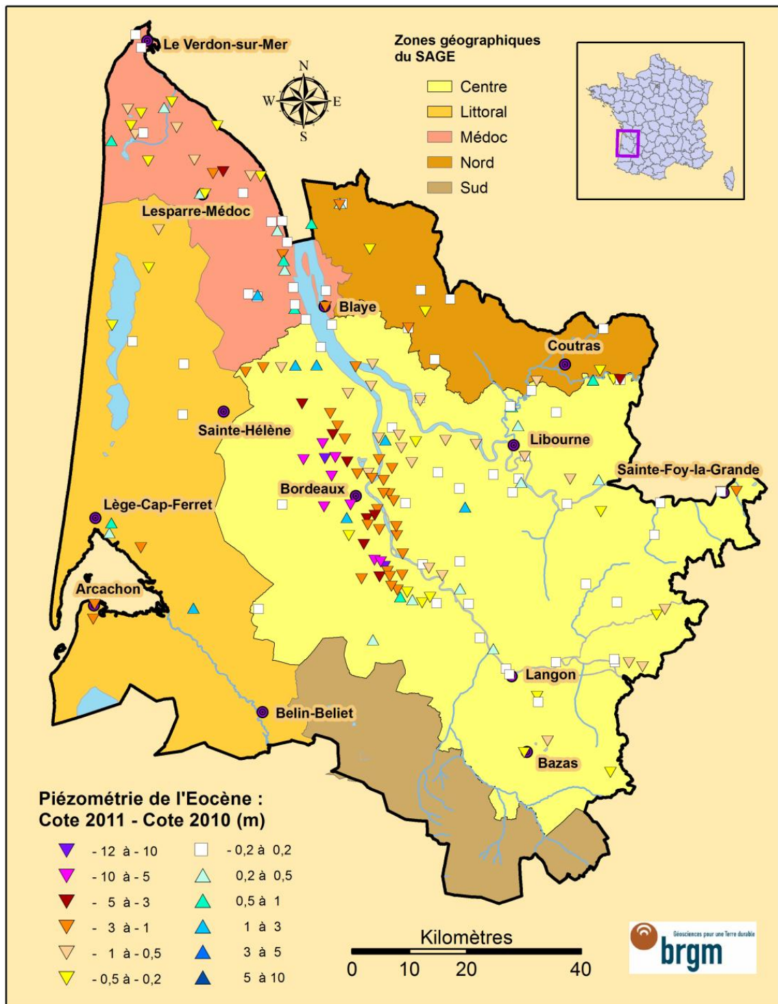
Illustration 22 : Evolution de la piézométrie entre 2010 et 2011 pour les nappes de l'Eocène
