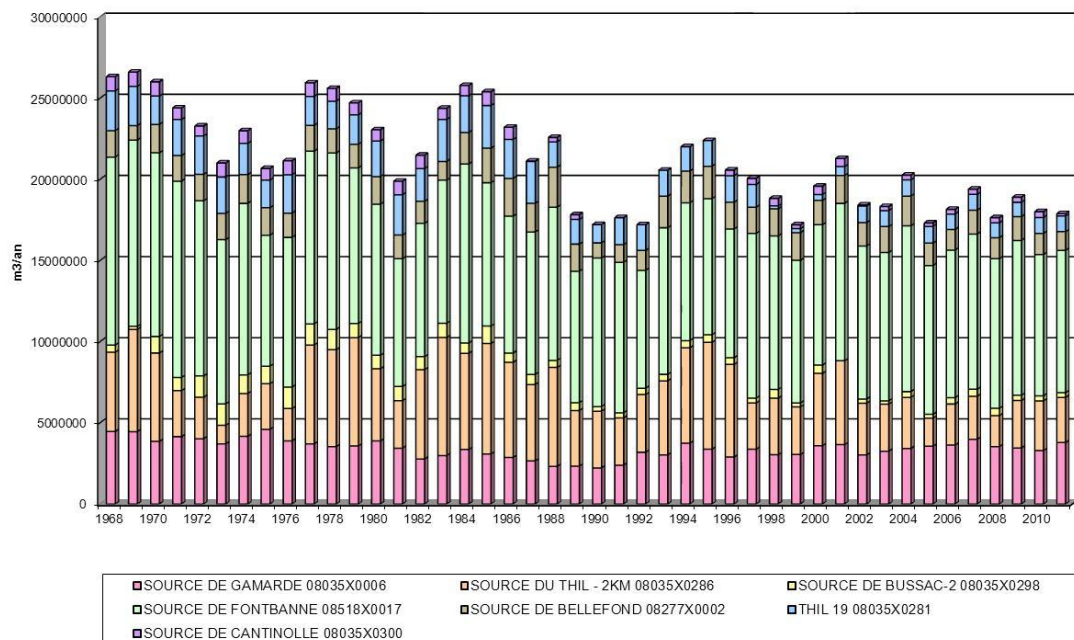
Illustration 30 : Evolution des prélèvements sur les sources oligocènes de 1968 à 2011
