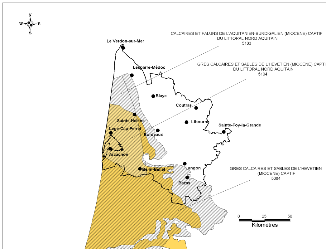
Illustration 39 : Emprises des masses d'eau 5084 ou FG084, 5103 ou FG103 et 5104 ou FG104 (Miocène captif)
