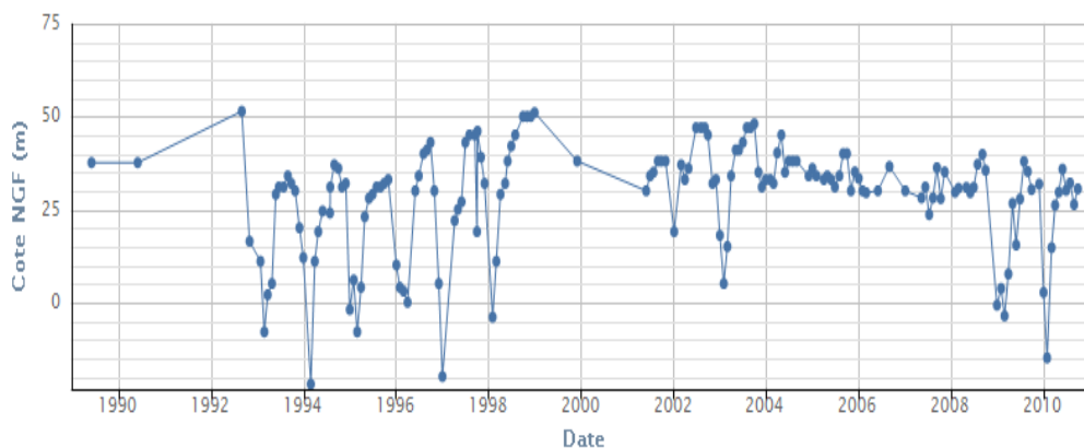
Illustration 12 : Evolution de la piézométrie sur l'ouvrage jurassique 08502X0069/GLTP1
