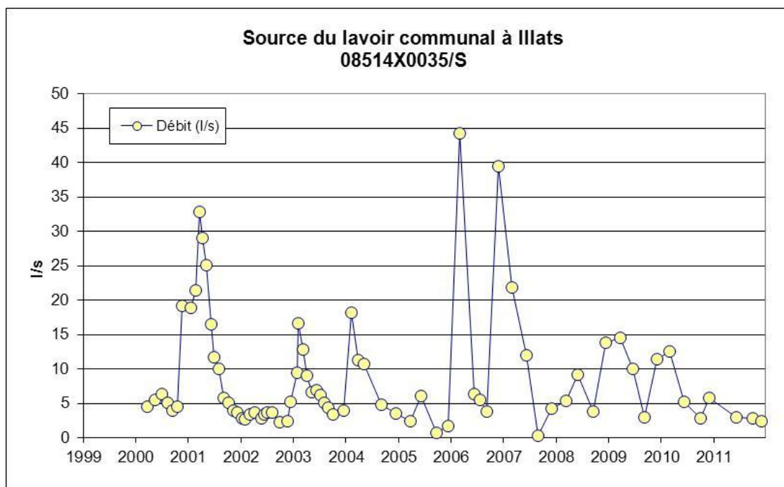
Illustration 35 : Débits de la source du lavoir communal à Illats
