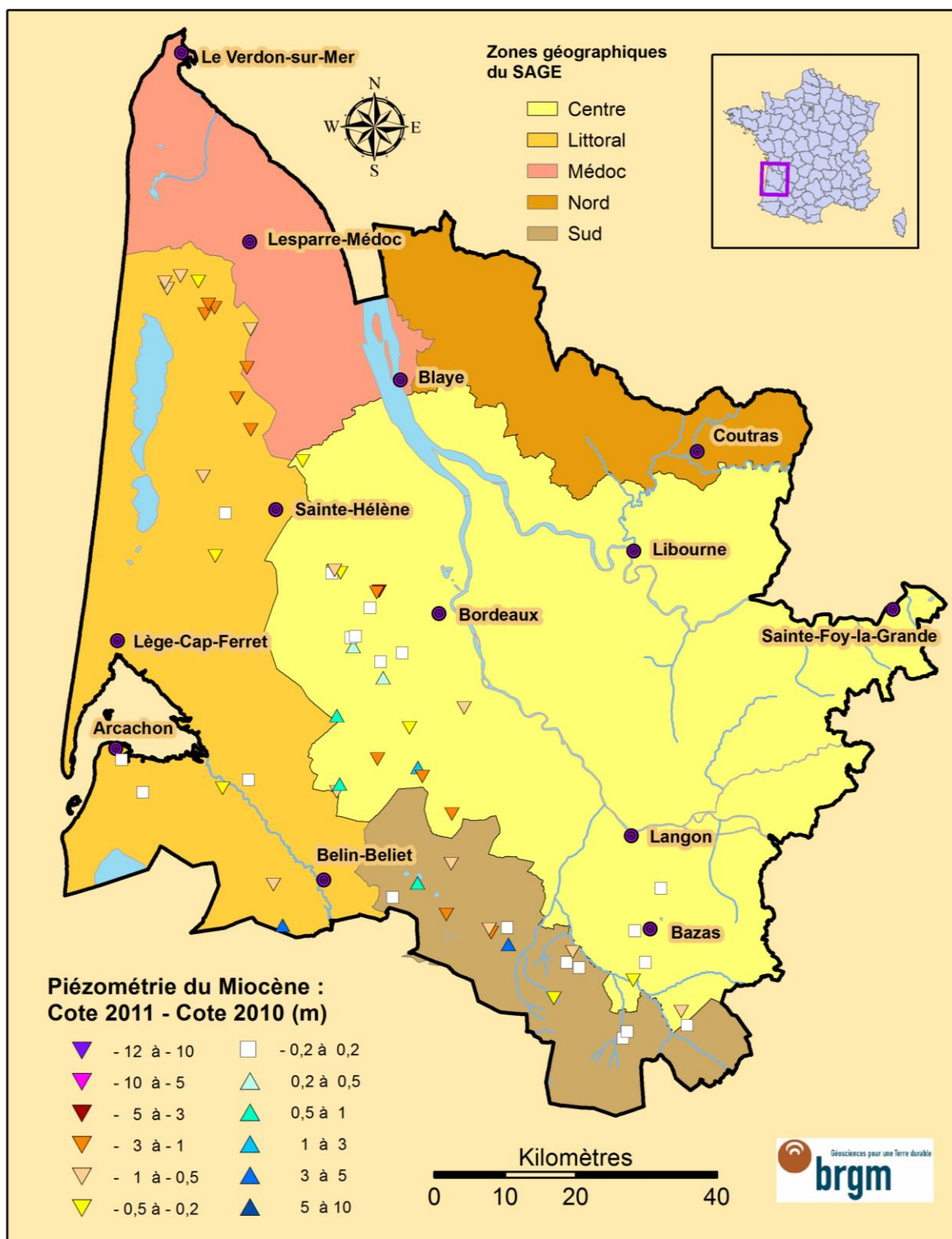
Illustration 43 : Evolution de la piézométrie entre 2010 et 2011 pour les nappes du Miocène
