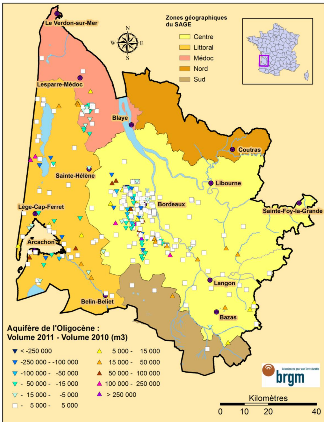
Illustration 29 : Evolution des prélèvements entre 2010 et 2011 pour les nappes de l'Oligocène
