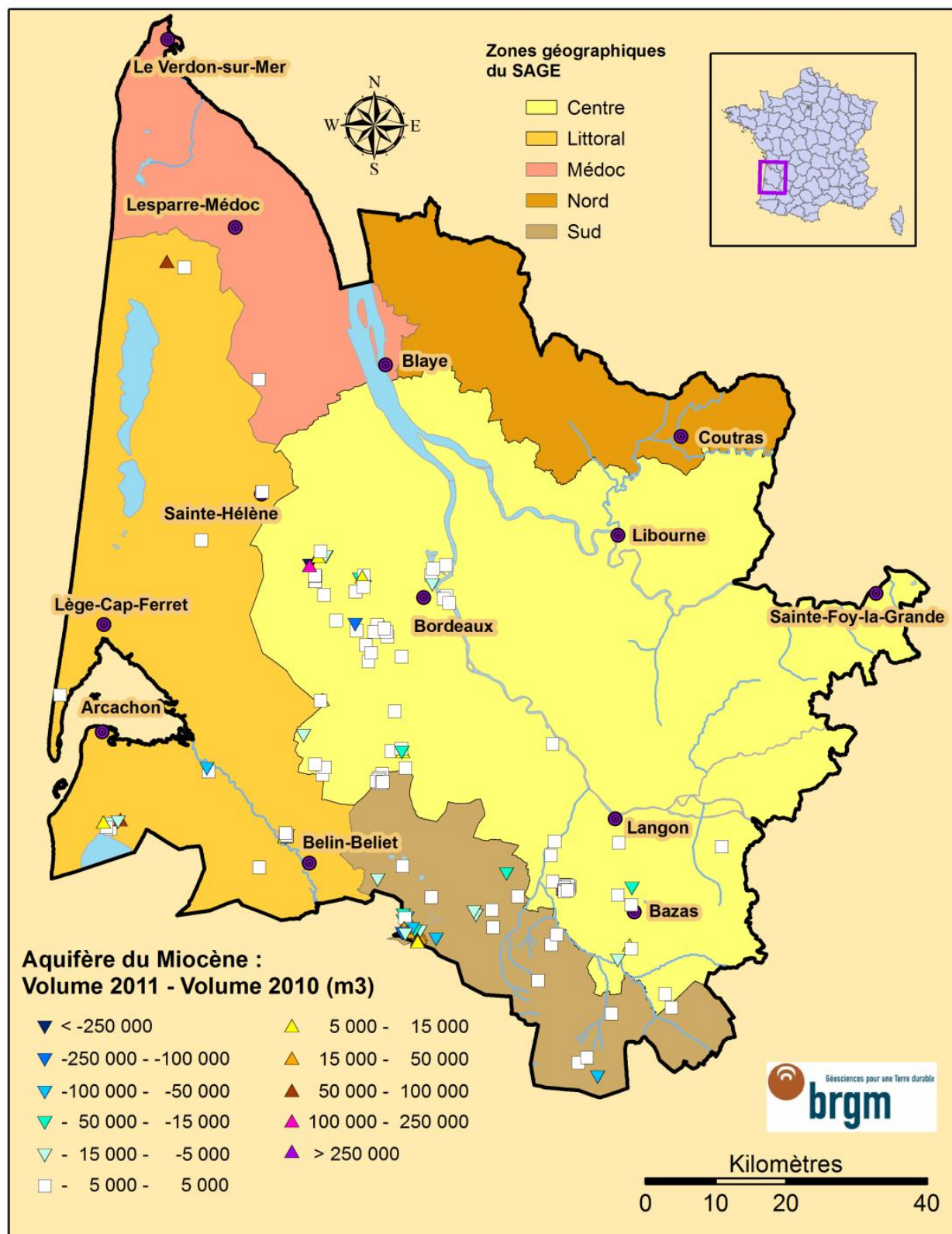
Illustration 41 : Evolution des prélèvements entre 2010 et 2011 pour les nappes du Miocène
