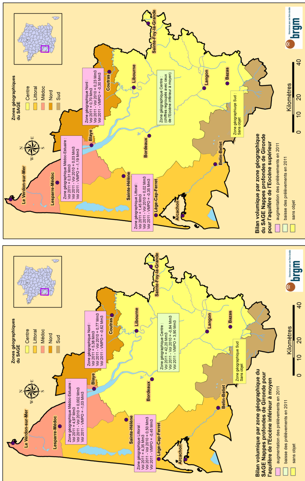
Illustration 21 : Evolution des prélèvements par zone géographique du SAGE « Nappes profondes » pour les nappes de l'Eocène inférieur à moyen et supérieur
