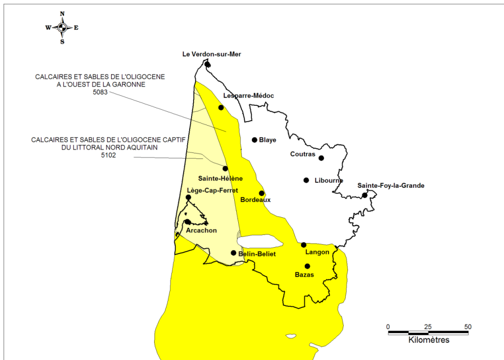
Illustration 27 : Emprises des masses d'eau 5083 ou FG083 et 5102 ou FG102 (Oligocène captif)
