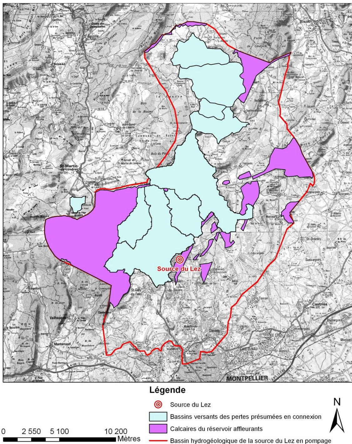
Illustration 12 : Limites de l'impluvium de l'aquifère du Lez et bassin hydrogéologique en régime de pompage
