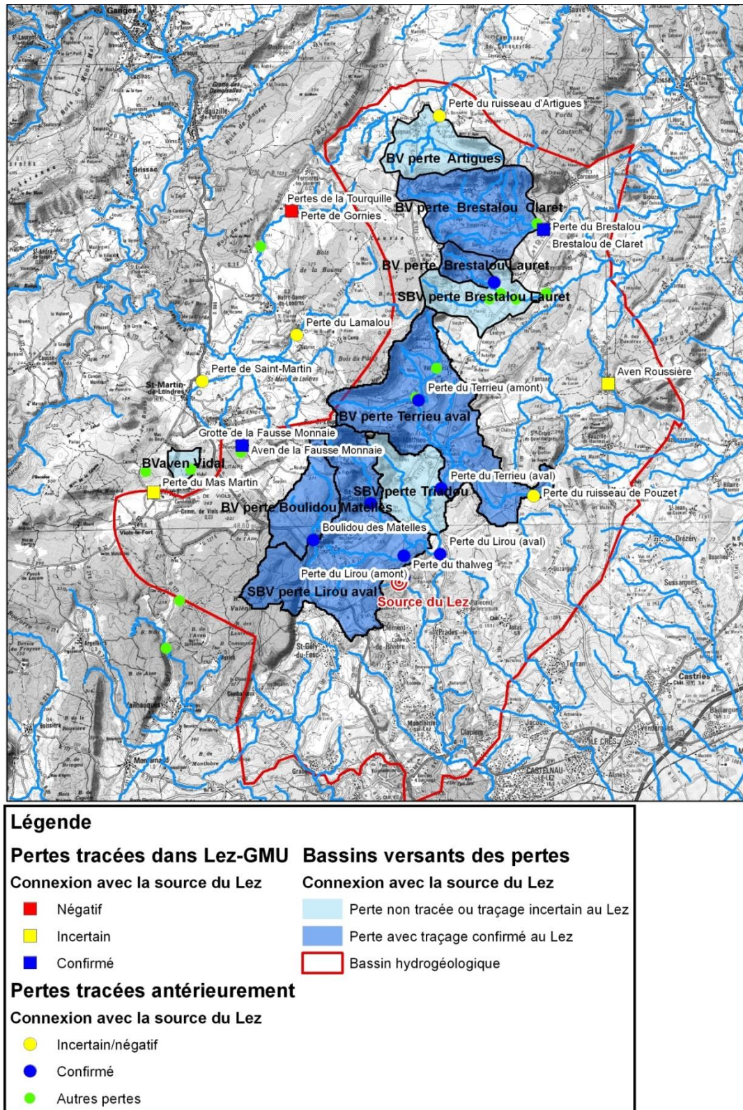
Illustration 11 : Carte des principales pertes, bassins des pertes et essais de traçages sur le bassin hydrogéologique en régime de pompage
