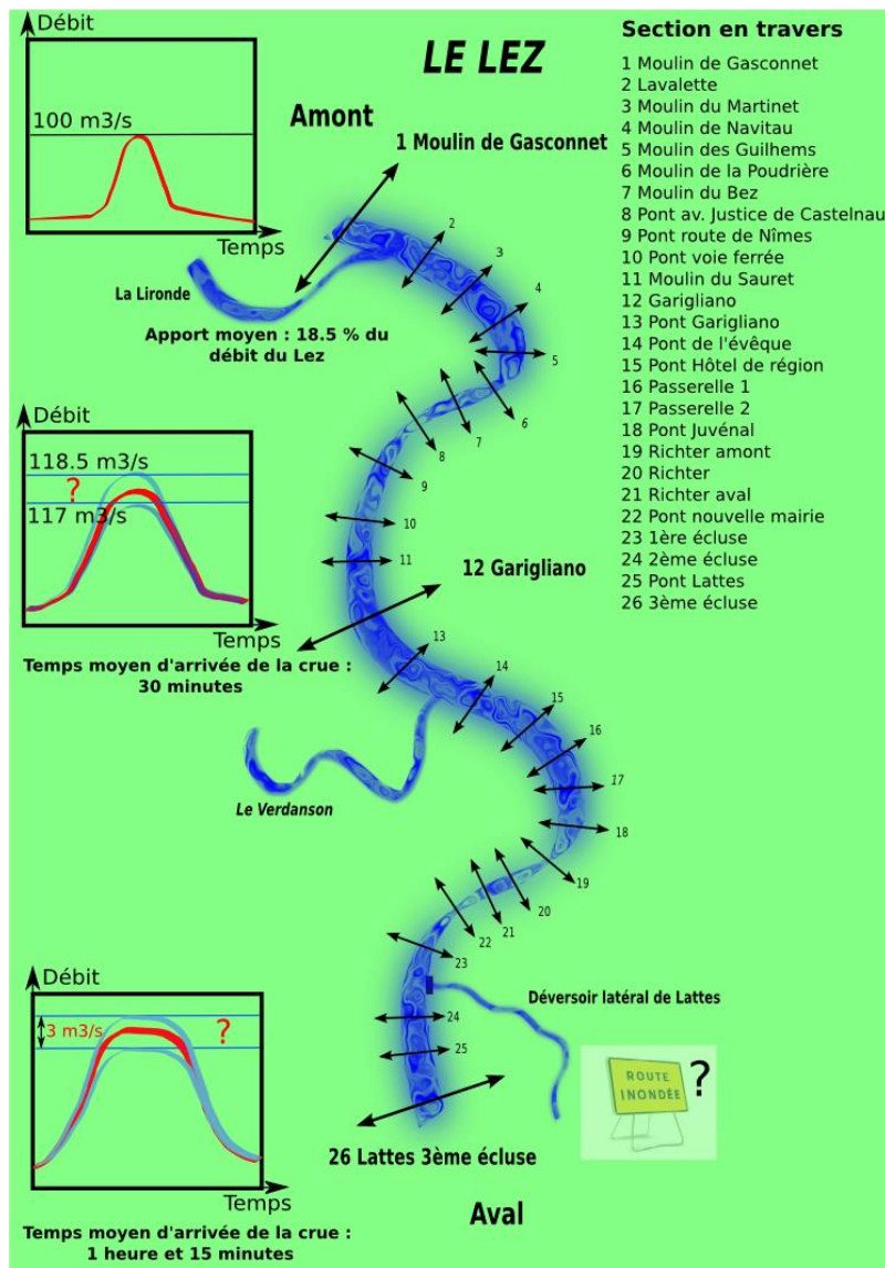
Illustration 64 : Zone du Lez modélisée sous SIC
