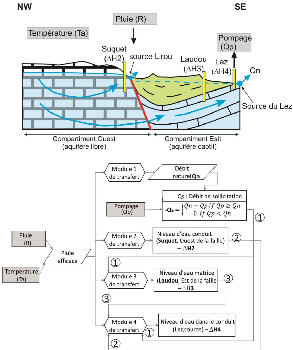
Illustration 20 : (a) coupe hydrogéologique de l'aquifère du Lez (b) schéma de modélisation inverse Tempo
