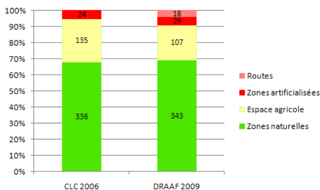
Illustration 53 : Occupation du sol : comparaison des statistiques exprimées en % et en km 2 pour les données CLC 2006 et DRAAF LR 2009 (agrégées respectivement en 3 et 4 classes)
