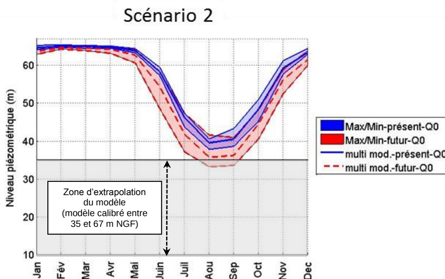
Illustration 73 : Comparaison des évolutions des moyennes mensuelles interannuelles de la piézométrie journalière. Traits pleins bleus : scénario de référence = climat présent [1971-2000] et prélèvement médian actuel [33 Mm 3 /an = Qp0]. Traits pointillés rouges : climat futur [2046-2065] et prélèvement médian actuel [33 Mm 3 /an = Qp0]. Les courbes enveloppes délimitent la gamme des moyennes interannuelles obtenues en considérant les 9 modèles climatiques. Les courbes au centre des courbes enveloppes caractérisent la moyenne multi-modèle. La limite 35 mNGF correspond au niveau d'eau minimum autorisé par le Déclaration d'Utilité Publique.
