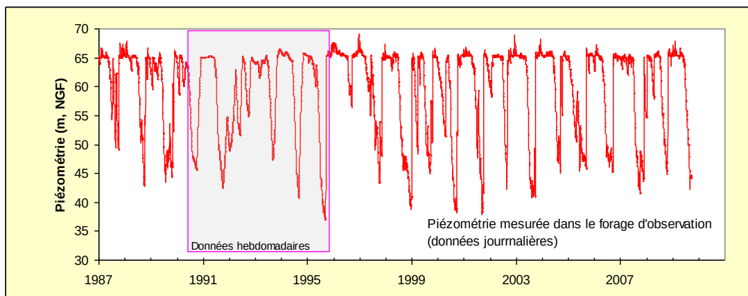
Illustration 33 : Graphique de la piézométrie mesurée dans le forage d'observation (données journalières) sur plus de vingt années, suite à la mise en exploitation par gestion active de la source du Lez, au niveau du captage
