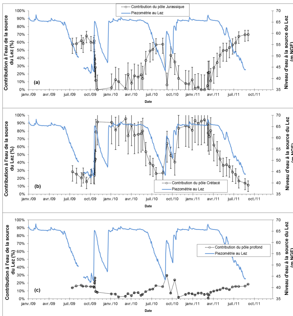
Illustration 38: Contributions relatives des trois pôles géochimiques aux eaux de la source du Lez sur la période d'étude (2009-2011)
