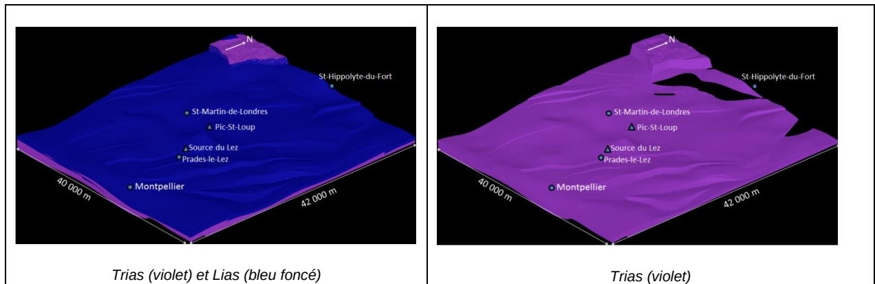
Illustration 4 : Modèles géologiques 3D de la zone d'étude avec empilement progressif des divers entités stratigraphiques
