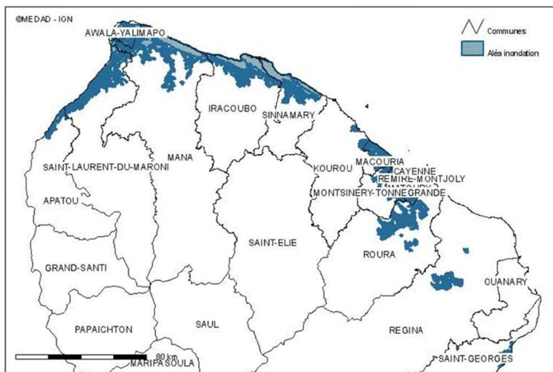
Figure 37 : Aléa Inondation pour la bande côtière (source DEAL Guyane)
