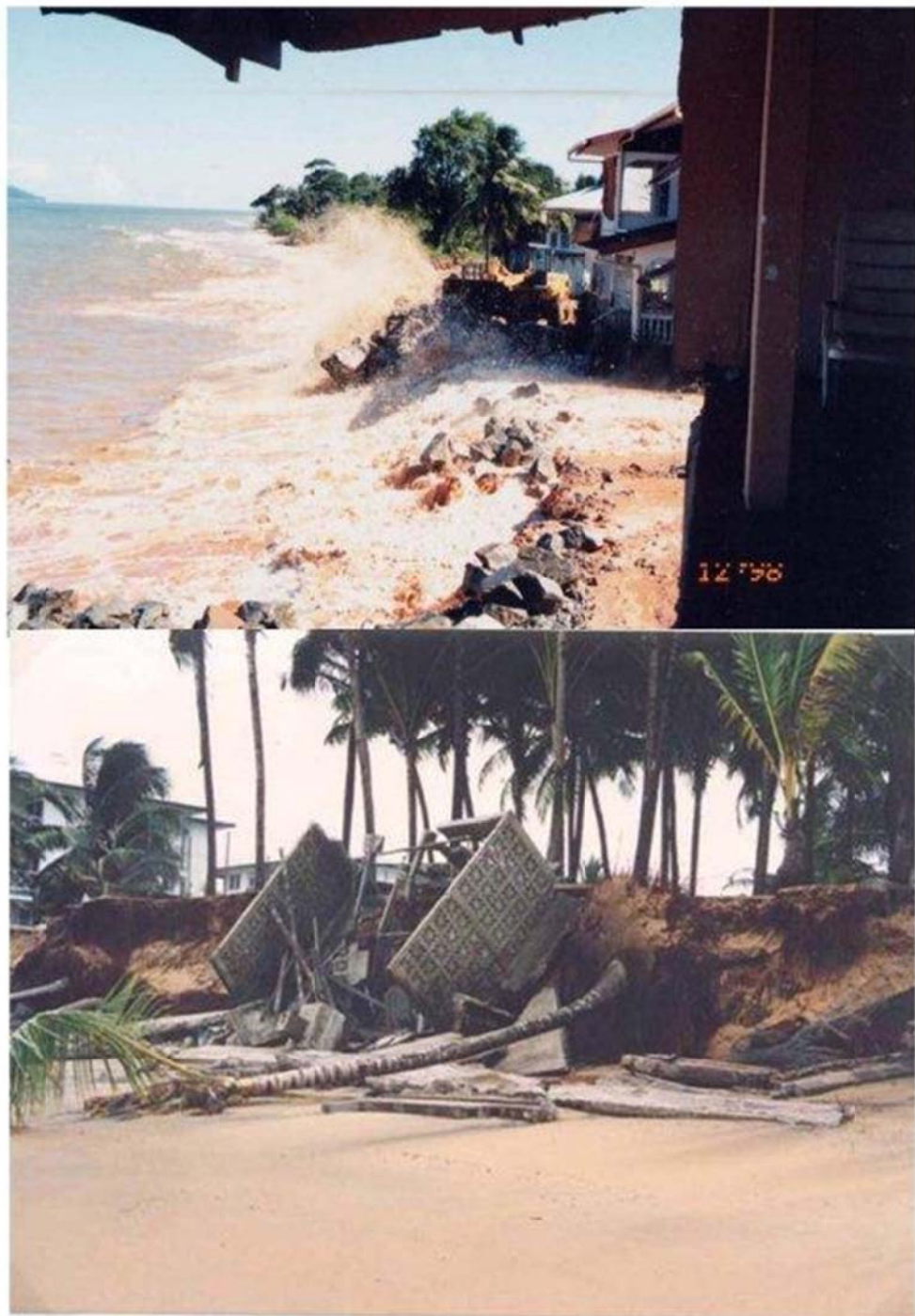
Figure 45 : Destruction de maisons sur les plages de Rémire Montjoly – fin des années '90 (source BRGM Guyane)
