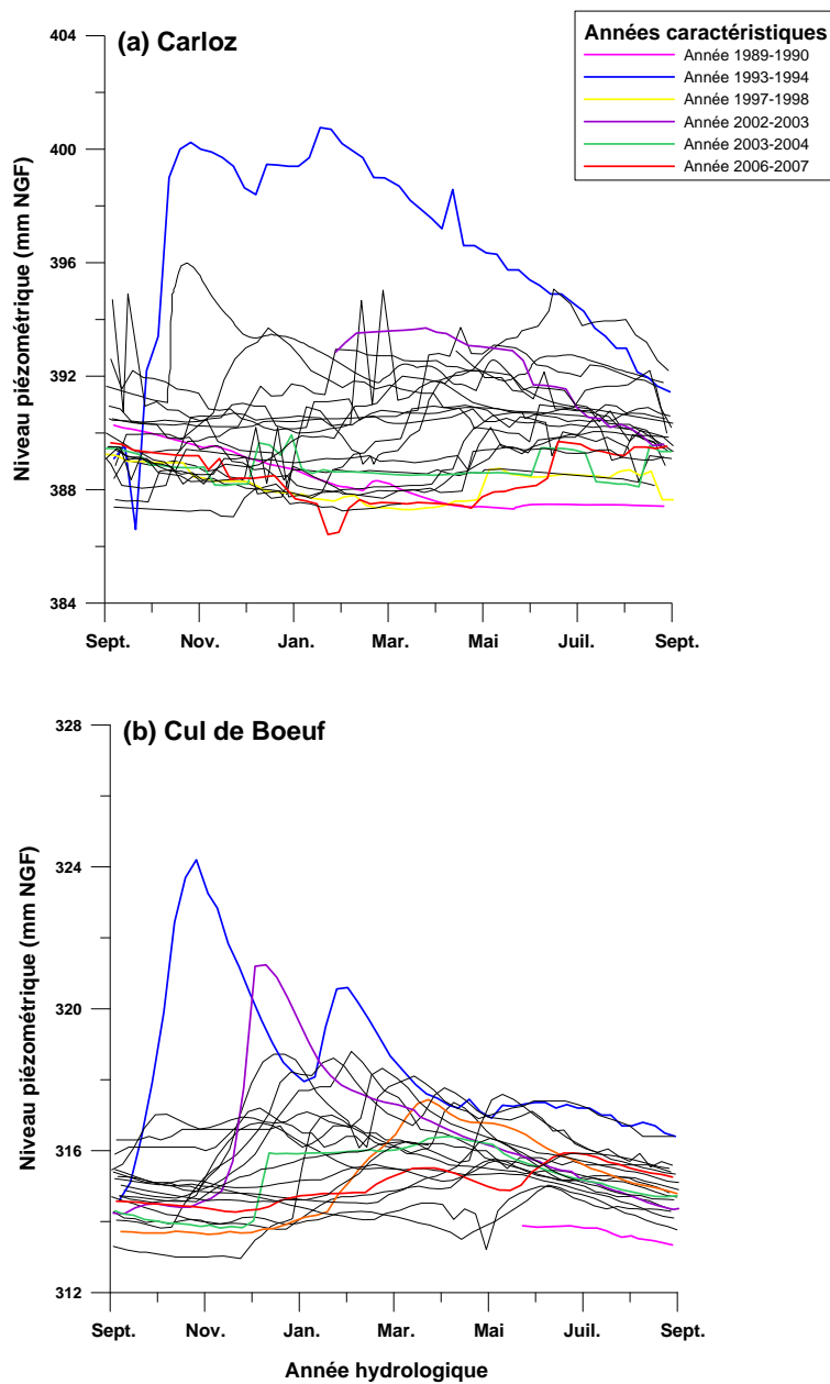
Illustration 73 : Variation de niveau piézométrique du forage Carloz (indice BSS : 07472X0012) (a) et du piézomètre de Cul de Boeuf (indice BSS : 07471X0005) (b) au cours d'une année hydrologique sur le sous-secteur Vésonne amont (Années hydrologiques 1987-1988 à 2009-2010 pour Carloz et 1989-1990 à 2009-2010 pour Cul de Boeuf)
