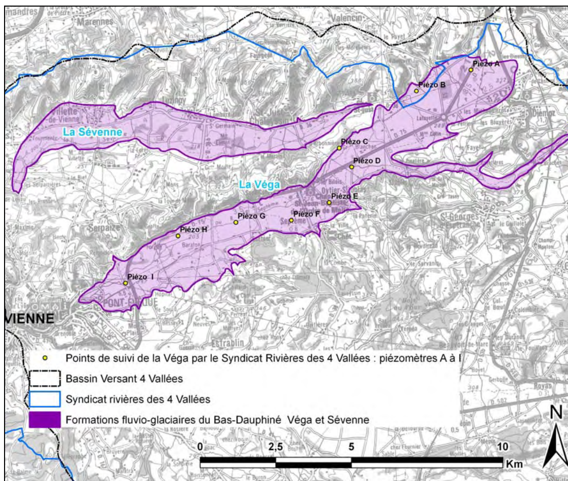
Illustration 76 : Localisation des piézomètres A à I sur la vallée de la Véga (suivi du Syndicat Rivières des 4 Vallées entre 2000 et 2010)
