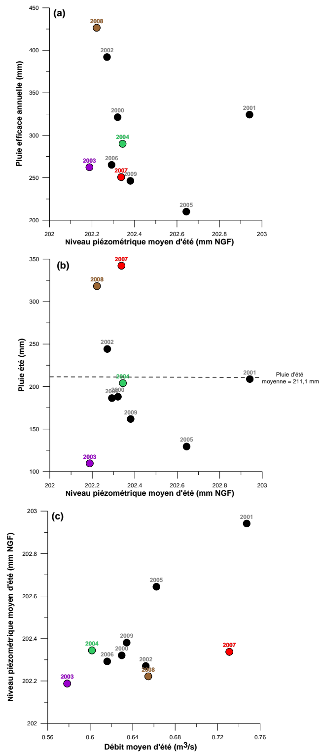
Illustration 85 : Niveau piézométrique moyen du piézo H pour l'été (mois de mai, juin, juillet, août) en fonction de la pluie efficace annuelle (a), de la pluie d'été (b) calculées pour la station météo de Bron et du débit moyen de la Vèga à Pont Evêque mesurés pour l'été (c).
