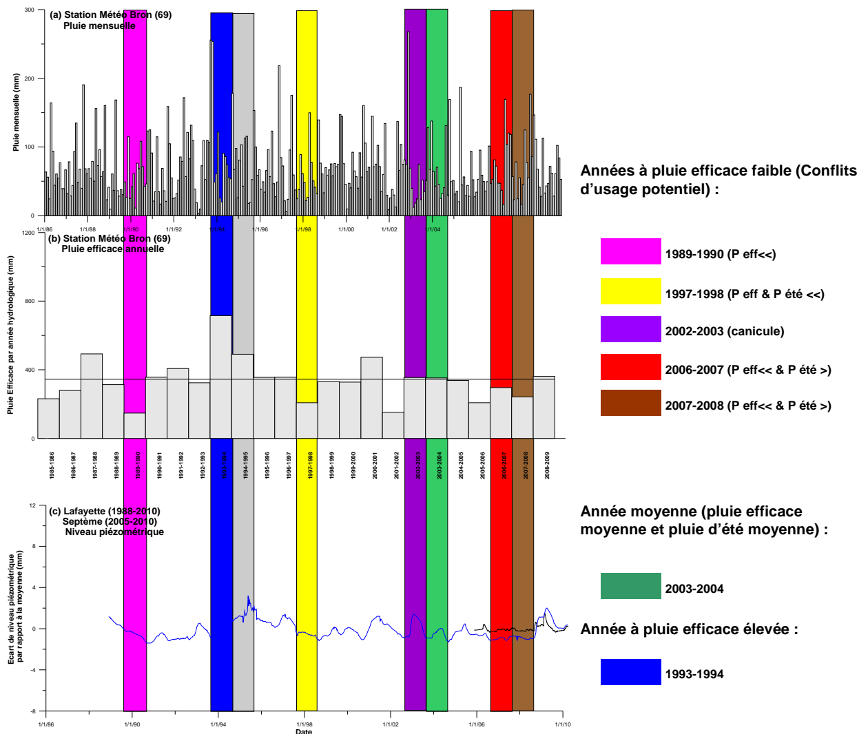
Illustration 79 : Variations temporelles de la pluie mensuelle (a), de la pluie efficace sur une année hydrologique (b), de l'écart de niveau piézométrique par rapport au niveau piézométrique moyen de la chronique du puits Lafayette et du piézomètre de Septème (c) sur le sous-secteur « Véga amont »
