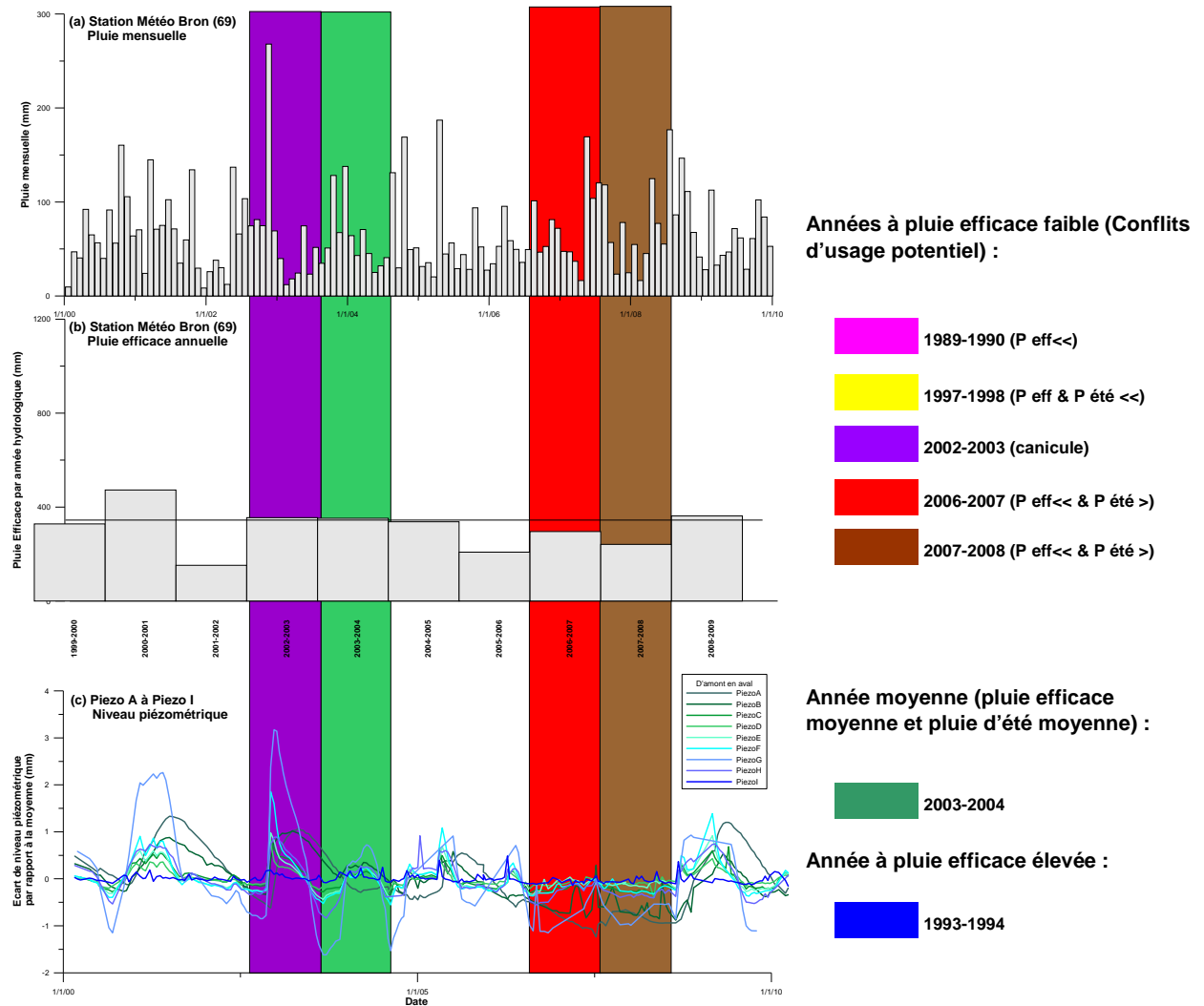
Illustration 81 : Variations temporelles de la pluie mensuelle (a), de la pluie efficace sur une année hydrologique (b), de l'écart de niveau piézométrique par rapport au niveau piézométrique moyen de la chronique des piézomètres A à I (c) sur les sous-secteurs « Véga amont » et « Véga aval »
