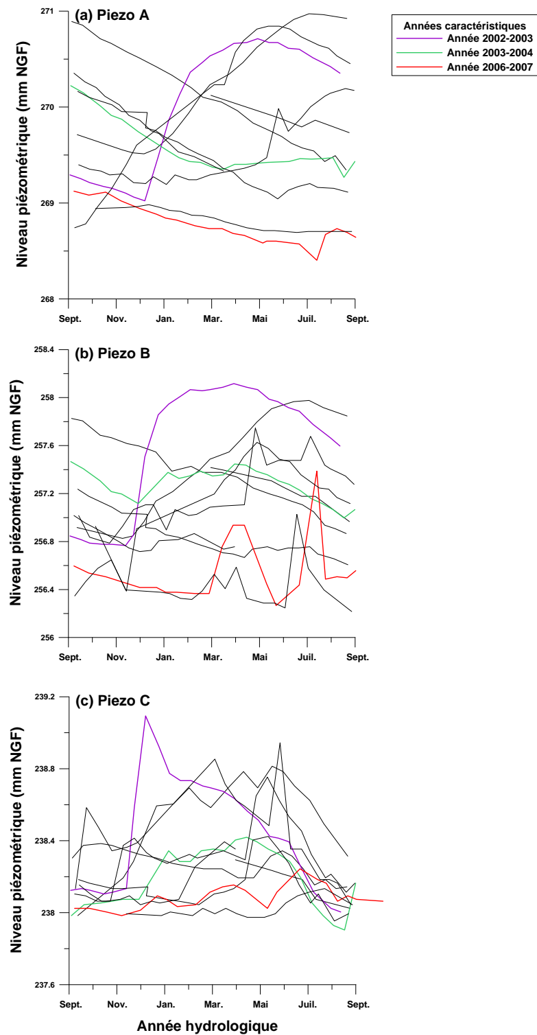
Illustration 70 : Variation des niveaux piézométriques des Piezo A (a), Piezo B (b) et Piezo C (c) au cours d'une année hydrologique sur le sous-secteur Véga amont (Années hydrologiques 1999-2000 à 2009-2010)
