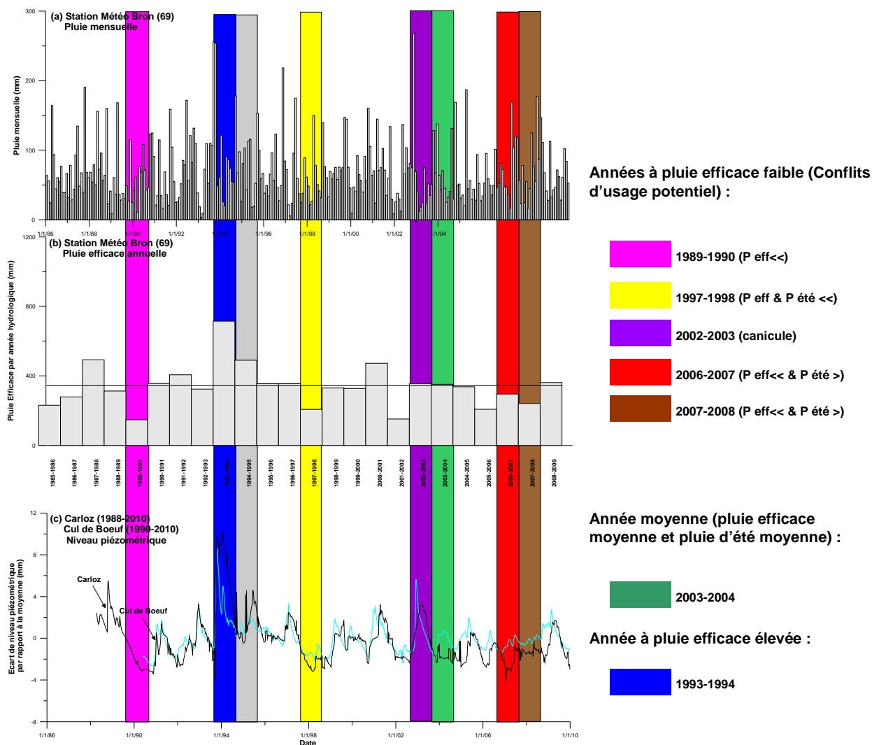
Illustration 80 : Variations temporelles de la pluie mensuelle (a), de la pluie efficace sur une année hydrologique (b), de l'écart de niveau piézométrique par rapport au niveau piézométrique moyen de la chronique du forage de Carloz et du piézomètre de Cul de Bœuf (c) sur le sous-secteur « Vésonne amont »
