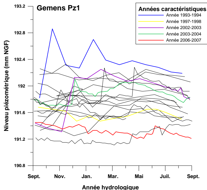
Illustration 75 : Variation de niveau piézométrique du piézomètre 1 de Gemens (indice BSS : 07463X0008) au cours d'une année hydrologique sur le sous-secteur Gère amont (Années hydrologiques 1991-1992 à 2009-2010)
