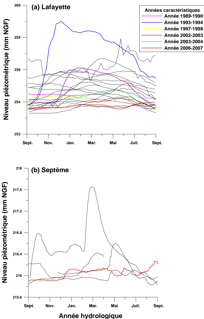
Illustration 69 : Variations des niveaux piézométriques du puits Lafayette (indice BSS : 07235X0011) (a) et du piézomètre de Septème (indice BSS : 07228X0017) (b) au cours d'une année hydrologique sur le sous-secteur Vêga amont (Années hydrologiques 1986-1987 à 2009-2010 pour Lafayette et 2005-2006 à 2009-2010 pour Septème)
