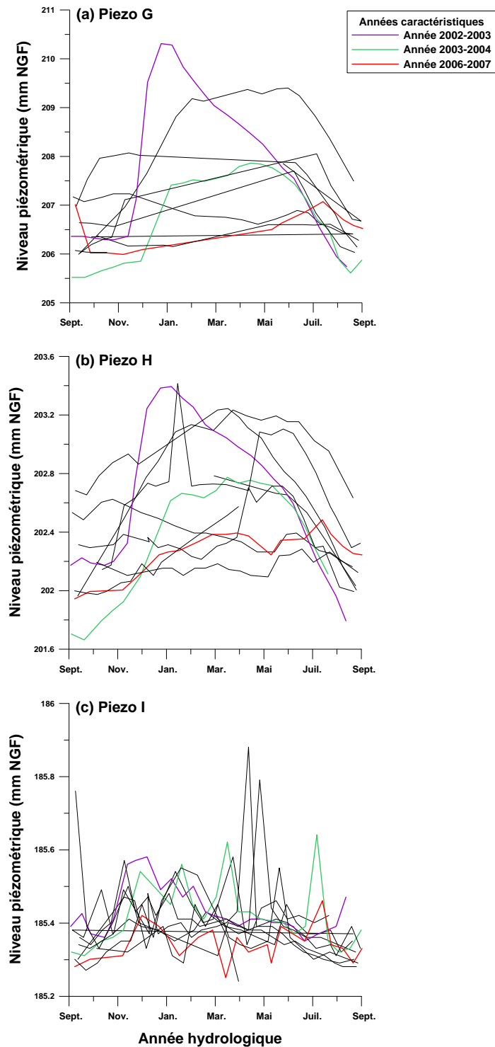
Illustration 72 : Variation de niveau piézométrique du Piezo G (a) sur le sous-secteur Véga amont et du Piezo H (b) et Piezo I (c) au cours d'une année hydrologique sur le sous-secteur Véga aval (Années hydrologiques 1999-2000 à 2009-2010)
