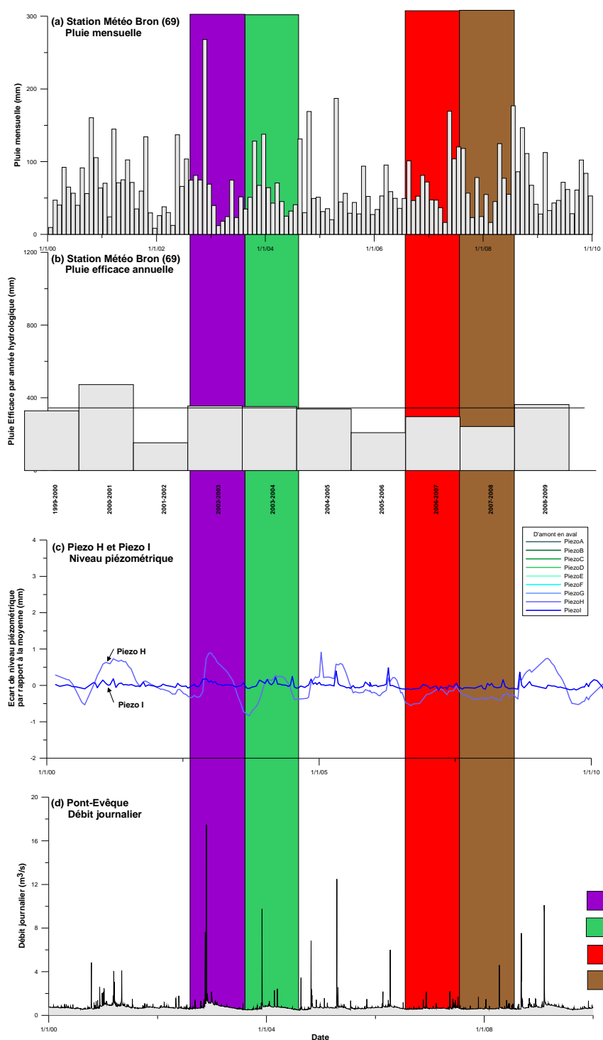
Illustration 83 : Variations temporelles de la pluie mensuelle (a), de la pluie efficace sur une année hydrologique (b), de l'écart de niveau piézométrique par rapport au niveau piézométrique moyen de la chronique de Piezo H et Piezo I (c) et du débit journalier de la Véga (d) sur le sous-secteur Véga aval.
