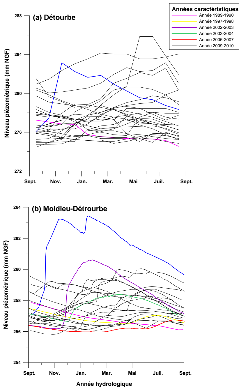
Illustration 74 : Variation de niveau pi  zom  trique du puits de D  tourbe (indice BSS : 07471X0001) (a) et du pi  zom  tre de Moidieu-D  tourbe (indice BSS : 07464X0005) (b) au cours d'une ann  e hydrologique sur le sous-secteur V  sonne aval (Ann  es hydrologiques 1965-1966    1997-1998 pour D  tourbe et 1986-1987    2009-2010 pour Moidieu-D  tourbe)
