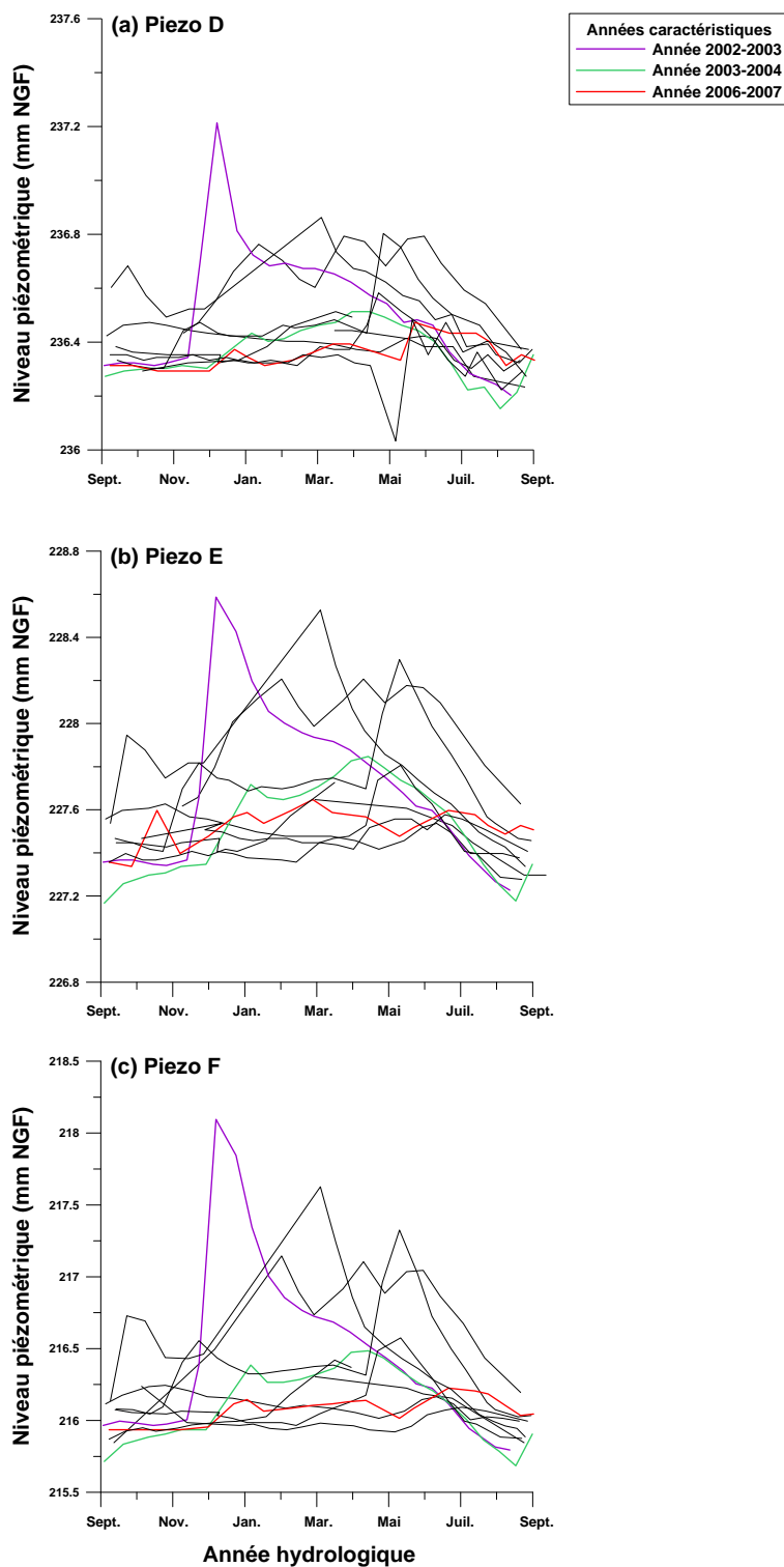
Illustration 71 : Variation de niveaux piézométriques des Piezo D (a), Piezo E (b) et Piezo F (c) au cours d'une année hydrologique sur le sous-secteur Véga amont (Années hydrologiques 1999-2000 à 2009-2010)
