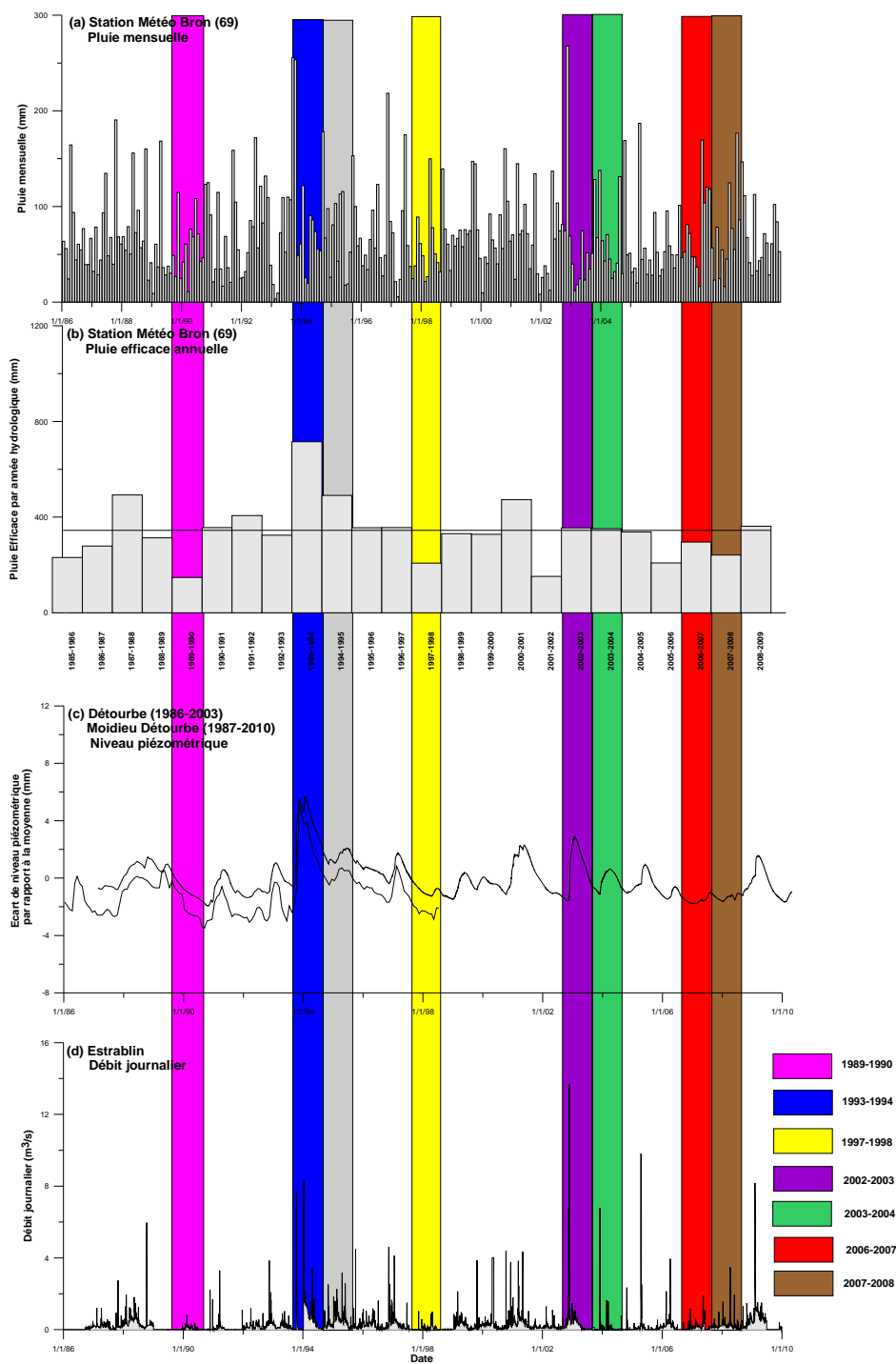
Illustration 84 : Variations temporelles de la pluie mensuelle (a), de la pluie efficace sur une année hydrologique (b), de l'écart de niveau piézométrique par rapport au niveau piézométrique moyen de la chronique de Détourbe et Moidieu-Détourbe (c) et du débit journalier de la Vésonne (d) sur le sous-secteur Vésonne aval.
