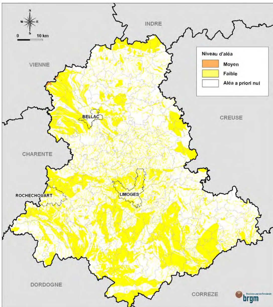
Illustration 1 - Carte départementale de l'aléa retrait-gonflement des sols argileux ou marneux de la Haute-Vienne (carte extraite du rapport BRGM/RP-58290-FR, juin 2010)
