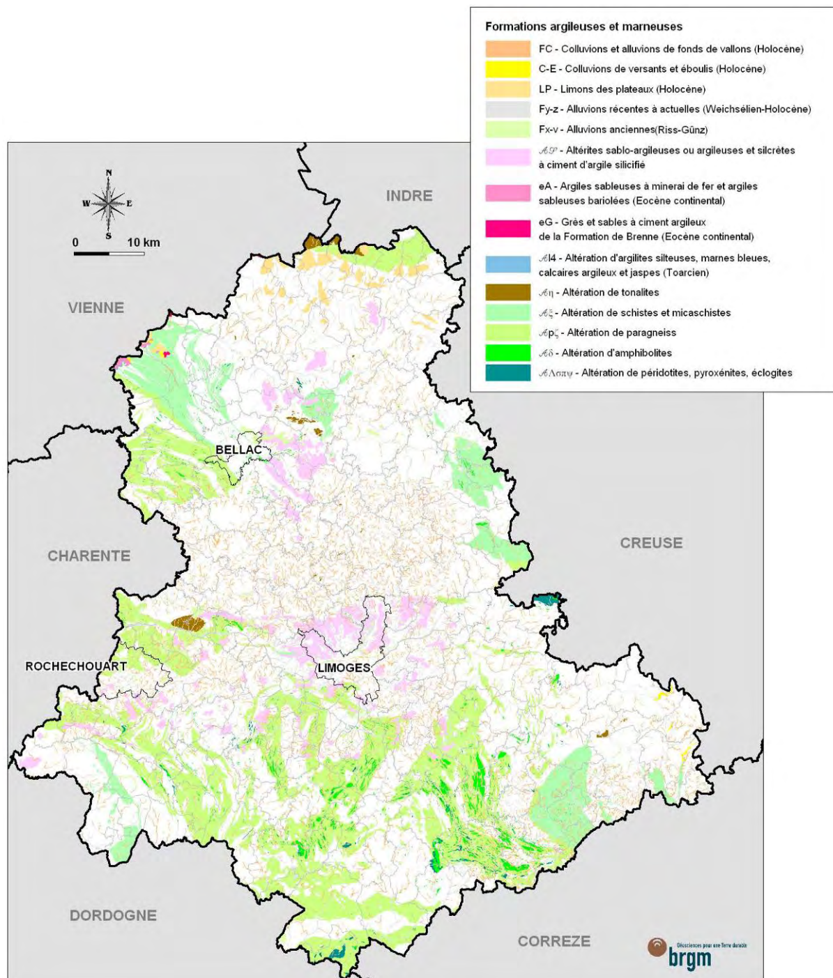
Illustration 1 : Carte synthétique des formations argileuses et marneuses de la Haute-Vienne (carte extraite du rapport BRGM/RP-58290-FR, juin 2010)
