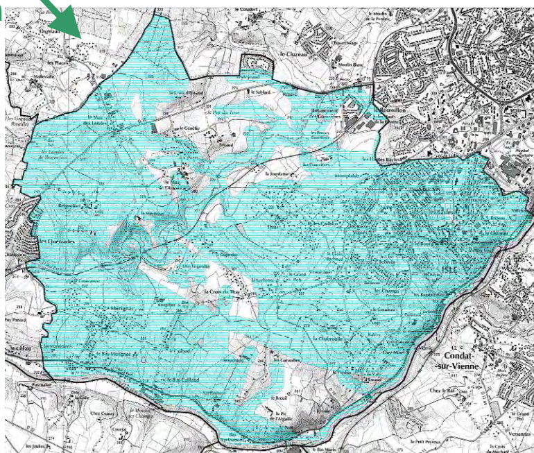
Illustration 2 - Transcription, pour la commune d'Isle, de la carte d'aléa en proposition de plan de zonage réglementaire
