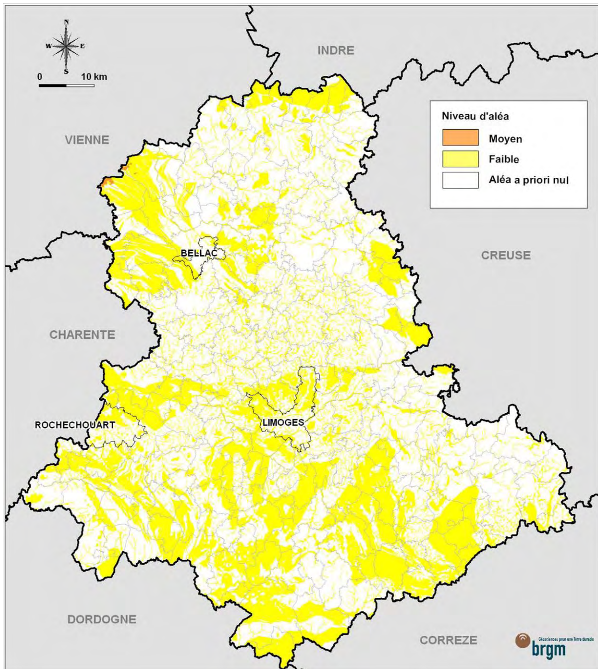
Illustration 3 – Carte départementale de l'aléa retrait-gonflement des sols argileux de la Haute-Vienne (carte extraite du rapport BRGM/RP-58290-FR, juin 2010)
