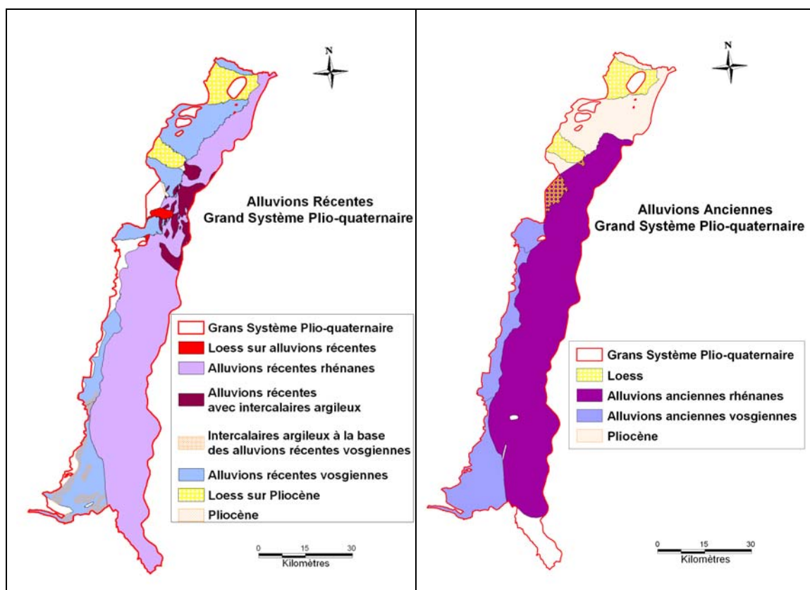
Illustration 15 – Découpage du système plio –quaternaire de la plaine d'Alsace
