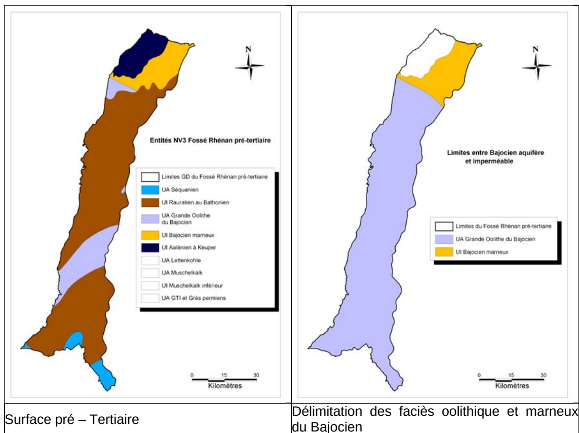
Illustration 19 – Découpage de la plaine d'Alsace (unités pré-Tertiaire)
