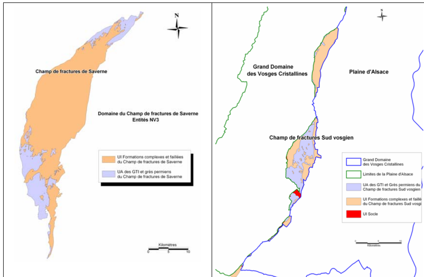
Illustration 25 - Découpage des zones de fractures
