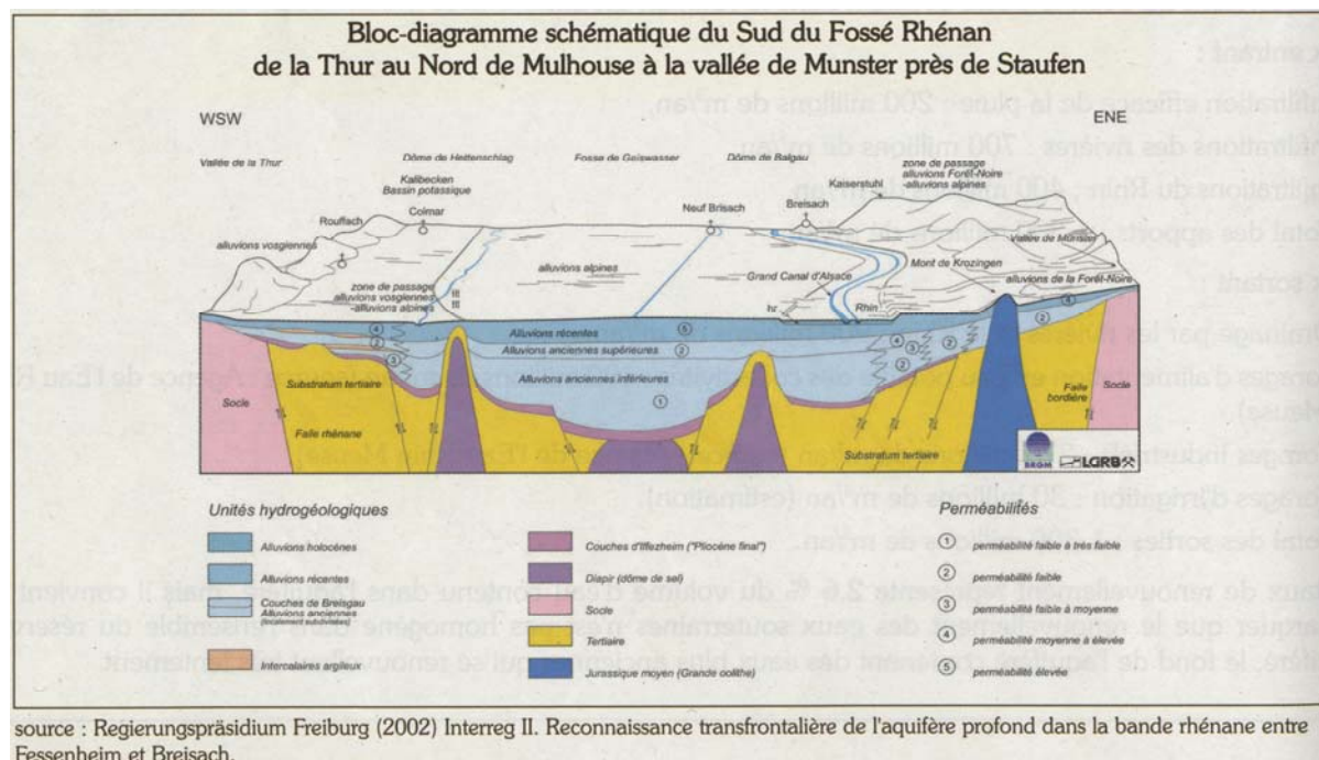
Illustration 14 – Coupe schématique du Sud du Fossé Rhénan
