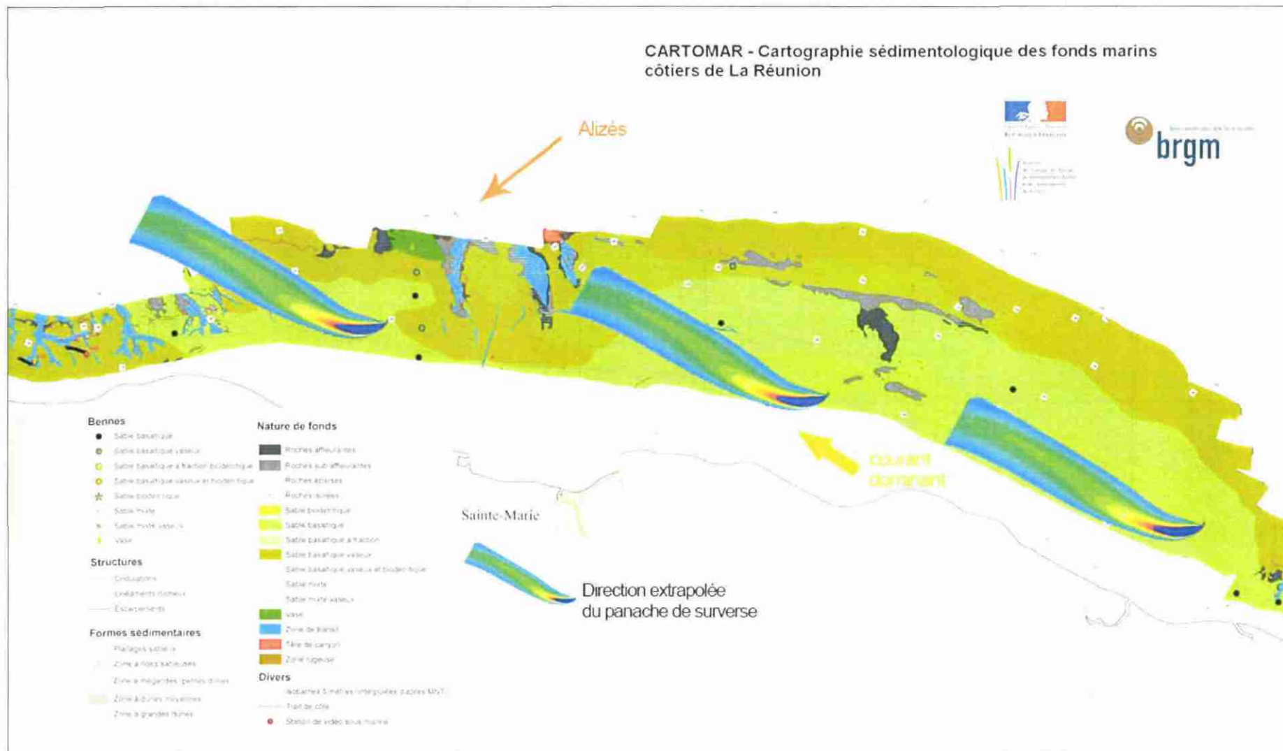
Figure 27 : Orientations possibles du panache de surverse dans l'hypothèse d'opérations d'extraction dans le secteur 2
