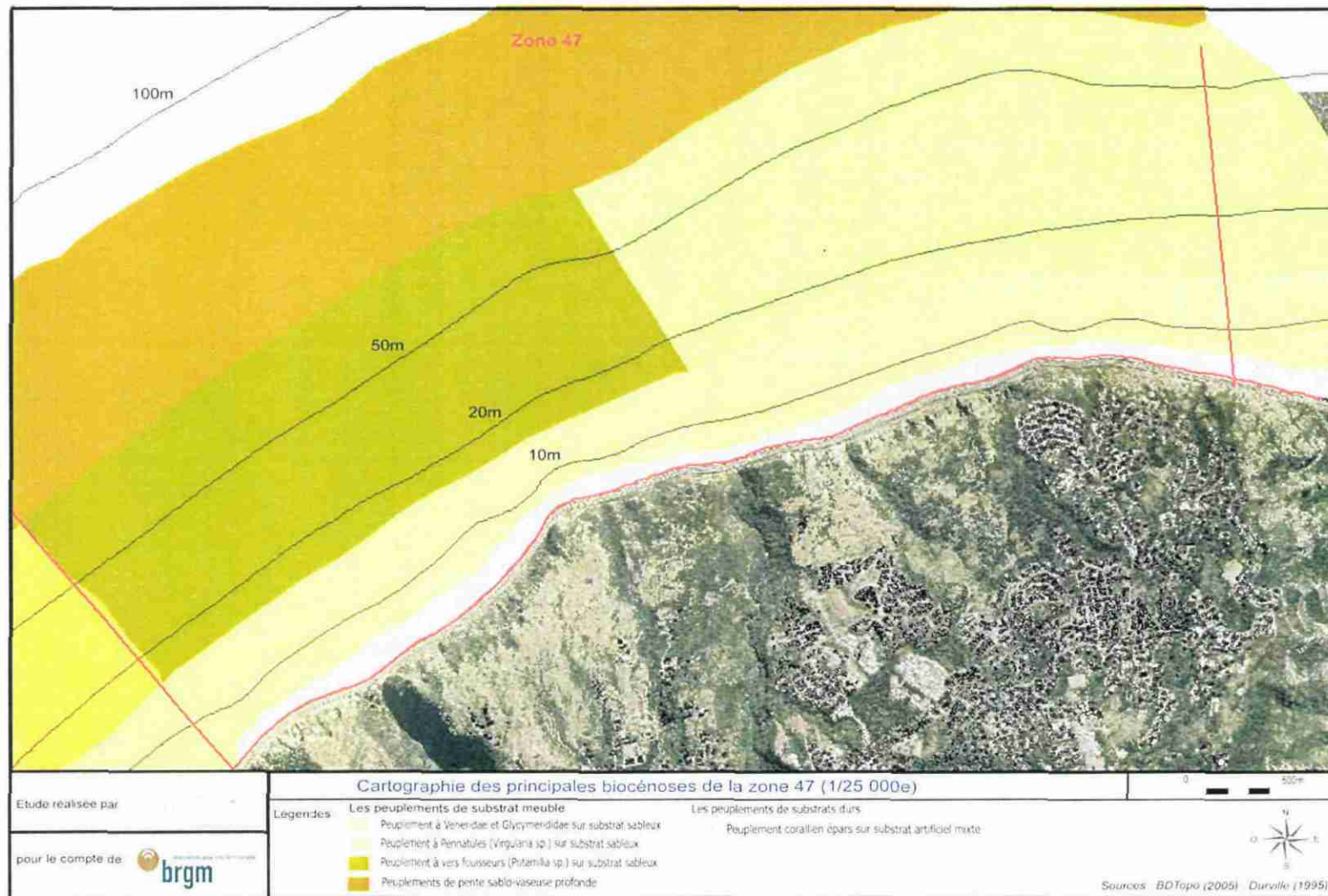
Figure 17 : Cartographie des principales biocénoses de l'unité géomorphologique 47
