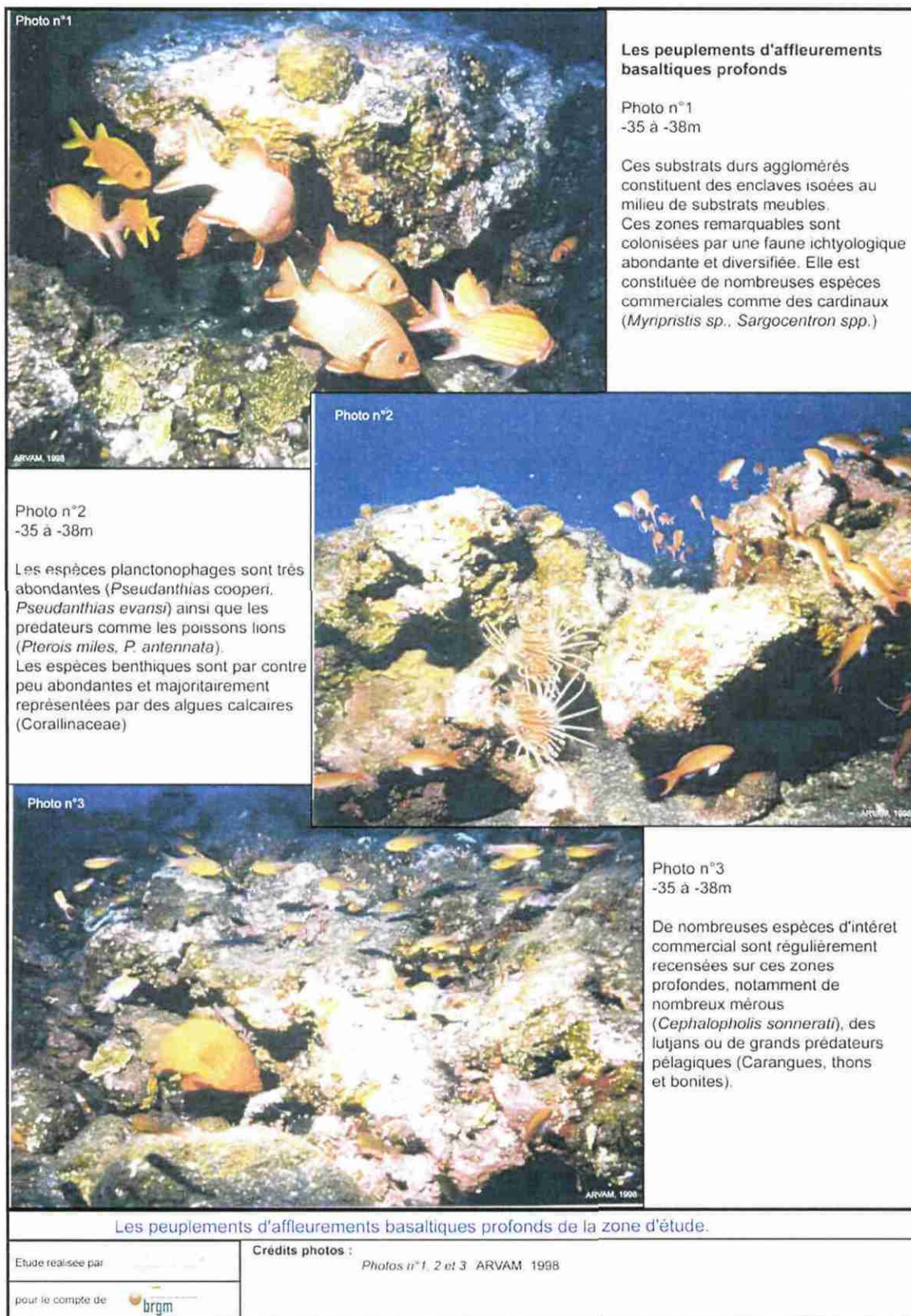
Figure 14 : Les peuplements d'affleurements basaltiques profonds (-35 à -60m)
