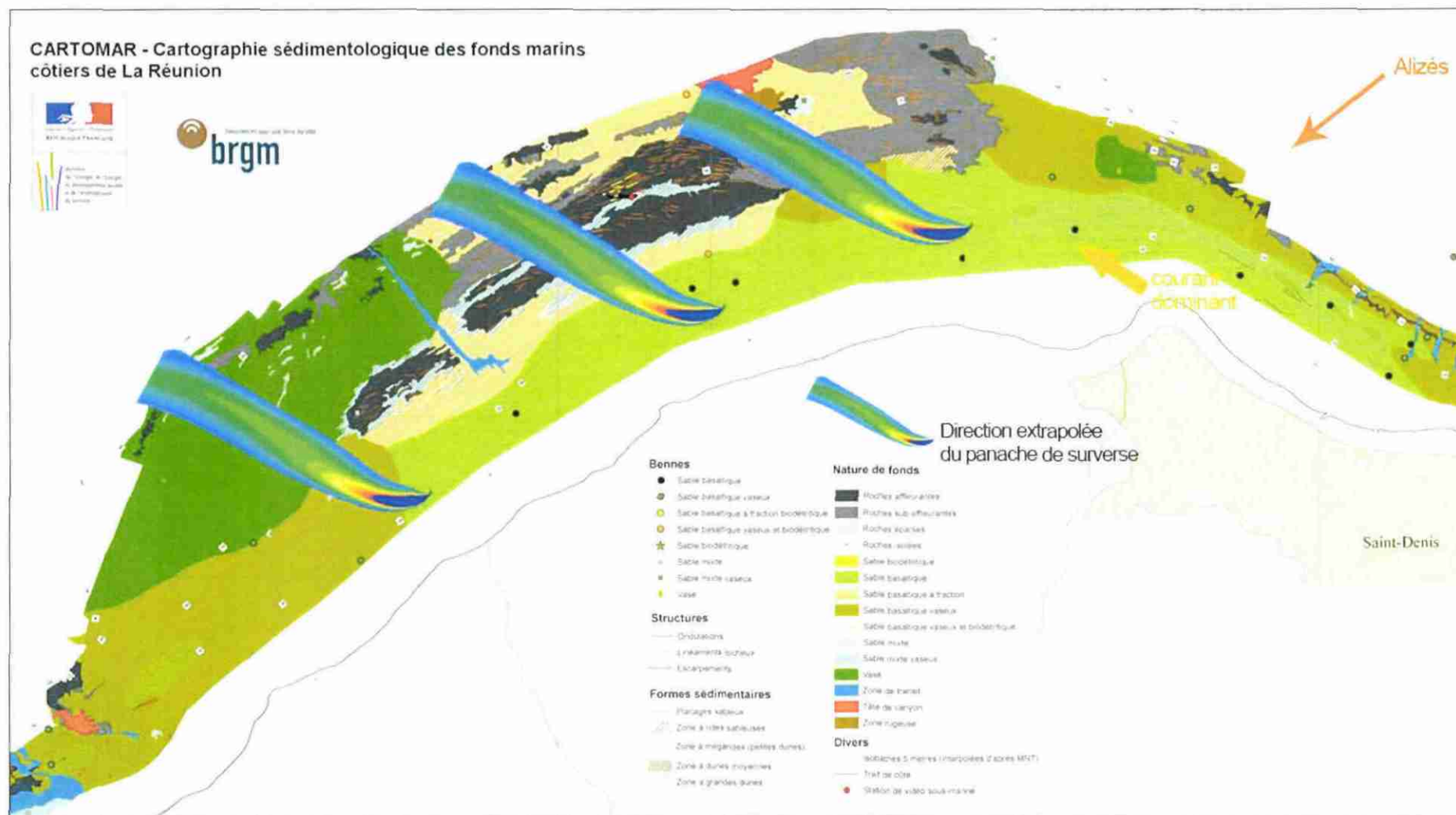
Figure 26 : Orientations possibles du panache de surverse dans l'hypothèse d'opérations d'extraction dans le secteur 1
