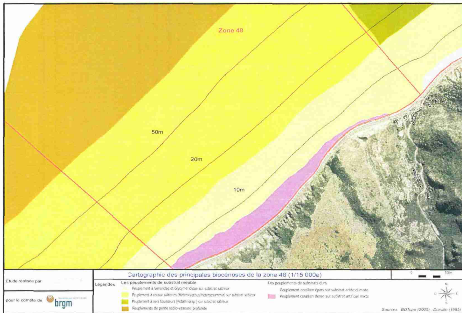
Figure 19 : Cartographie des principales biocénoses de l'unité géomorphologique 48
