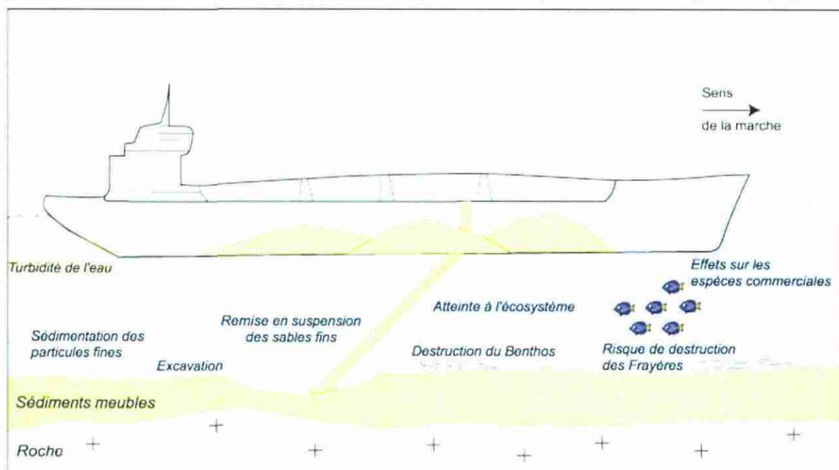
Figure 24 : Illustration des différents impacts potentiels des travaux d'extraction de sables (source IFREMER)
