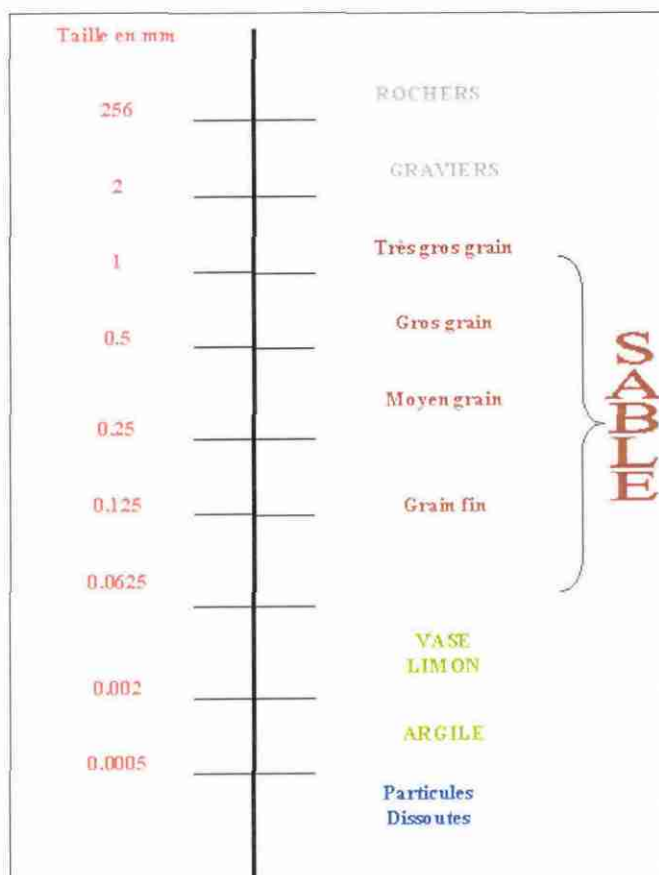
Figure 10 : Echelle de Wentworth
