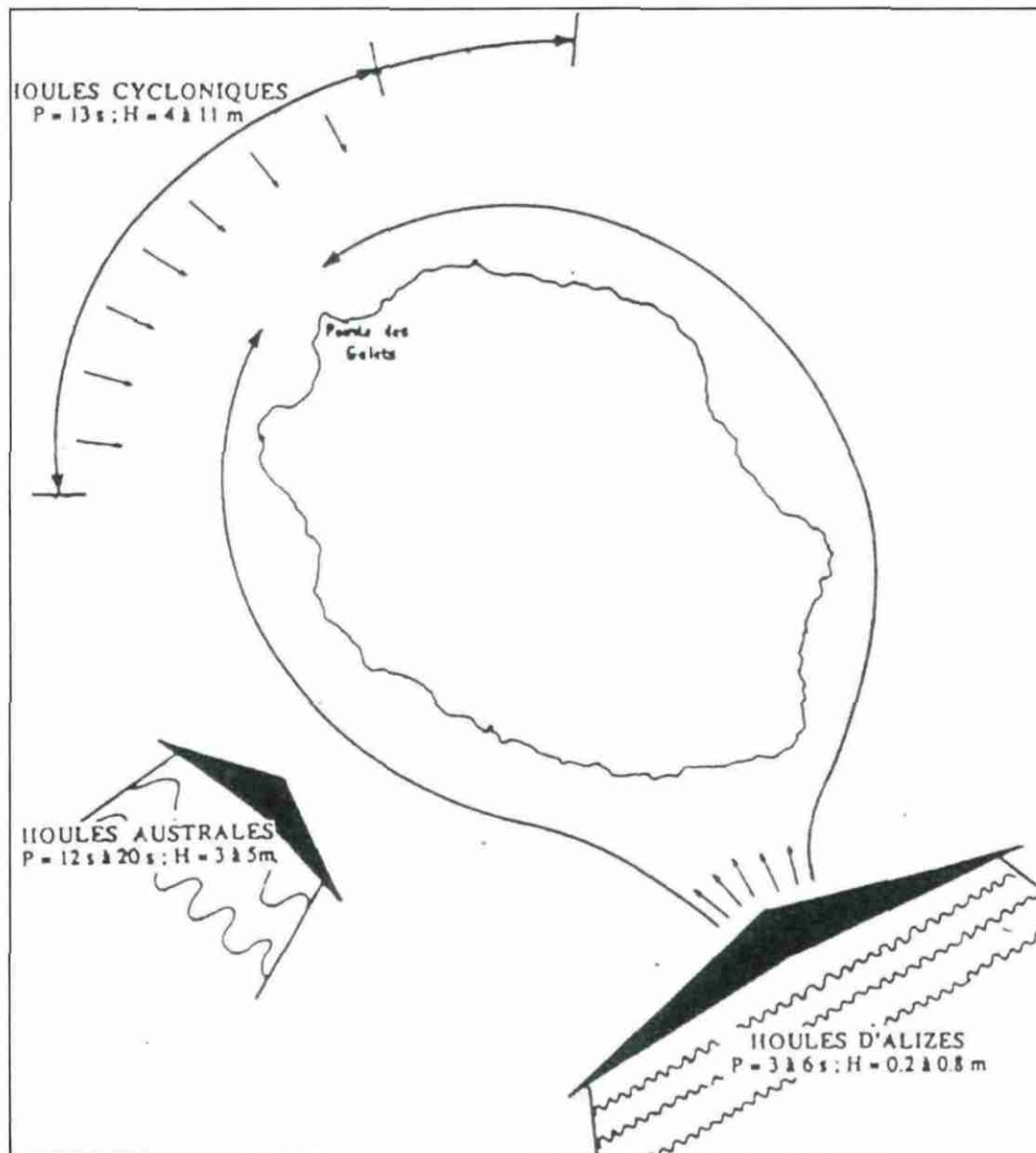
Figure 6 : Les différents régimes de houle à La Réunion (Gabrié, 1982)
