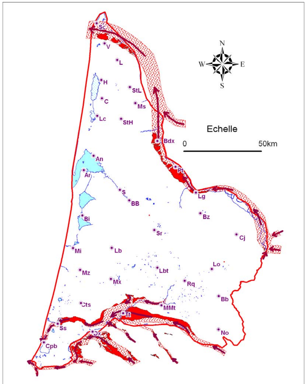
Figure 14 : Extension des alluvions du Mindel et affleurements
