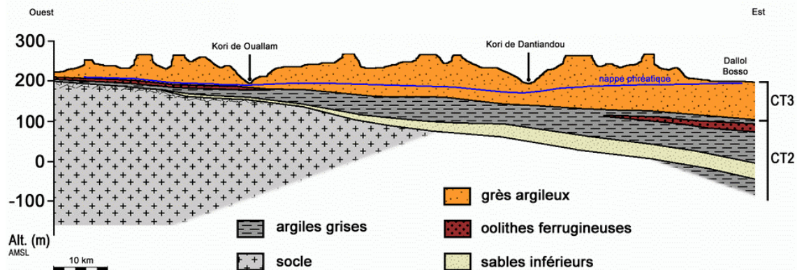
Figure 1 – Coupe hydrogéologique schématique de la zone d'étude (Massuel, 2005)
