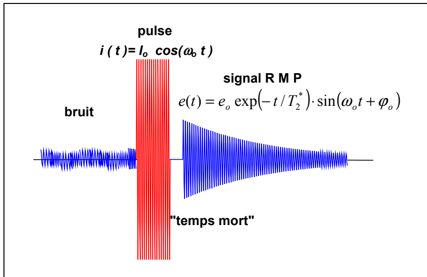
Figure 5 – Schéma en fonction du temps d'une séquence émission/réception
