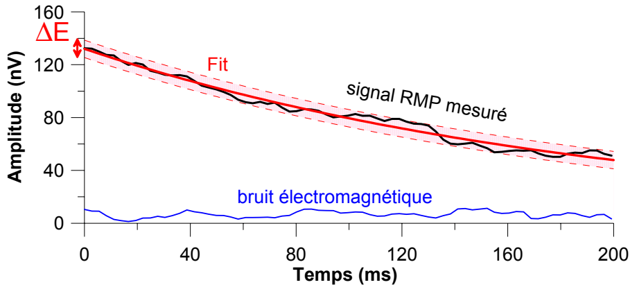
Figure 16 – Incertitude sur la mesure du signal RMP liée au bruit électromagnétique
