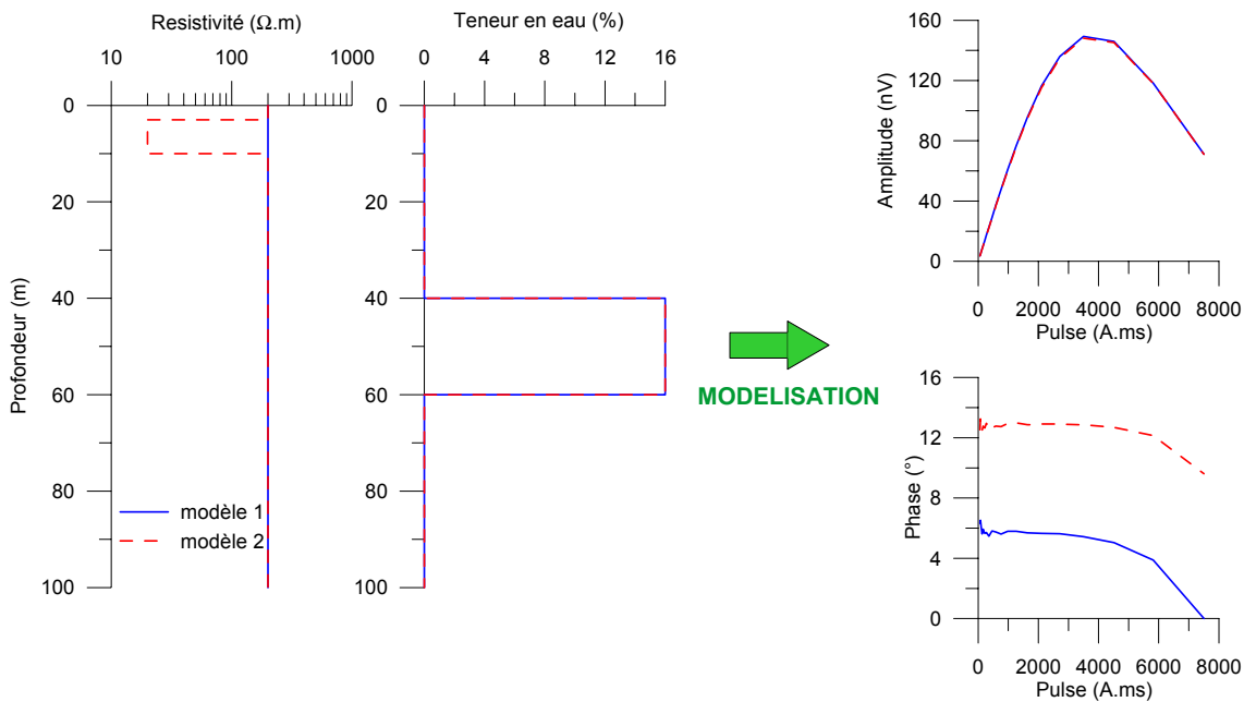
Figure 21 – Effet d'un niveau conducteur superficiel sur le signal RMP. A gauche : paramètres initiaux : résistivité et teneur en eau. A droite : réponse RMP
