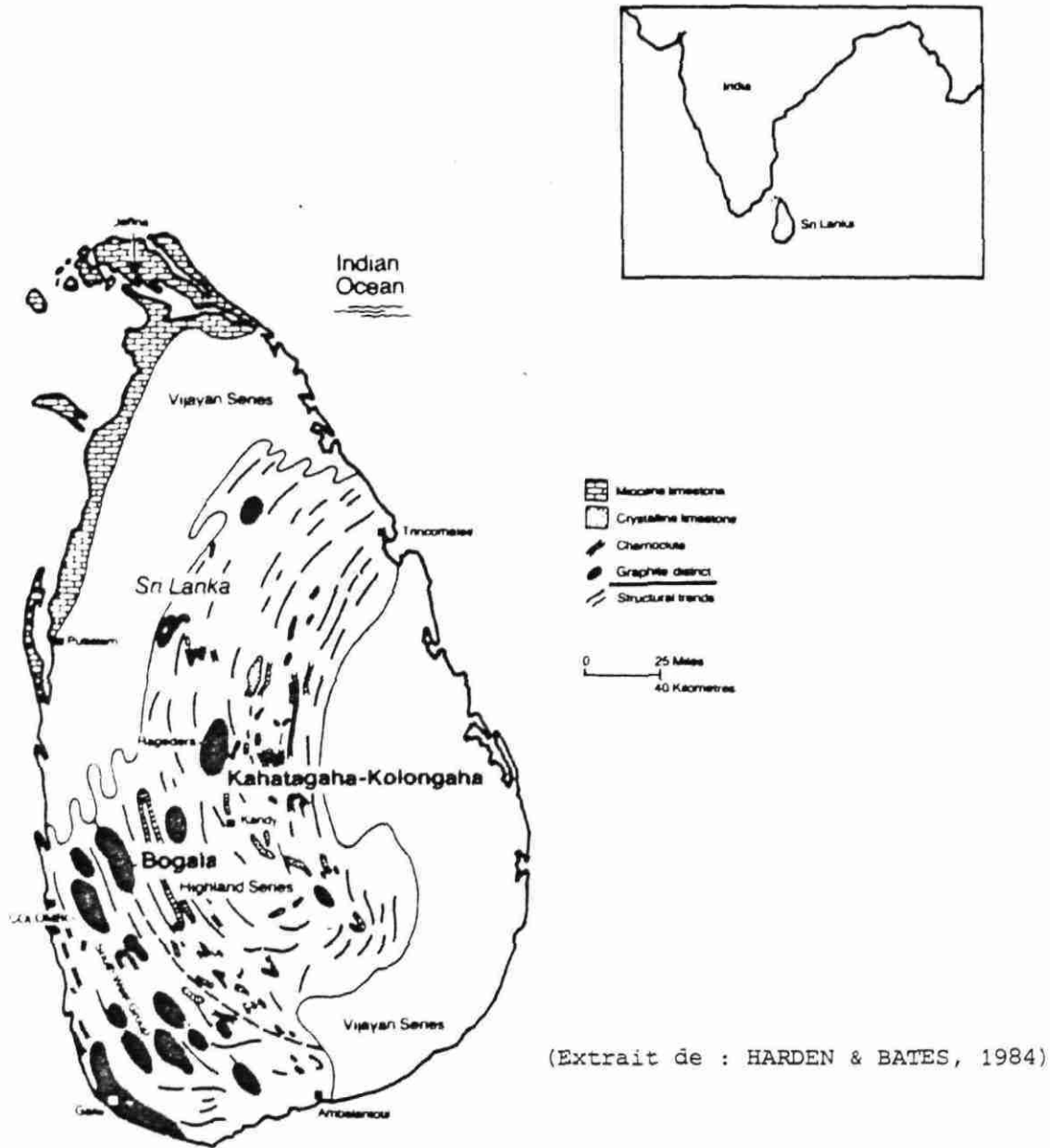
Fig. 4 : Localisation des gisements de graphite de Sri-Lanka
